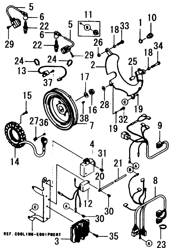
FIG. 6 ELECTRIC-EQUIPMENT
