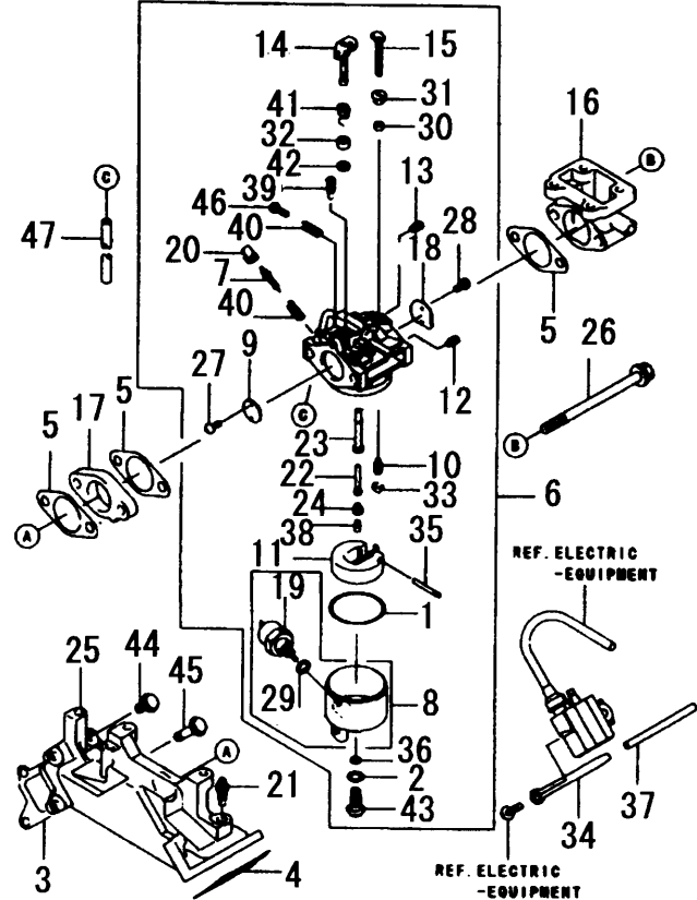
FIG. 8 CARBURETOR
