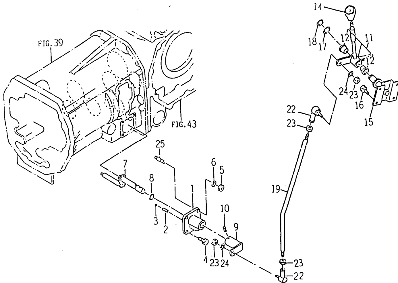
FIG : 50. 체인지 관계(CHANGE)
