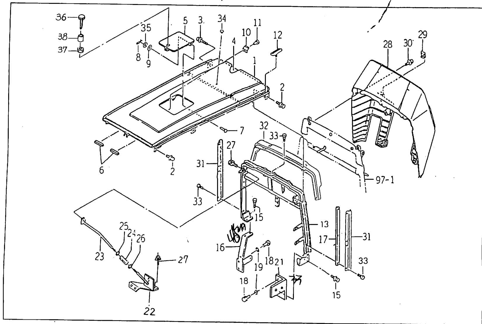
FIG : 90. 본넷 관계(1) (BONNET 1)
