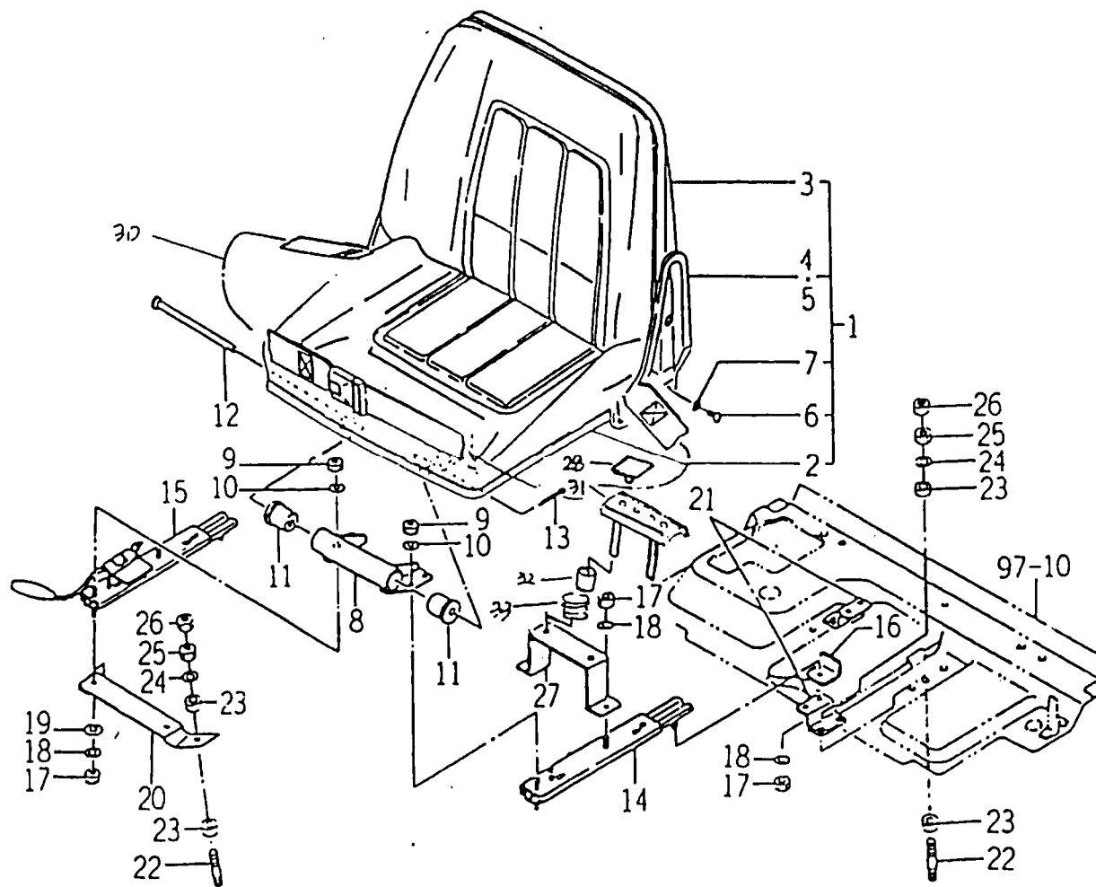
FIG : 95. 씨트 관계(SEAT)
