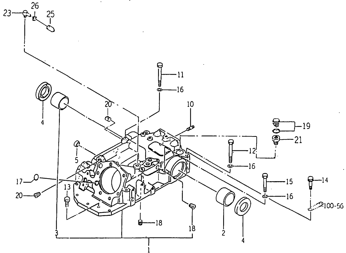
FIG : 69. 실린더 케이스 관제(CYLINDER CASE)
