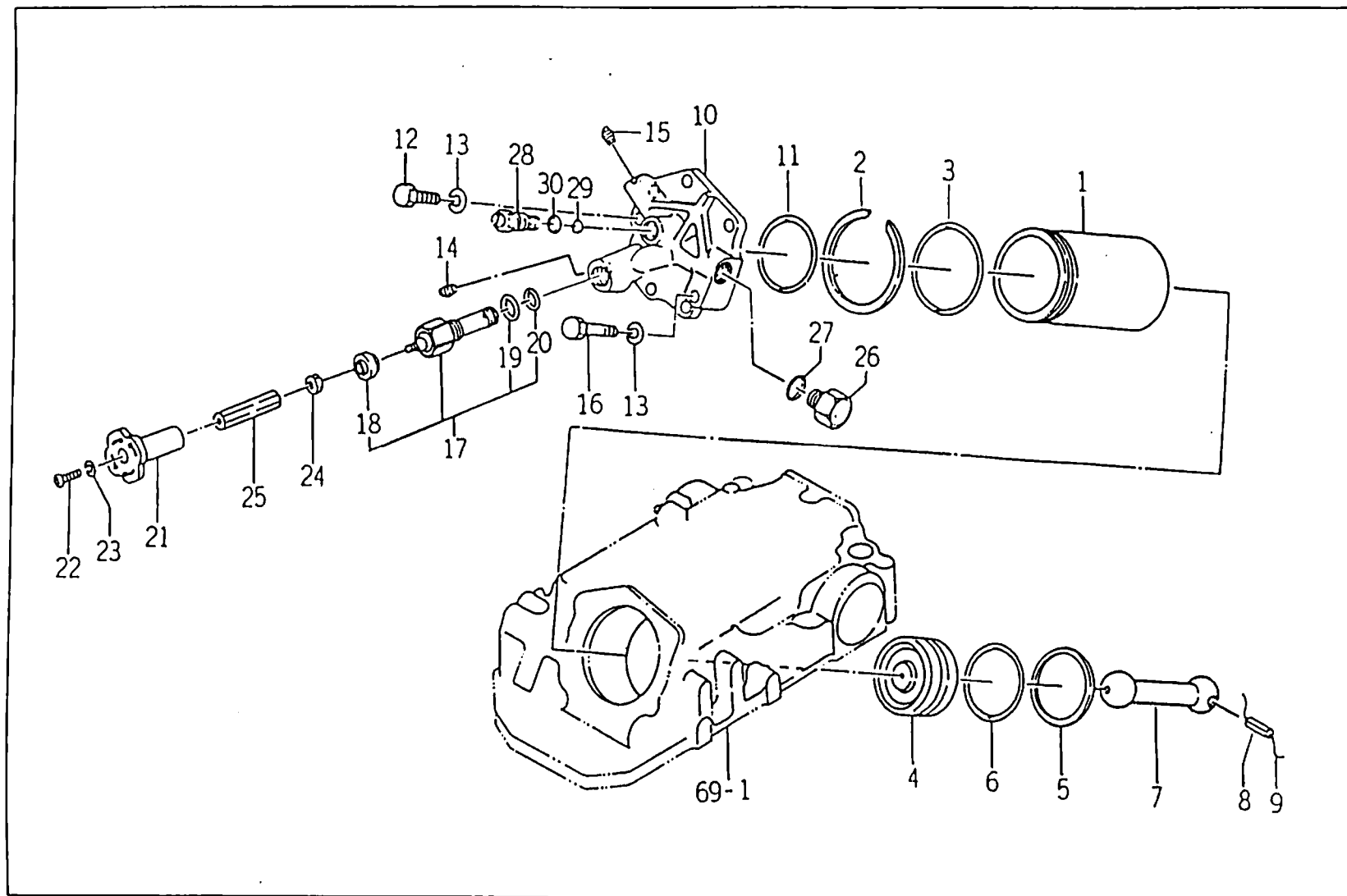
FIG : 73. 실린더 관개(CYLINDER)
