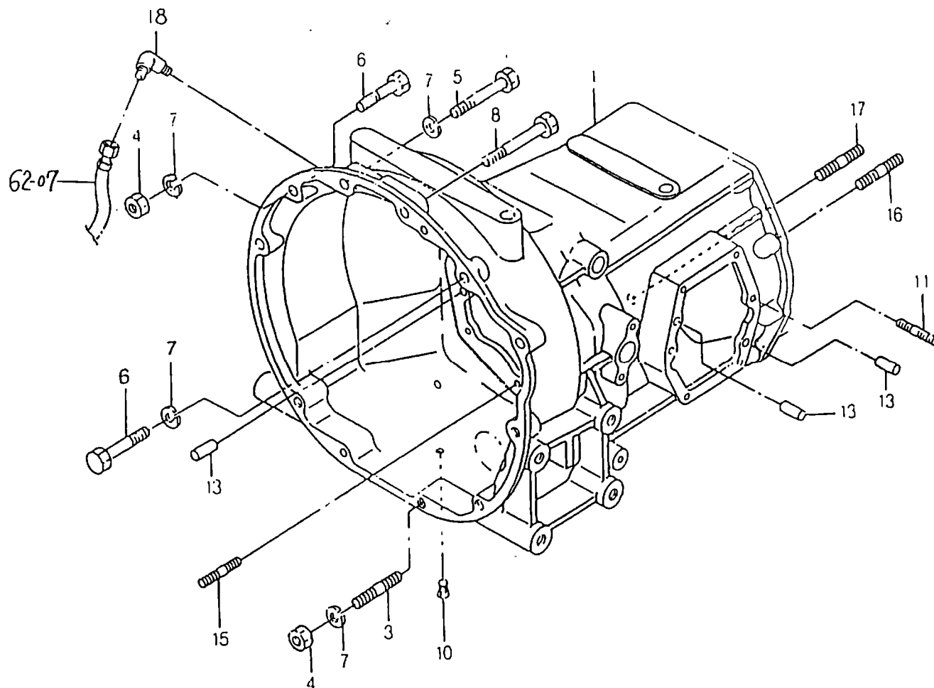
FIG : 31. 프론트 미션케이스 관계(FRONT MISSION CASE)
