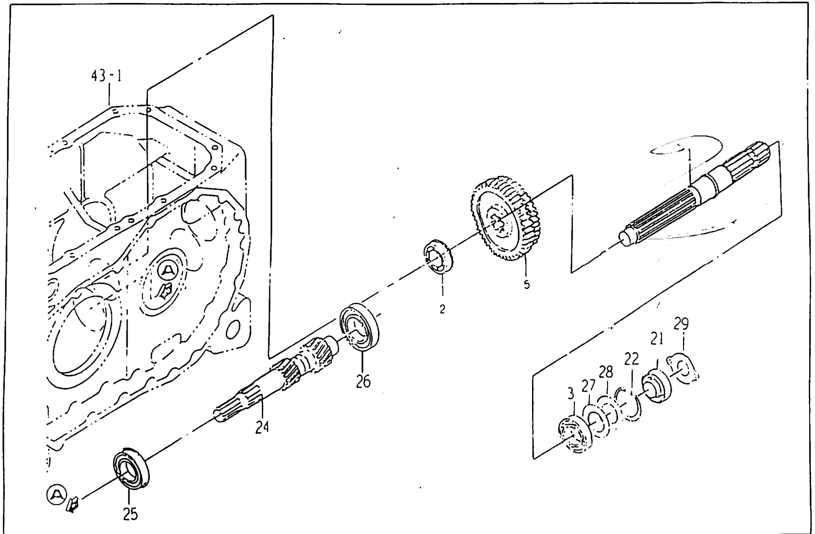
FIG : 51. P.T.O 체인지 기어 관계(P.T.O CHANGE GEAR)
