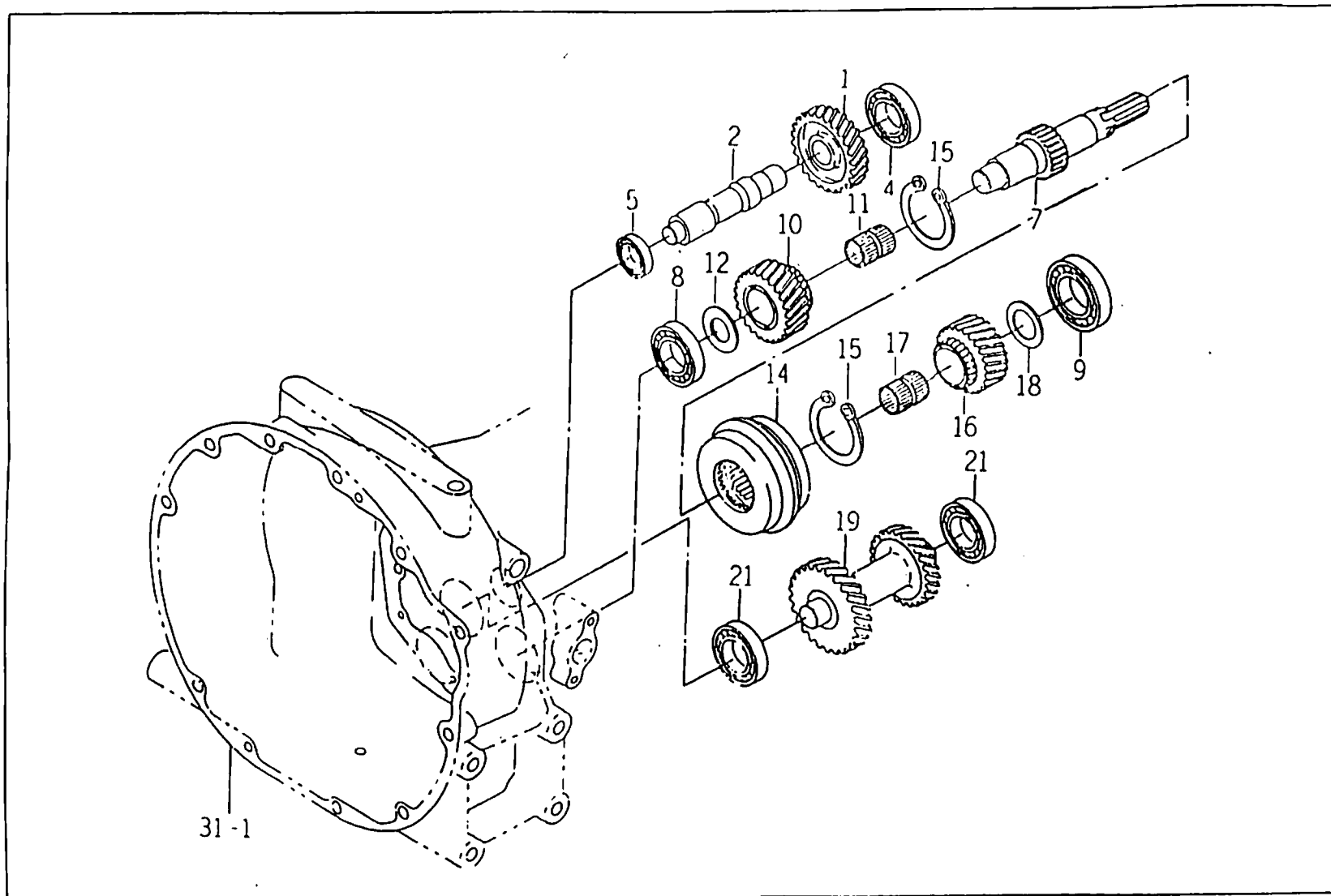
FIG : 34. 리버스 체인지 기어 관계(REVERSE CHANGE GEAR)
