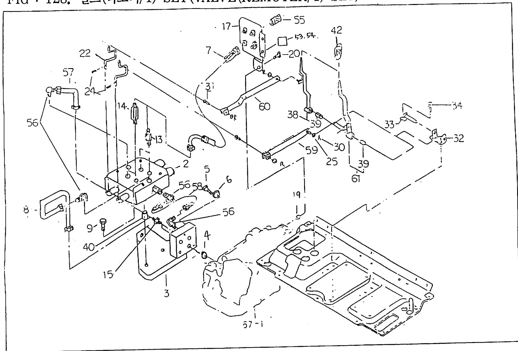
FIG : 128. 밸브(리모터/1) SET (VALVE(REMOTER/1) SET)
