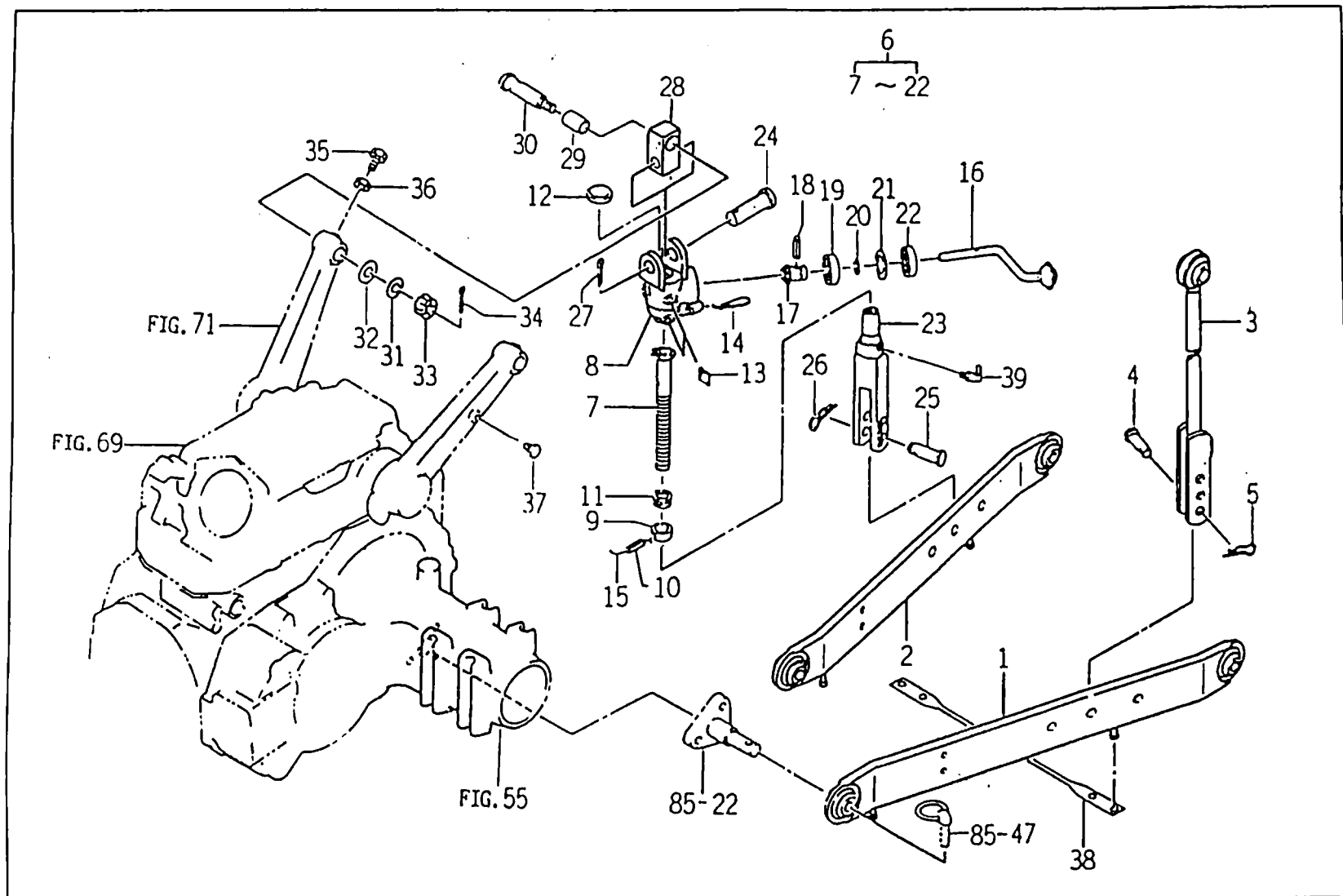
L 0012.1A FIG : 86. 로아링크 및 리프트 로드 관계(ROAR LINK & LIFT ROD)
