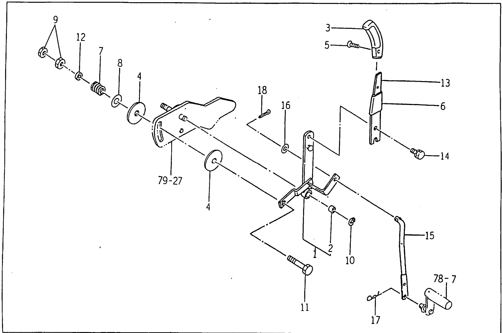
FIG : 80. 드레프트 레바 관계(DRAFT LEVER)
