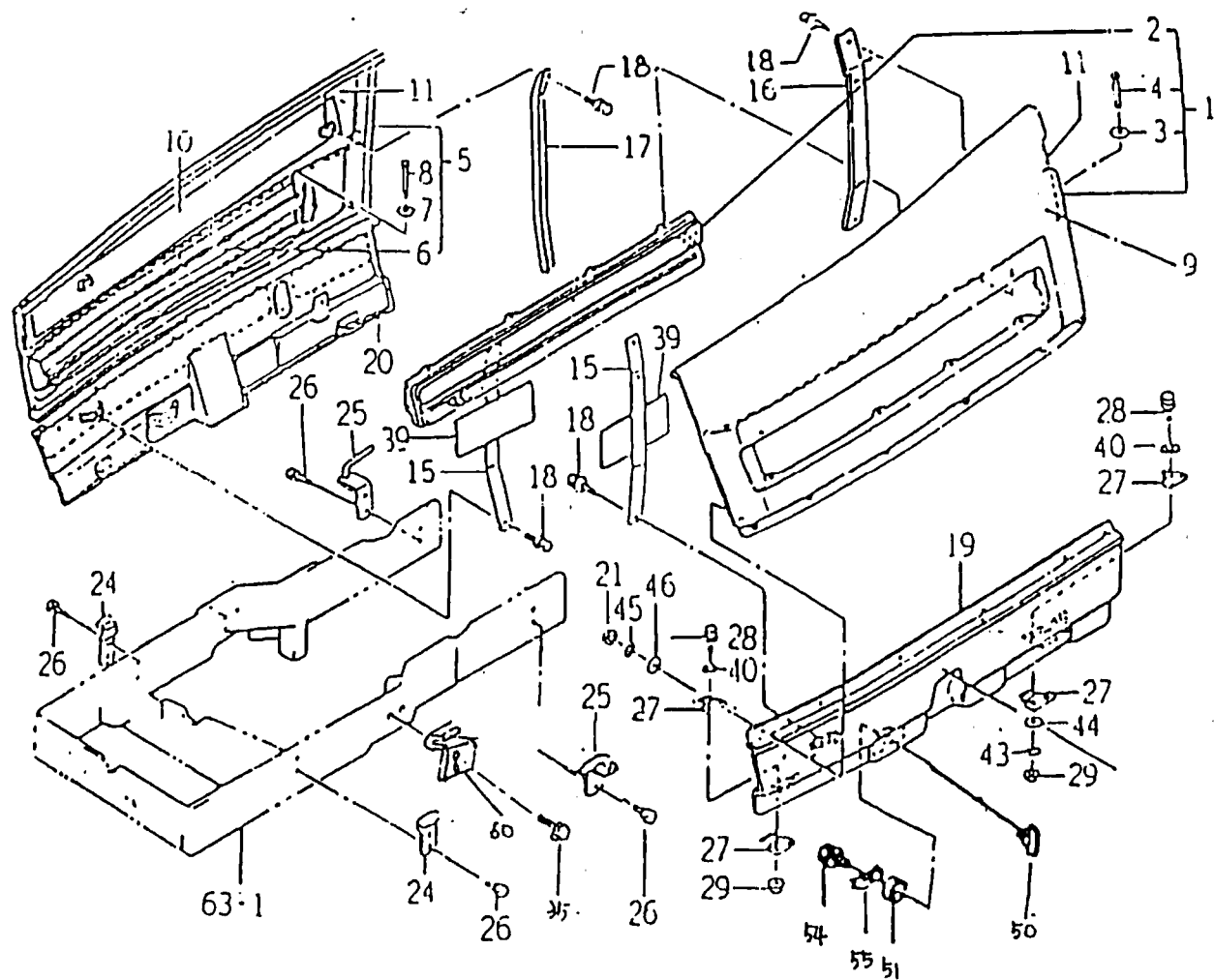
FIG : 92. 팬카바 관계(FAN COVER)
