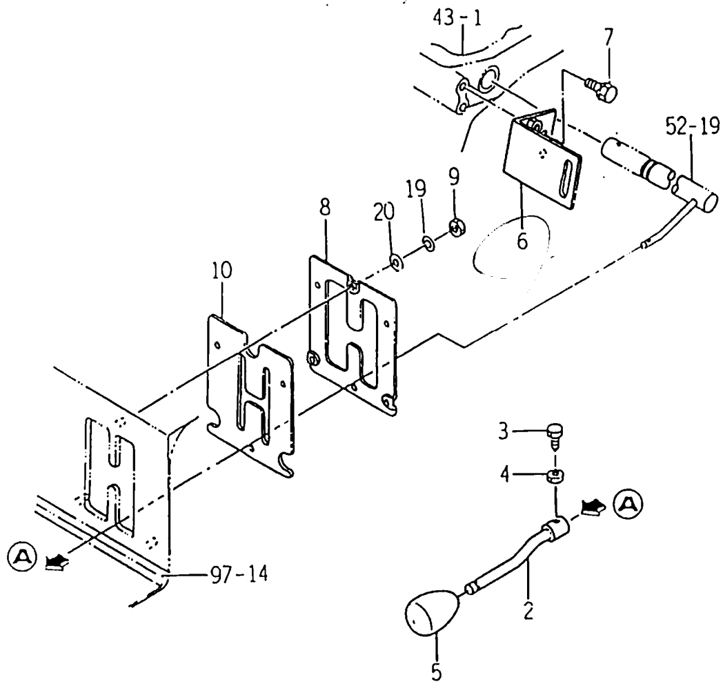
FIG : 53. P.T.O 레바 관제(P.T.O LEVER)
