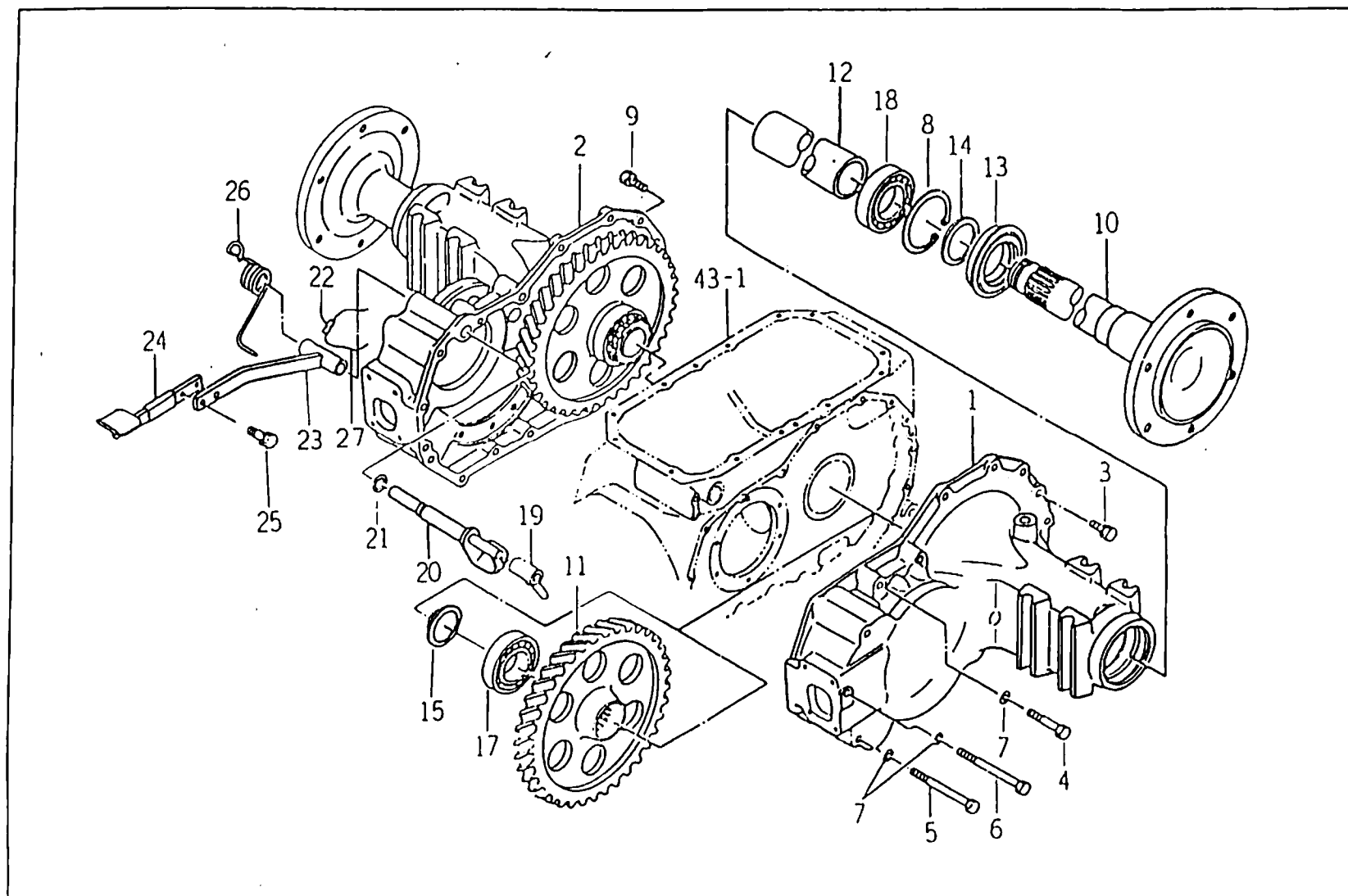
FIG : 55. 리어 액슬하우징 관계 (REAR AXLE HOUSING)
