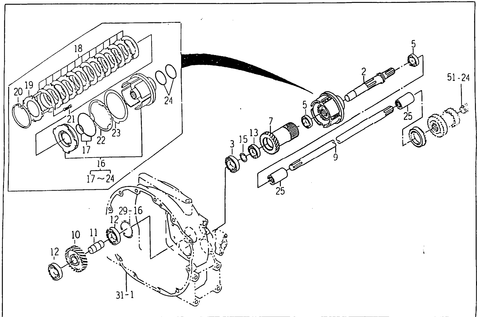
FIG : 36. P.T.O 드라이브 샤프트 관제(P.T.O DRIVE SHAFT)
