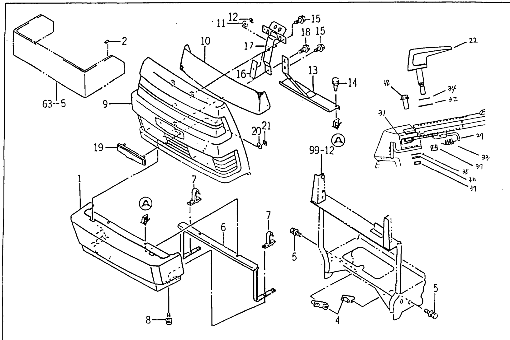
FIG : 91. 본넷 관계(2) (BONNET 2)
