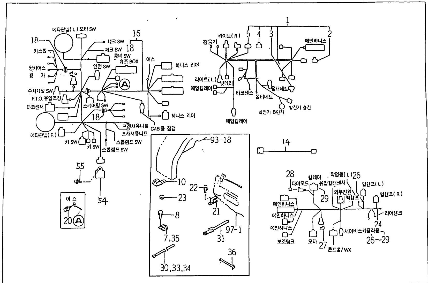
FIG : 106. 하니스 관계(1) (HARNESS 1)
