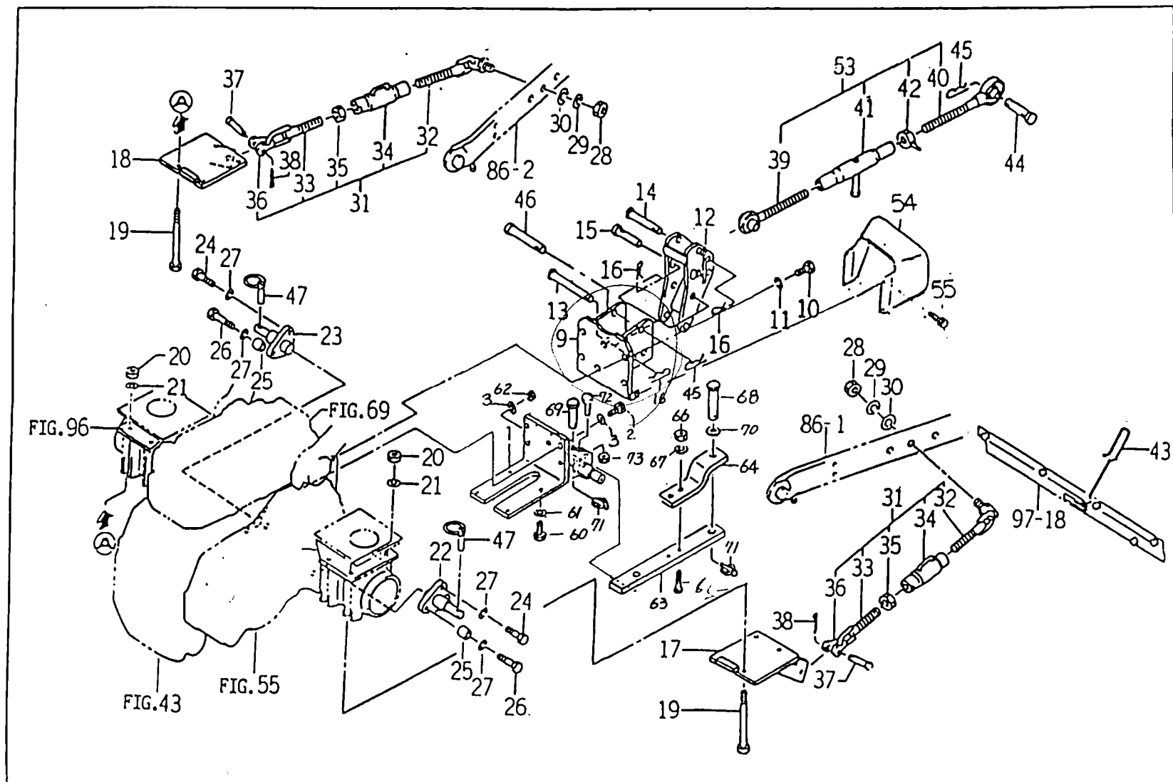
FIG : 85. 히치 및 3P링크 관계(HITCH & 3 POINT LINK)
