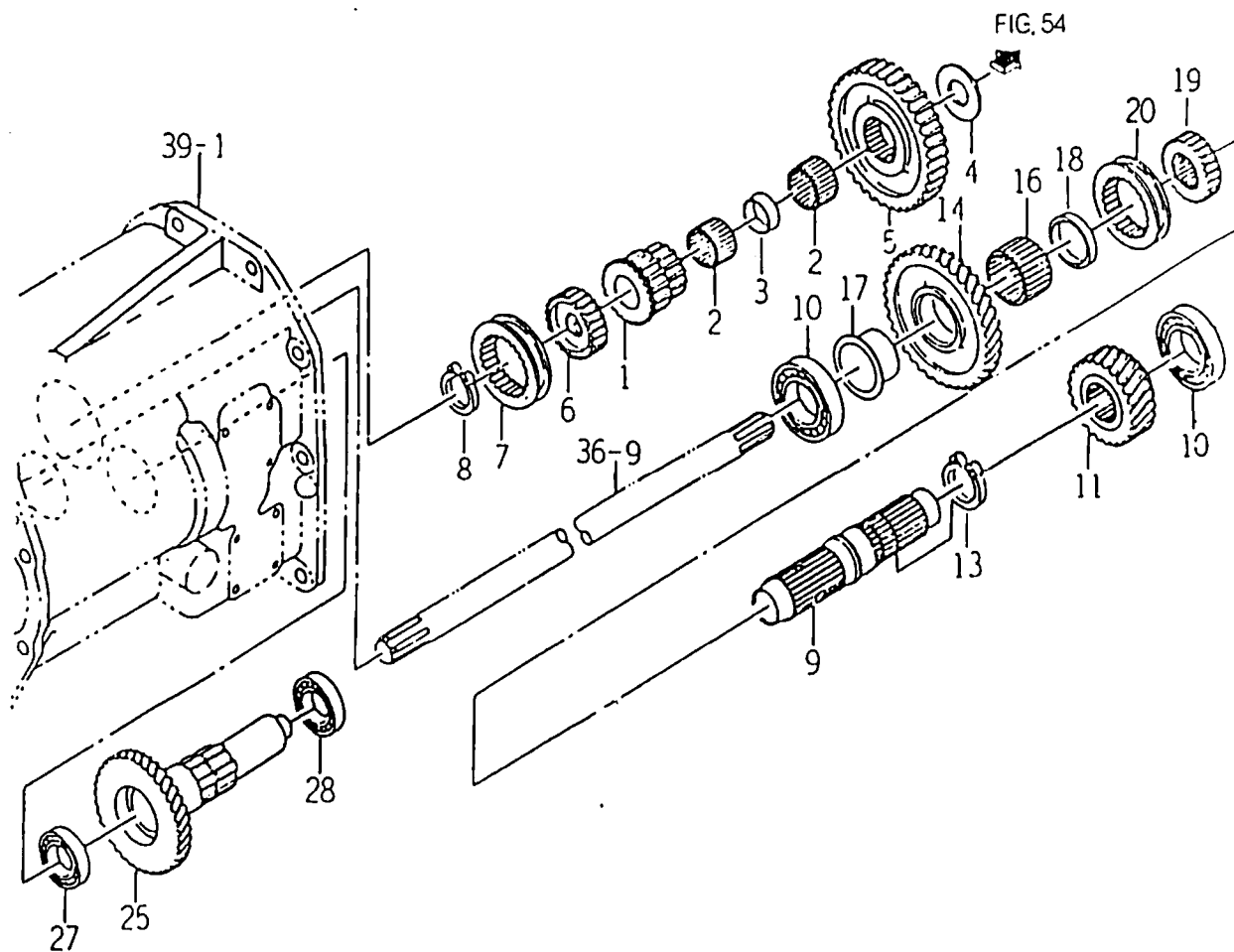
FIG : 44. 서브 체인지 기어 관계(SUB - CHANGE GEAR)
