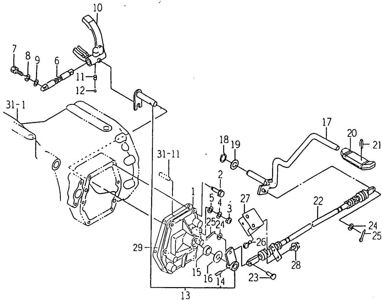
FIG : 38. 리버스 체인지 관제(REVERSE CHANGE)
