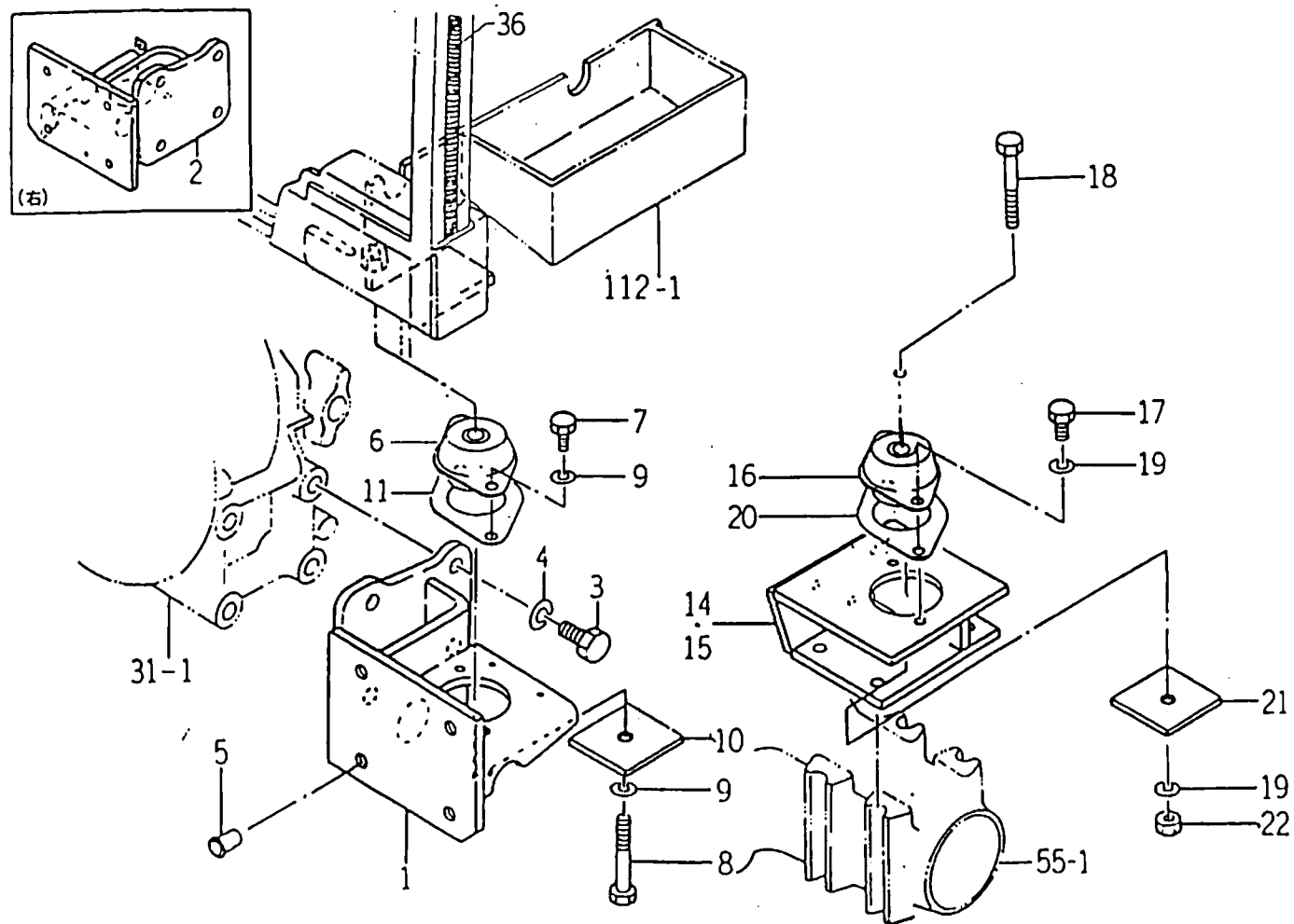
FIG : 96. 프론트 및 리어 마운트 관제(FRONT & REAR MOUNT)
