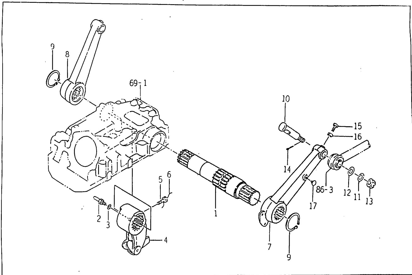
FIG : 71. 리프트 암 관계(LIFT ARM)
