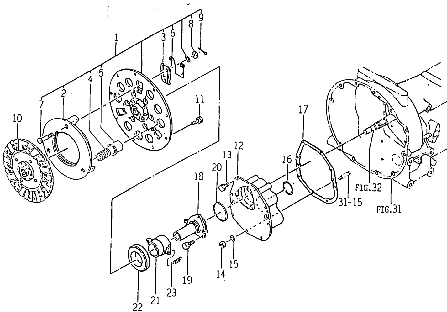
FIG : 29. 클러치 관계(CLUTCH)
