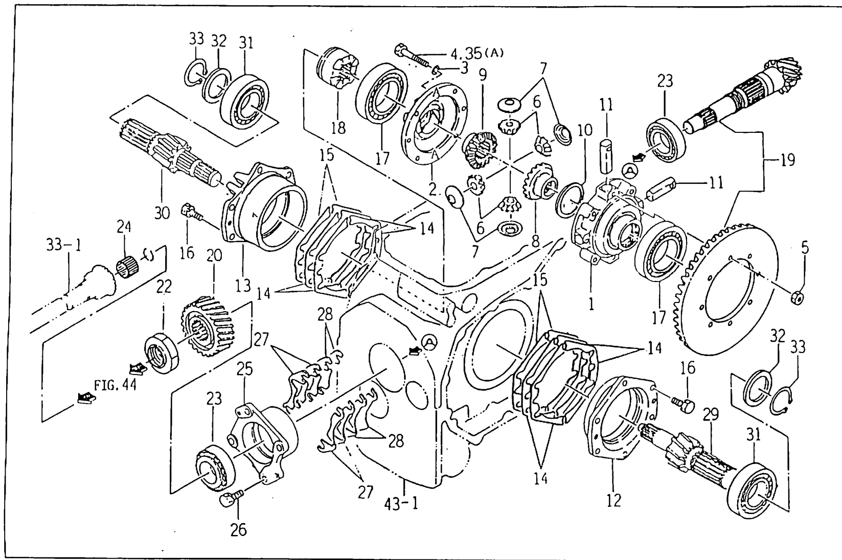
FIG : 54. 디프케이스 관제(DIFF CASE)
