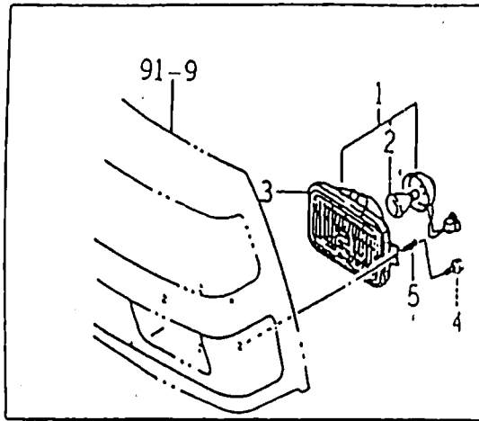
FIG : 100. 전장 관계(2) (ELECTRIC SYSTEM 2)
