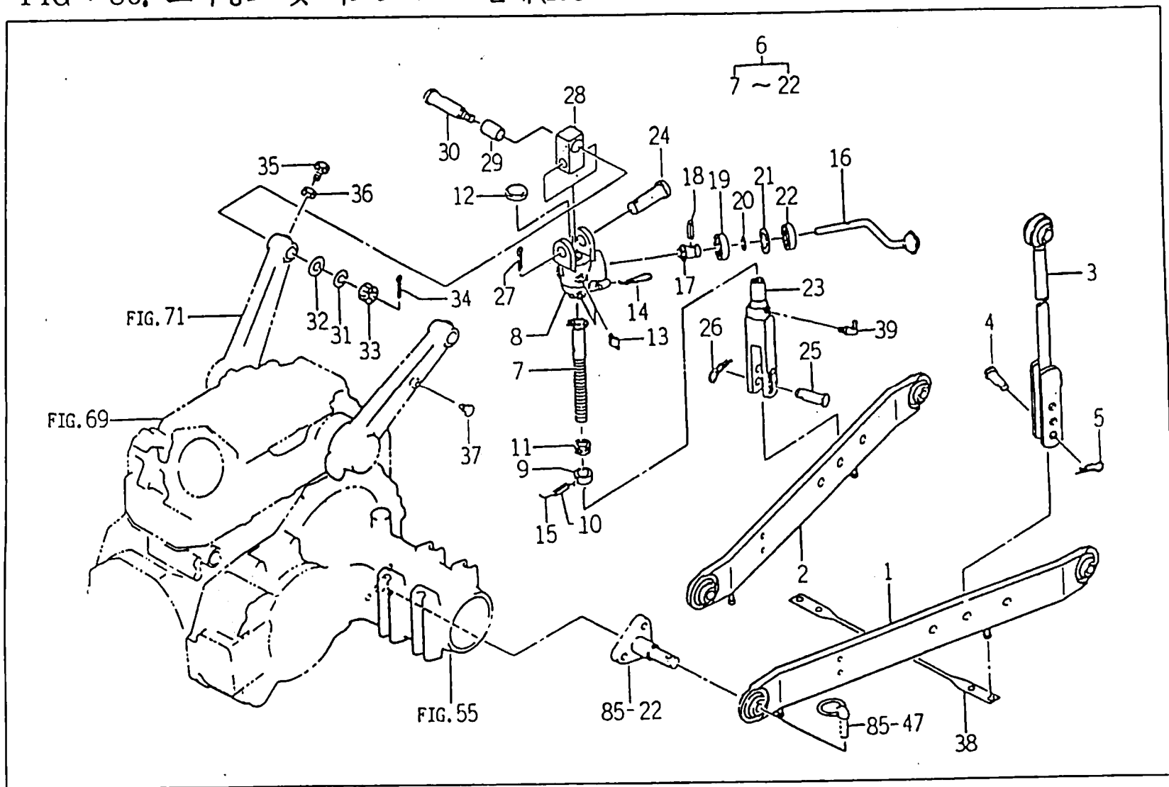
FIG : 86. 로아링크 및 리프트 로드 관계(ROAR LINK & LIFT ROD)
