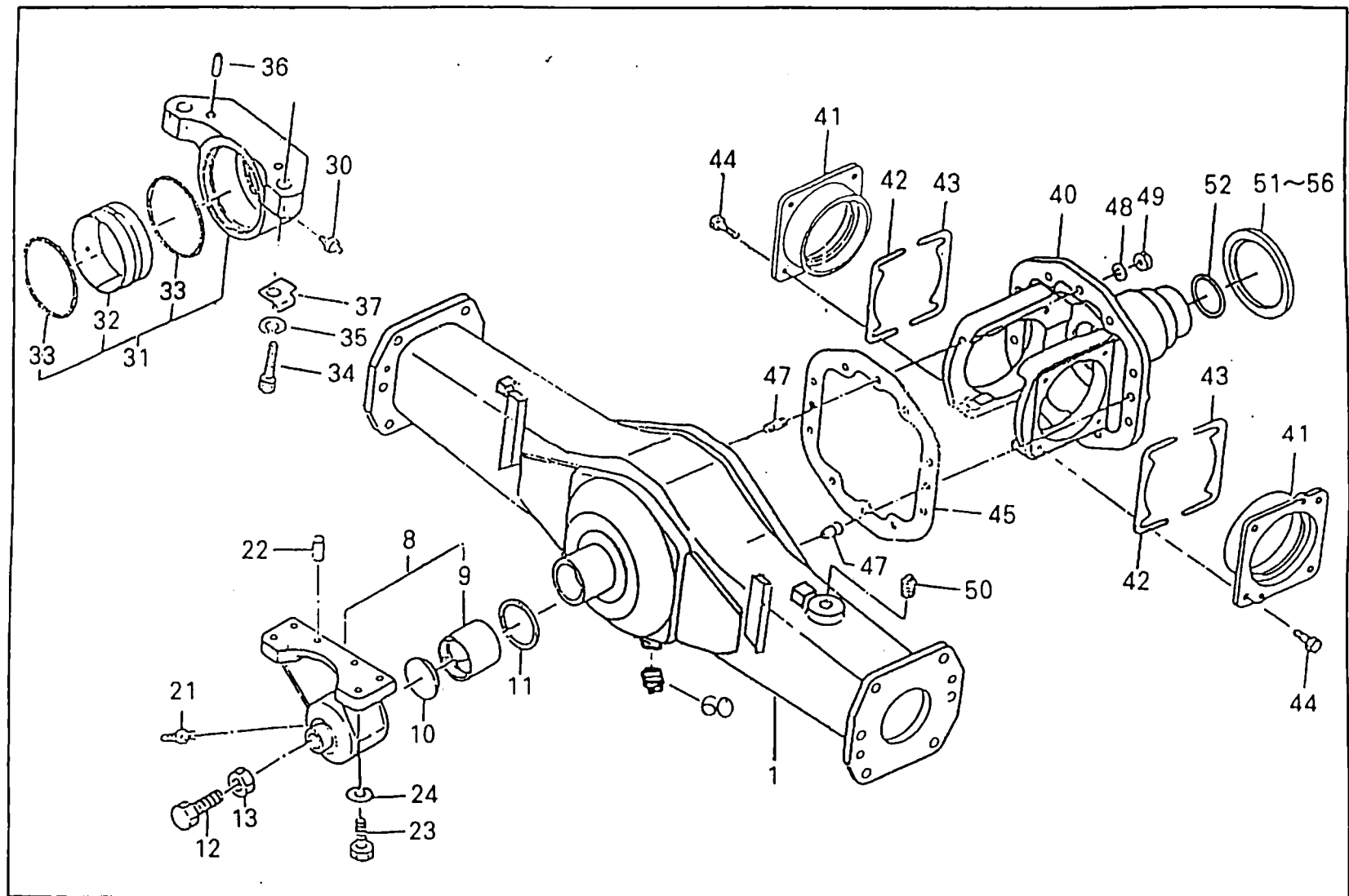
FIG : 65. 액슬 하우징 관계 (AXLE HOUSING)
