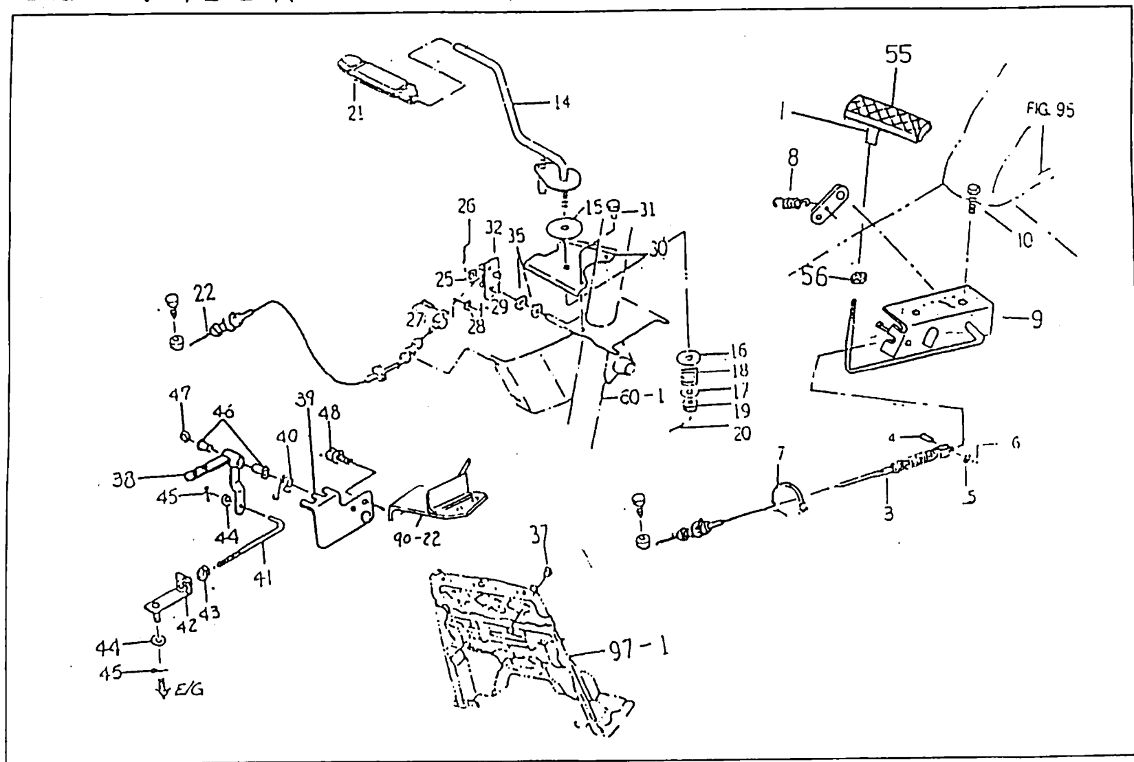
FIG. 27. 액셀 관계(ACCELERATOR)
