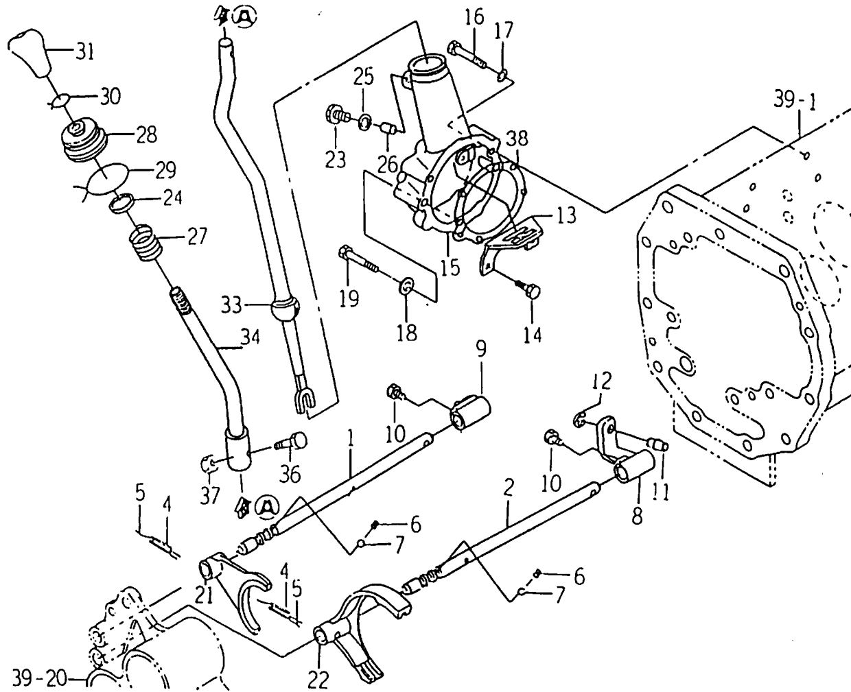
FIG : 37. 메인 체인지 관계(MAIN CHANGE)
