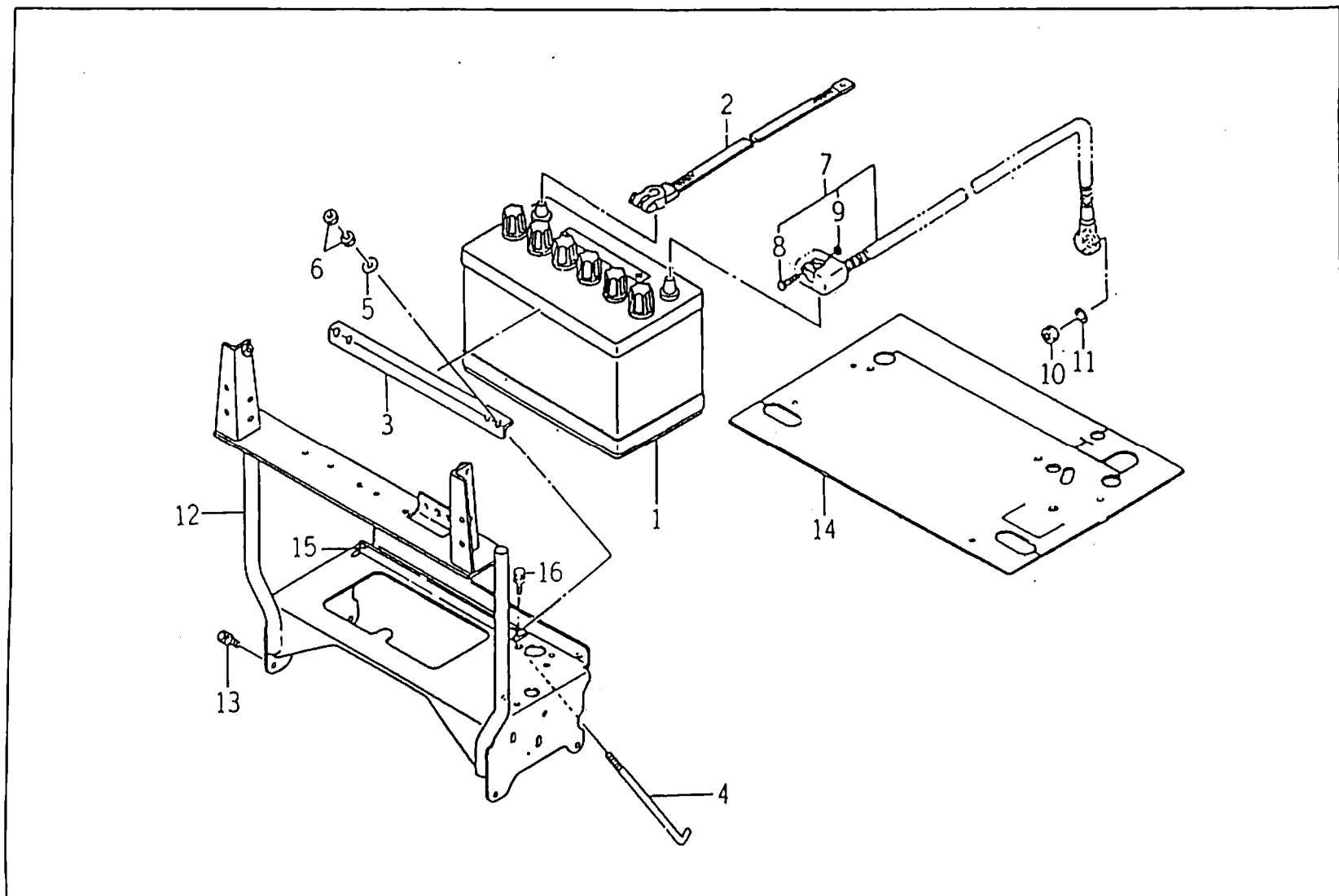
FIG : 99. 전장 관계(1) (ELECTRIC SYSTEM 1)
