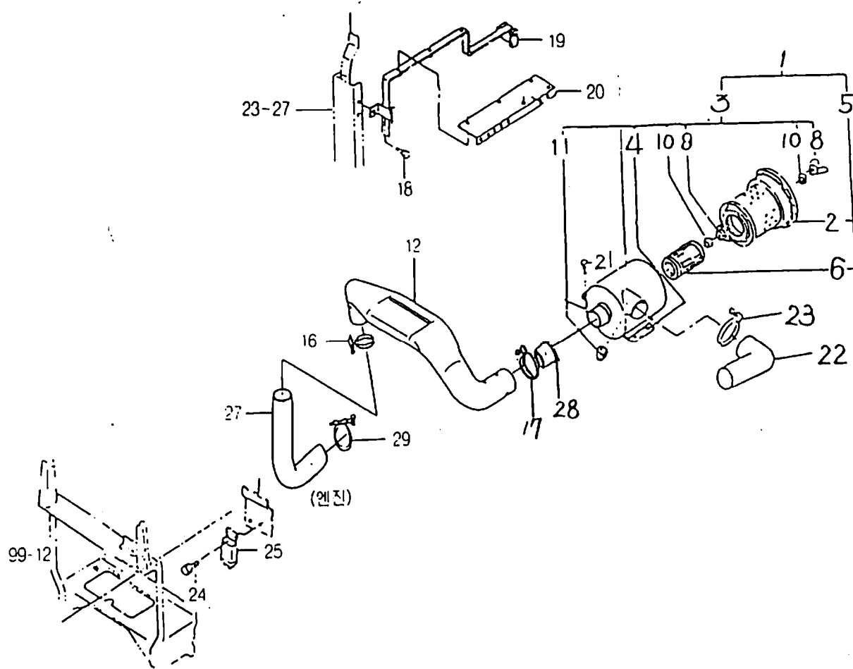
FIG : 22. 에어크리너 관계(AIR CLEANER)
