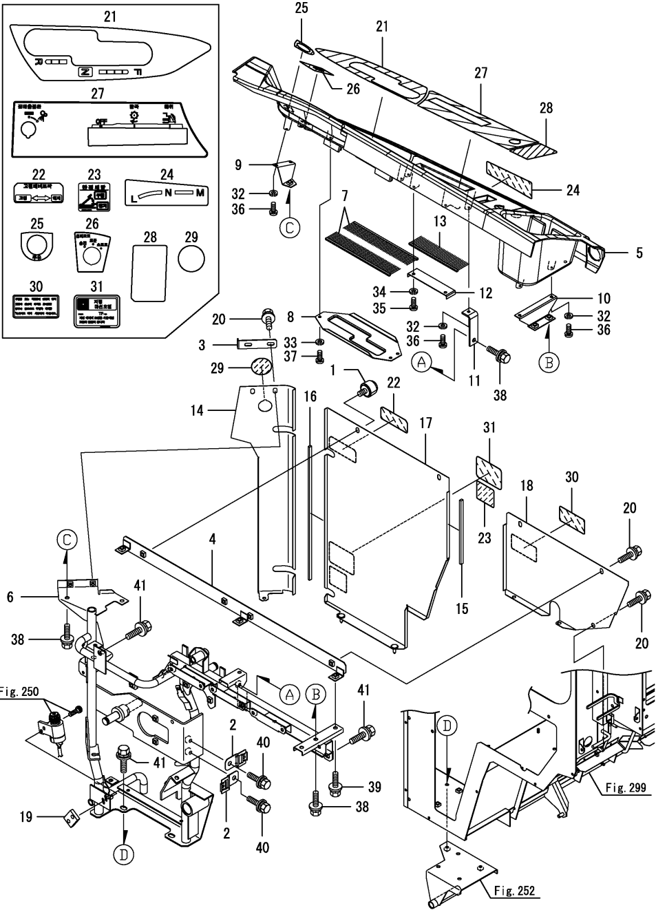
Fig.245. 사이드칼럼(1)
