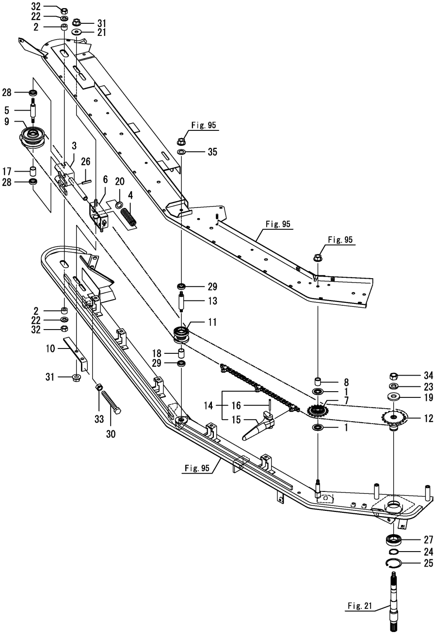
OCNP6-M05021 수확(2) Fig.100. 상반송롤러(우)
