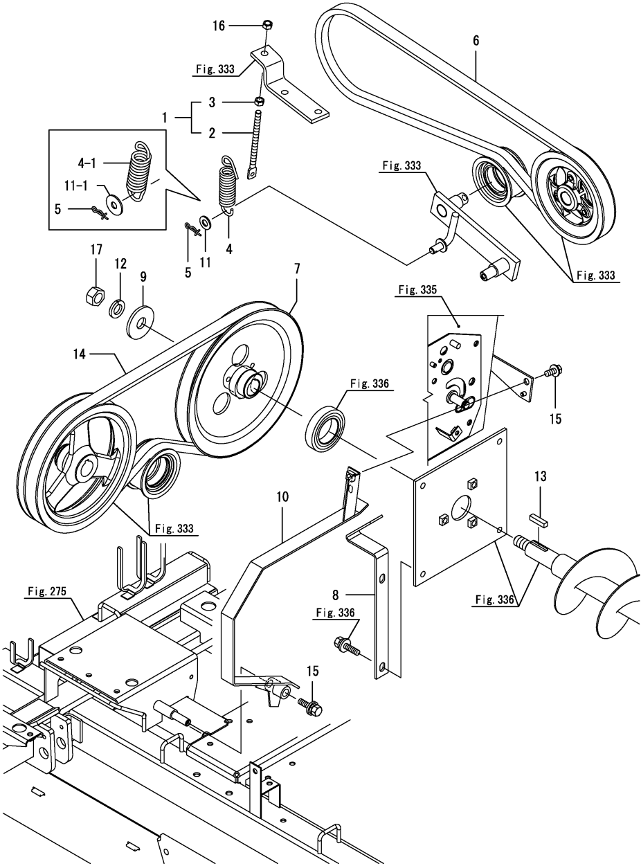
Fig.334. 오거 벨트
