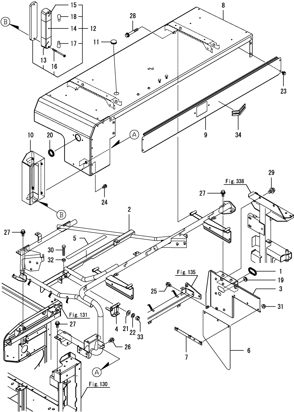
Fig.200. 쥘배출프레임(상)
