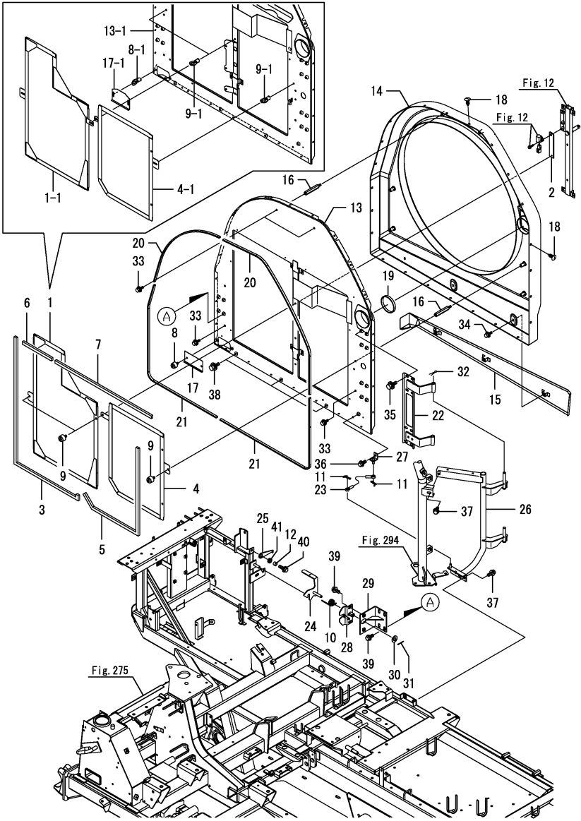
Fig.295. 엔진실 커버
