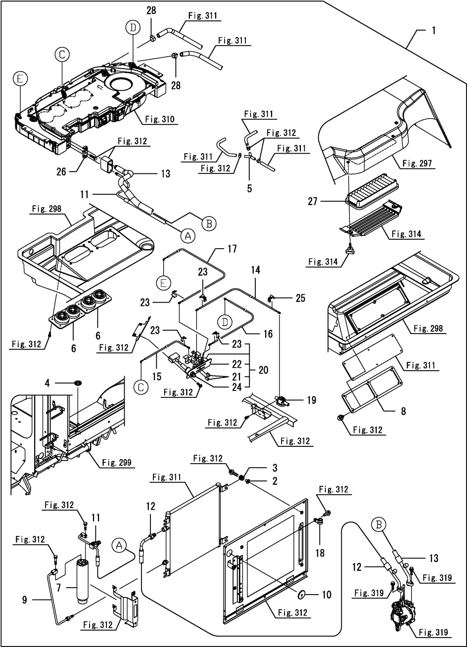
Fig.309. 에어컨(1)
