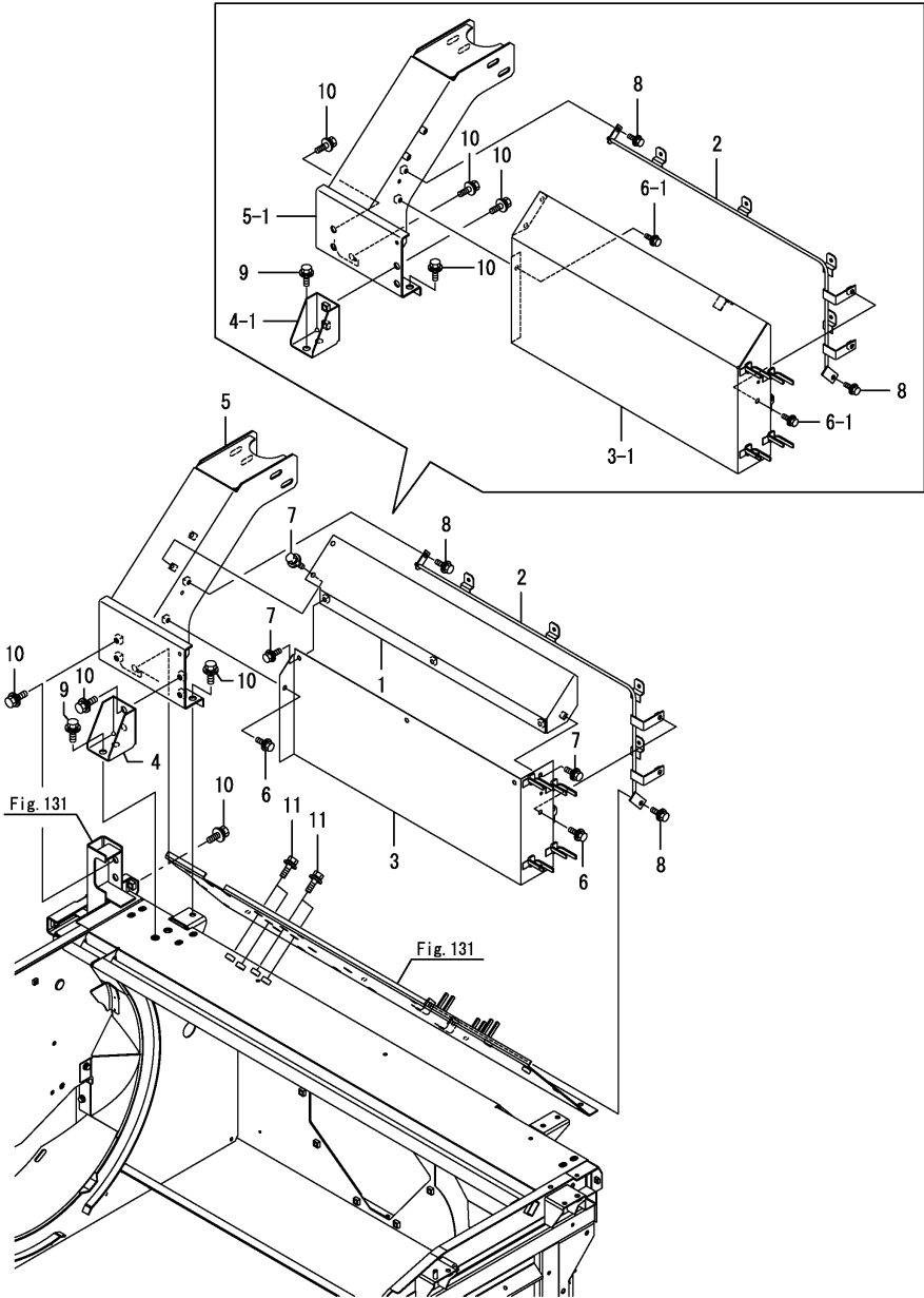
Fig.349. 탱크 고정
