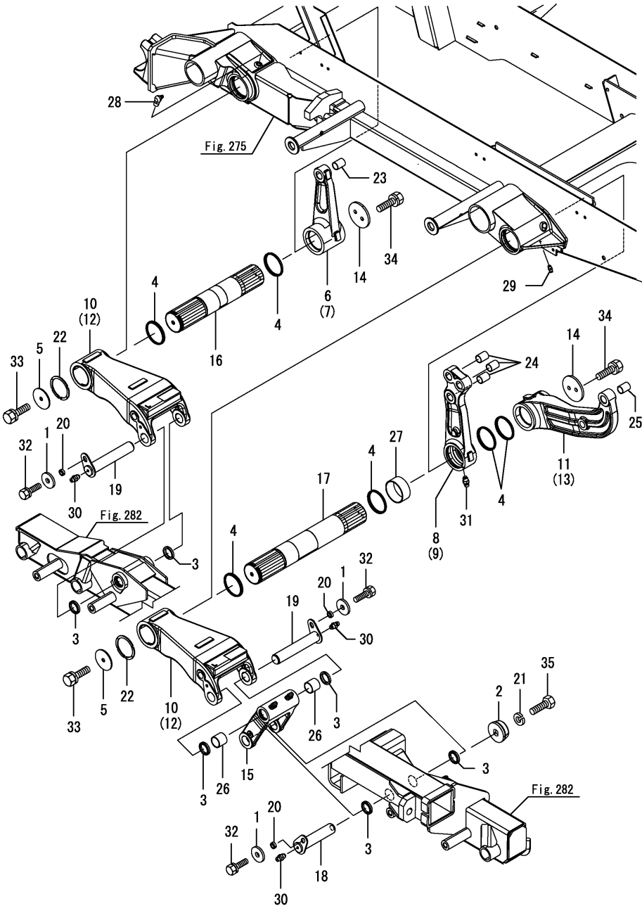
OCNP6-M05021 이동(3) Fig.292. 스윙(1)(피칭 U.F.O.)
