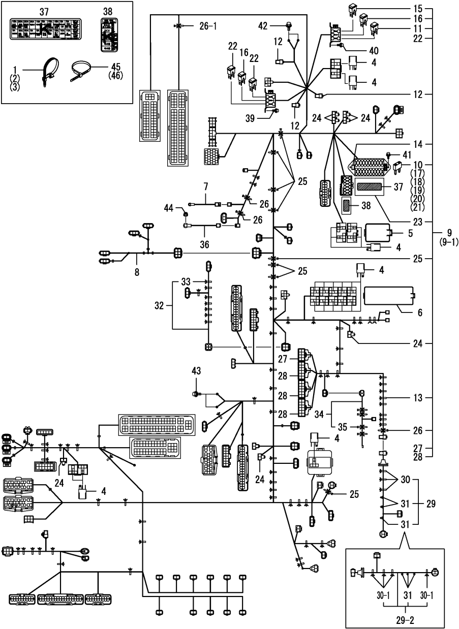
Fig.322. 배선(주행)
