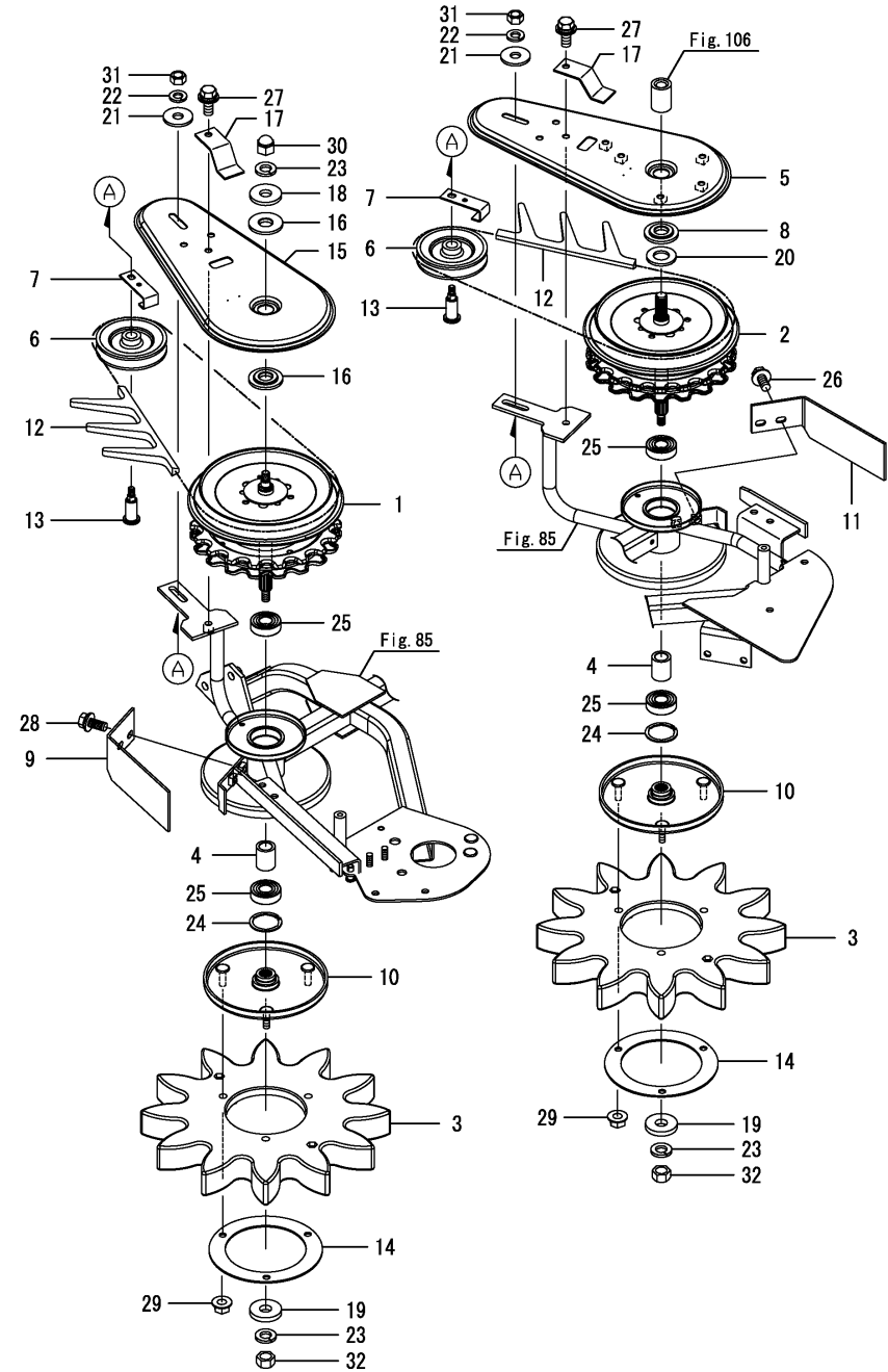
OCNP6-M05021 수확(2) Fig.76. 스타휠(중-우)
