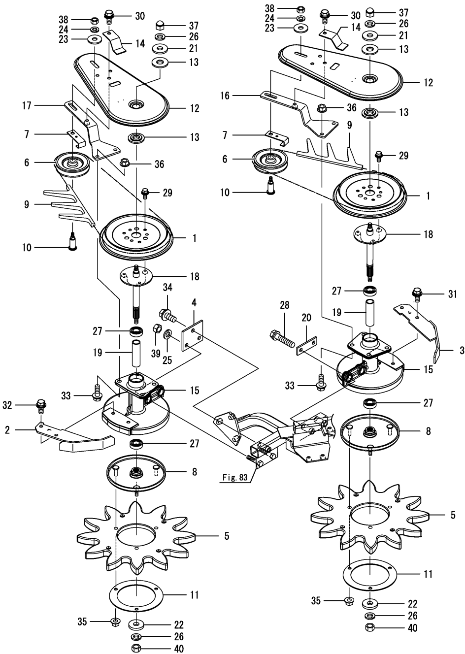
Fig.74. 스타휠(중-좌)
