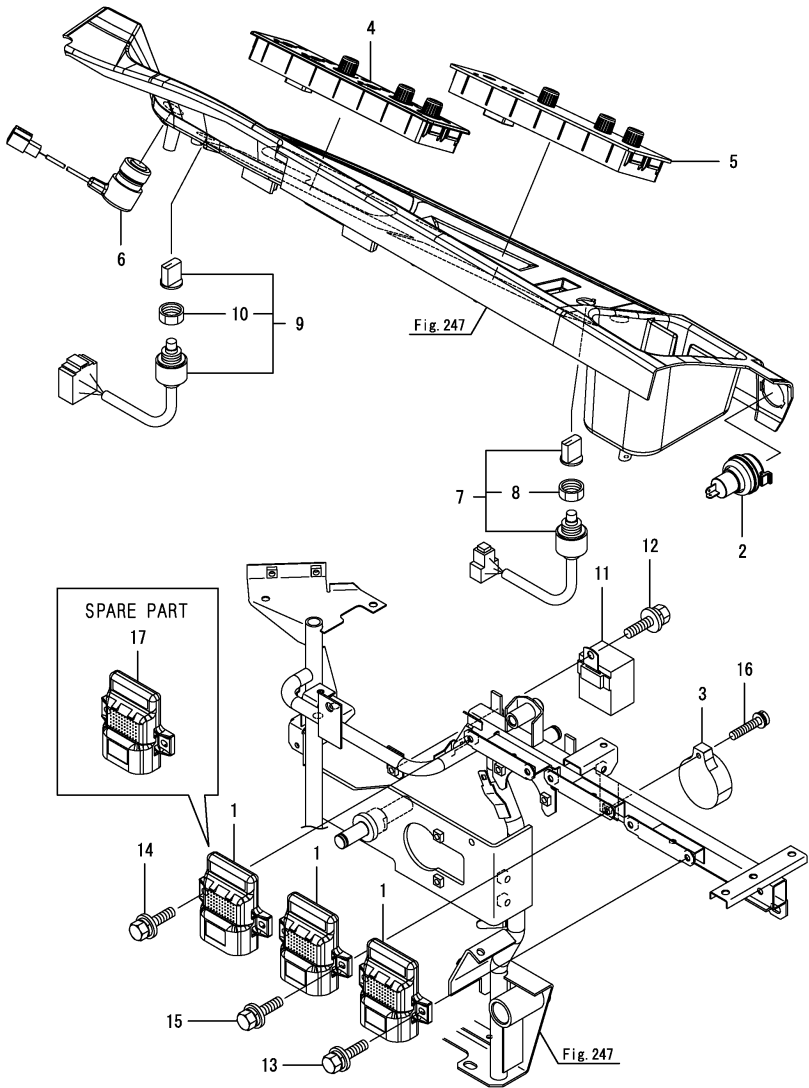
Fig.248. 측면 컬럼(2)(피칭 U.F.O.)
