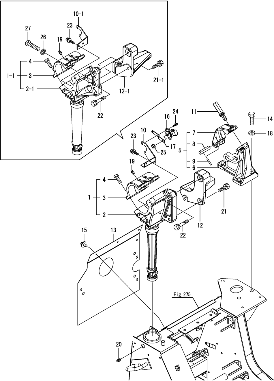
Fig.264. 회동지점
