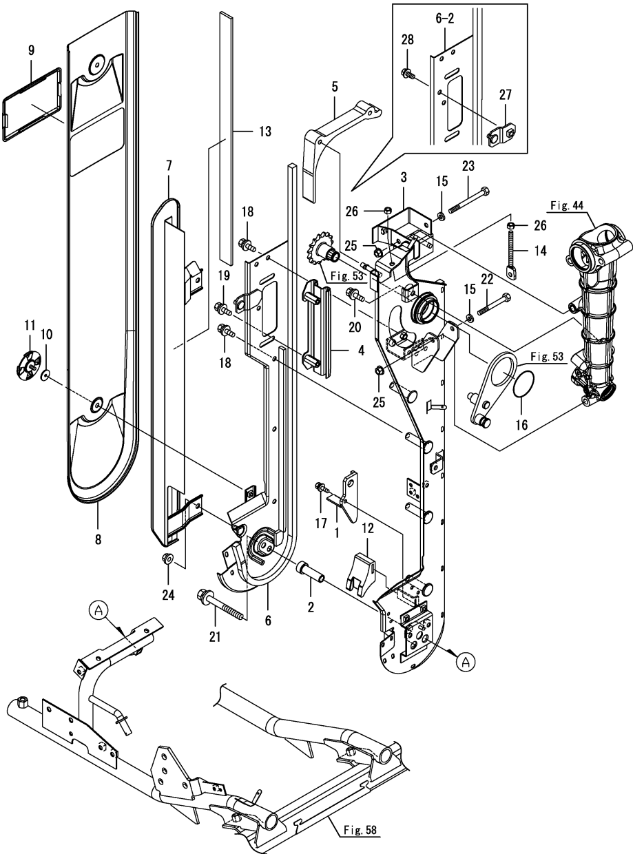
Fig.52. 픽업 케이스(중앙)(3)
