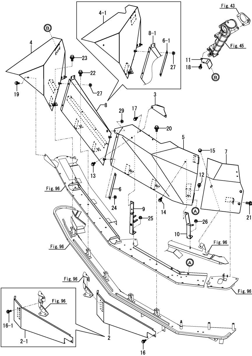
Fig.112. 상단 이송 가이드(오른쪽)
