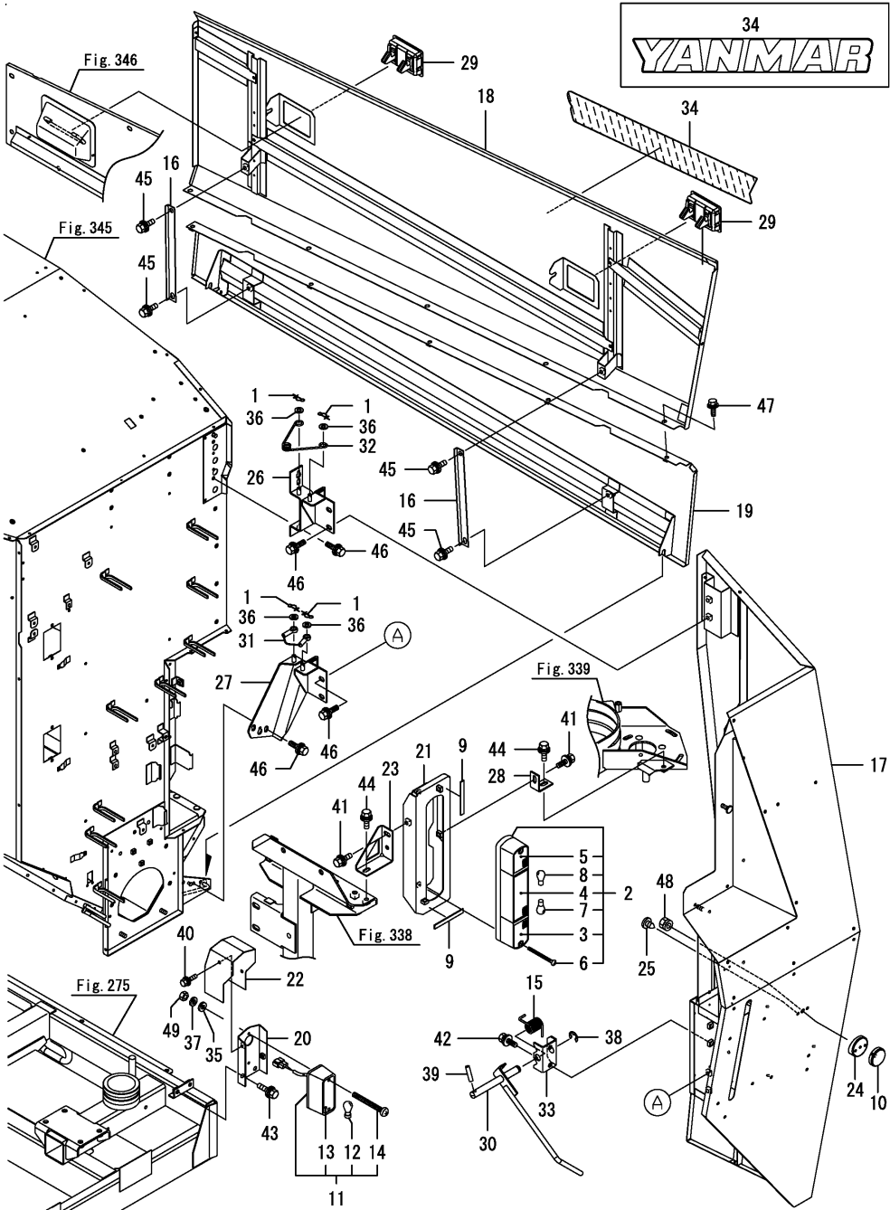
Fig.353. 탱크커버
