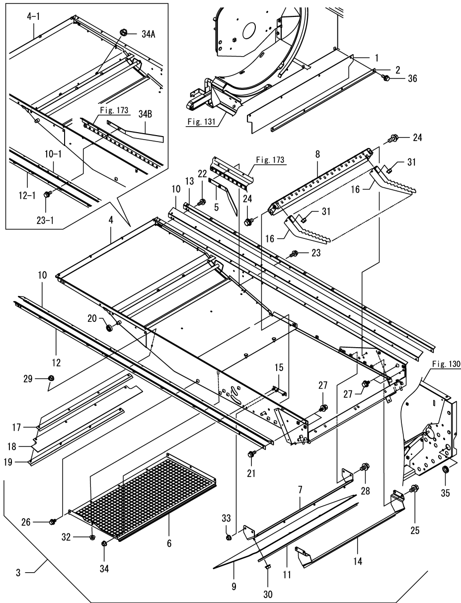
Fig.171. 요동선별프레임(1)
