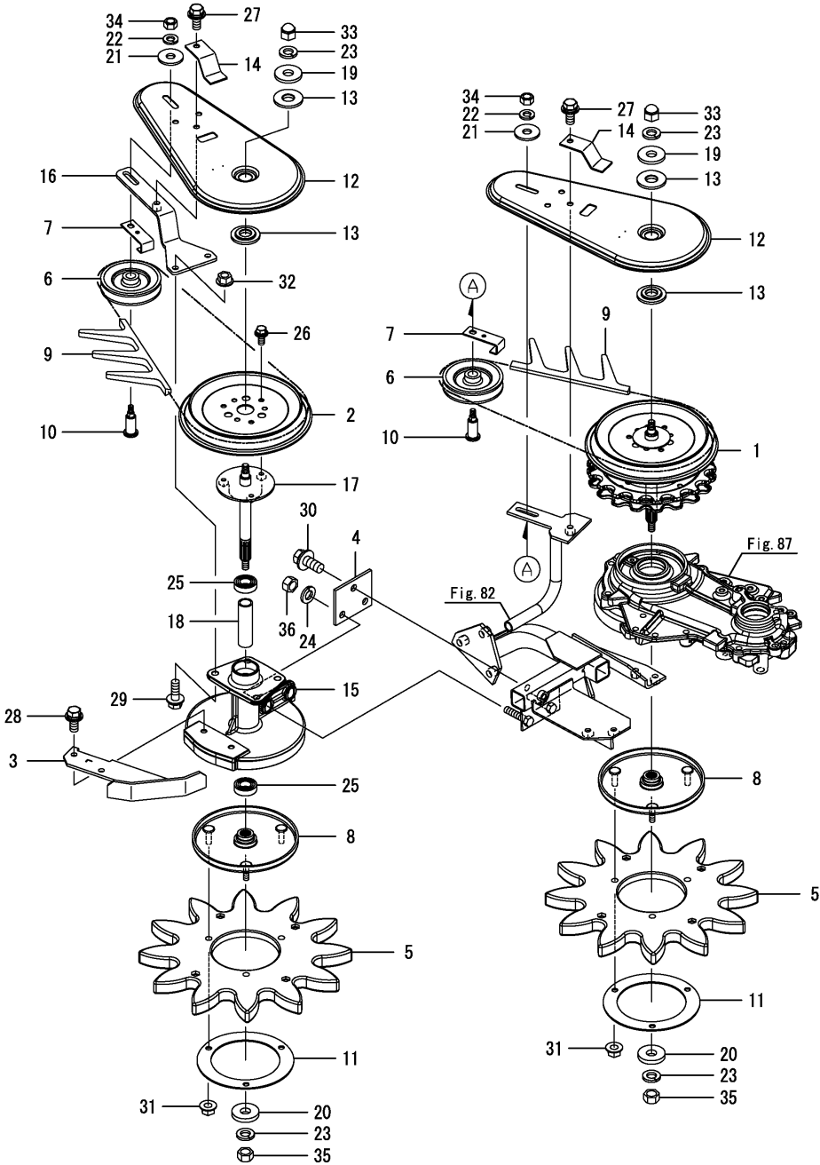
Fig.73. 스타휠(중-좌)
