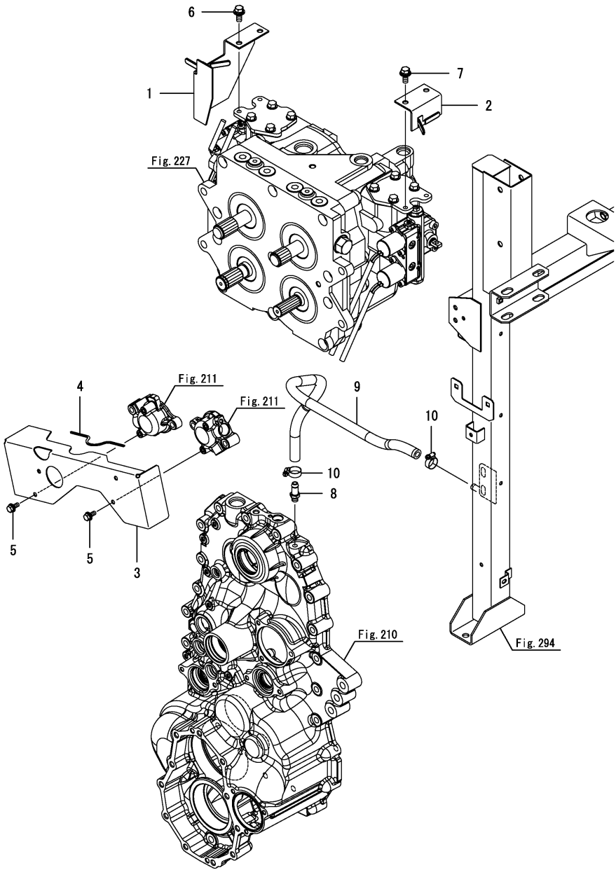
Fig.203. 미션커버
