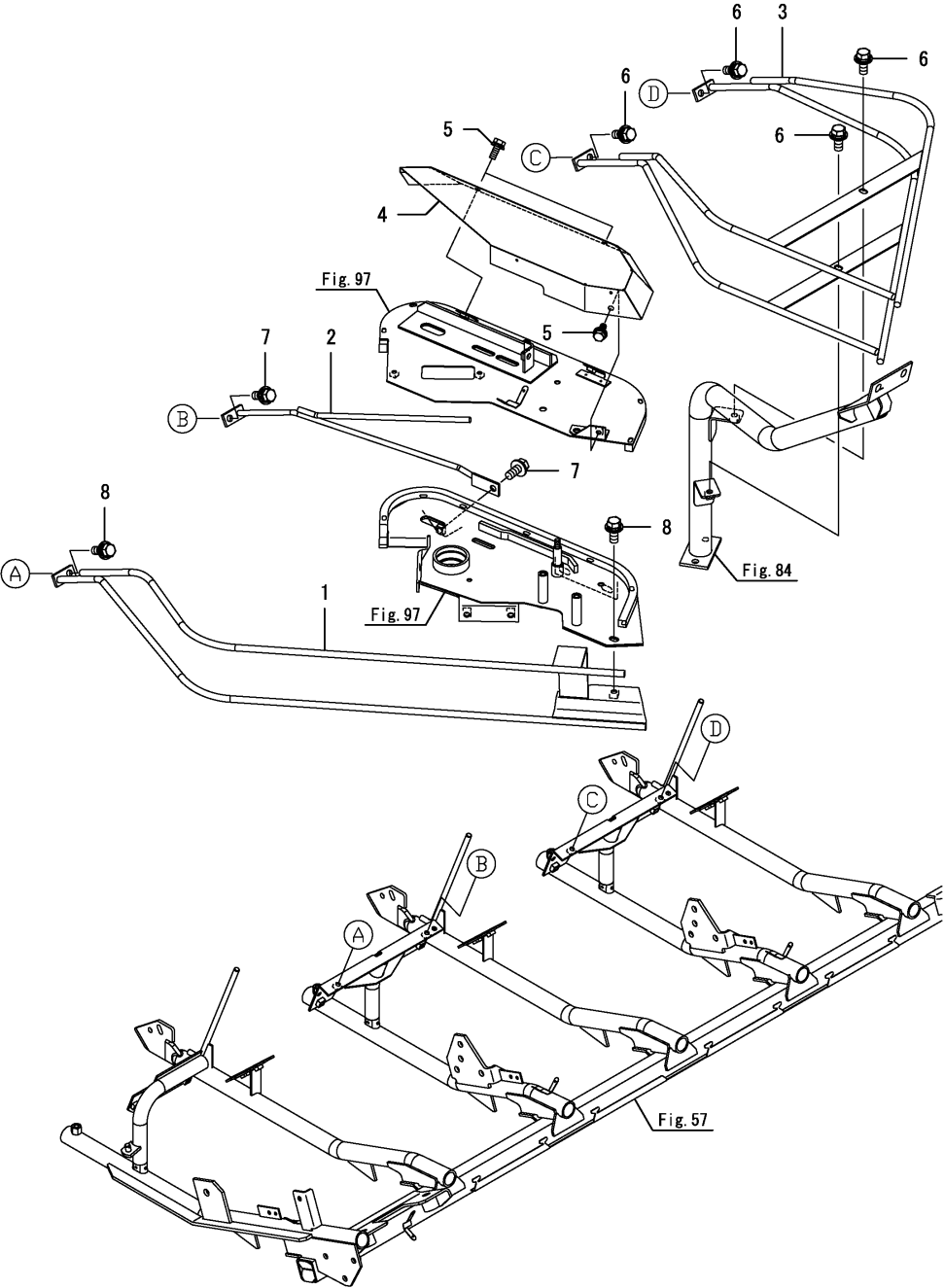
Fig.113. 상반송가이드(중)
