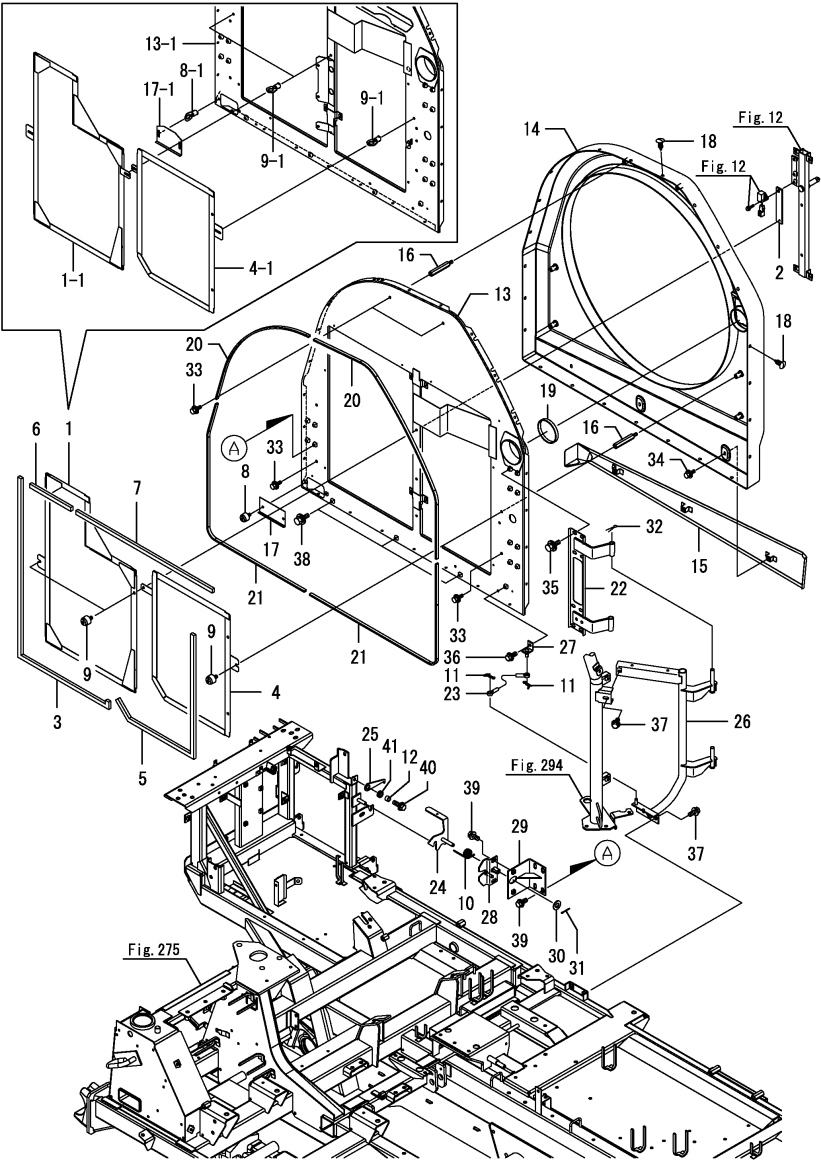
Fig.295. 엔진실 커버
