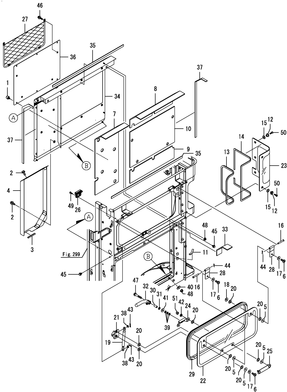
Fig.302. 캐빈 삭구(후면)
