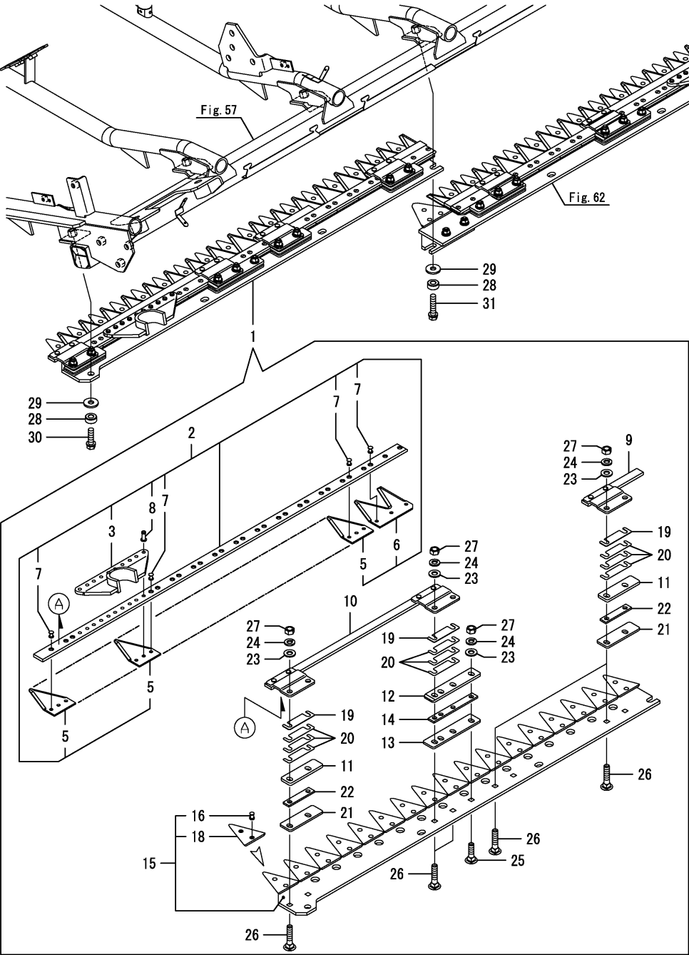
Fig.61. 예취날(좌)
