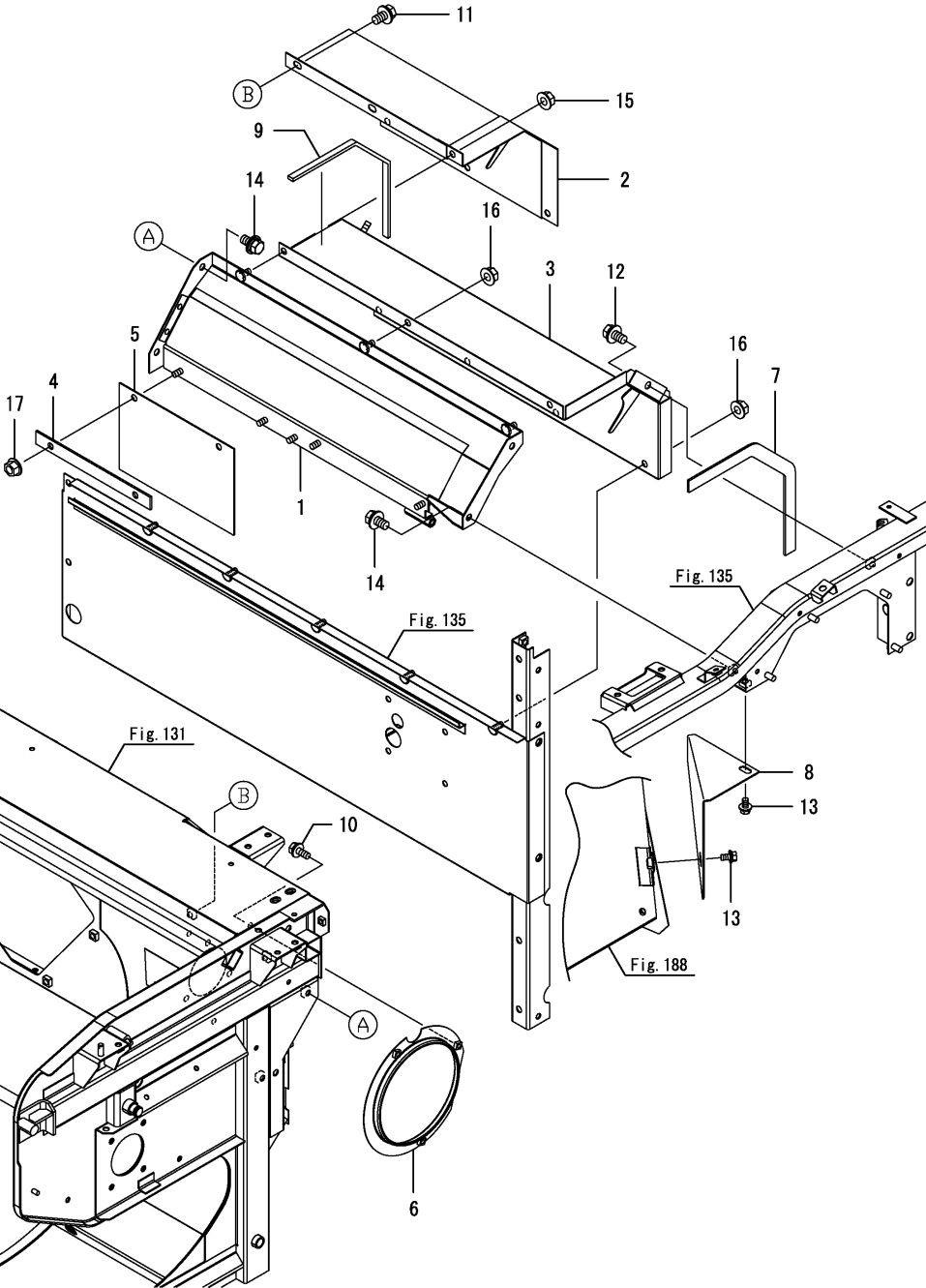
Fig.168. 처리 드럼 커버
