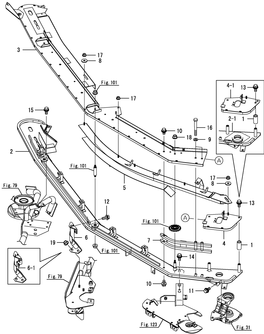
Fig.96. 상단 이송 케이스(오른쪽)
