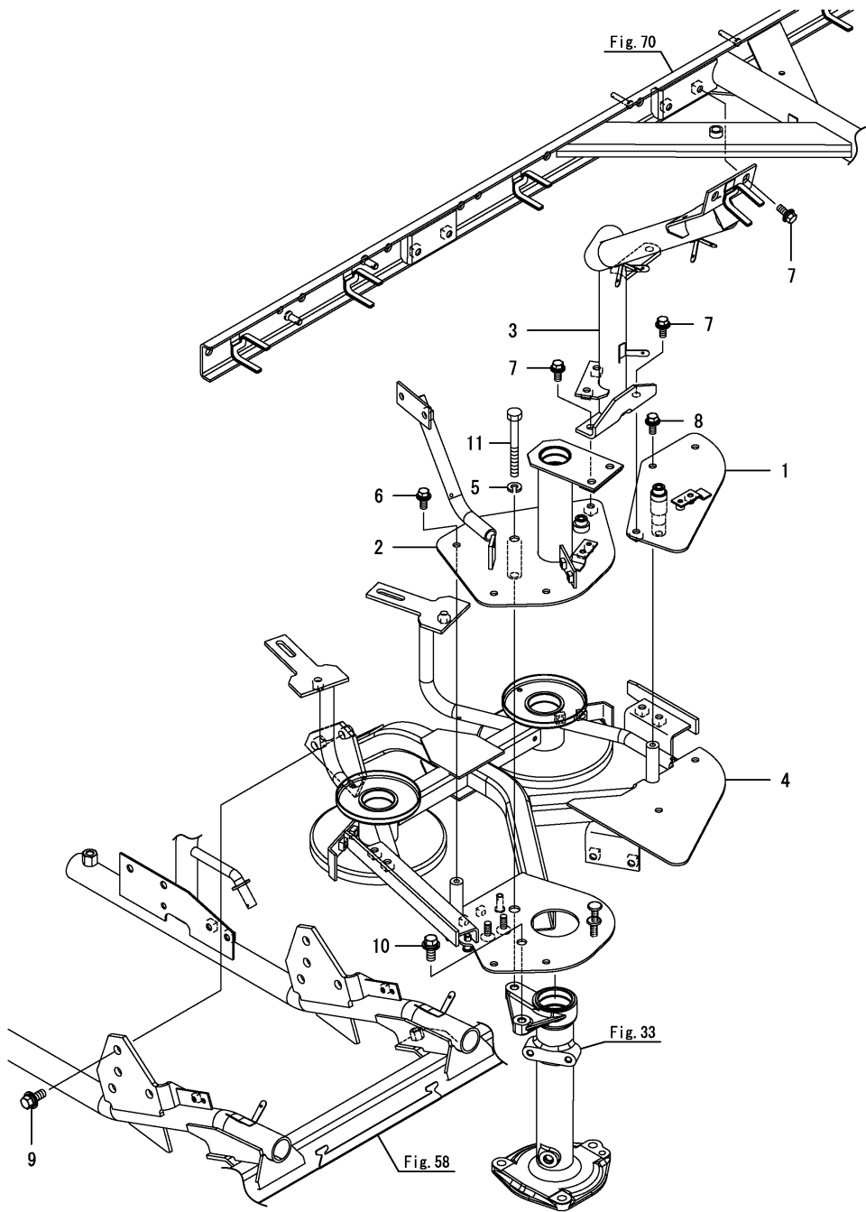
OCNP6-M05021 수확(2) Fig.85. 끌어모음프레임(중-우)
