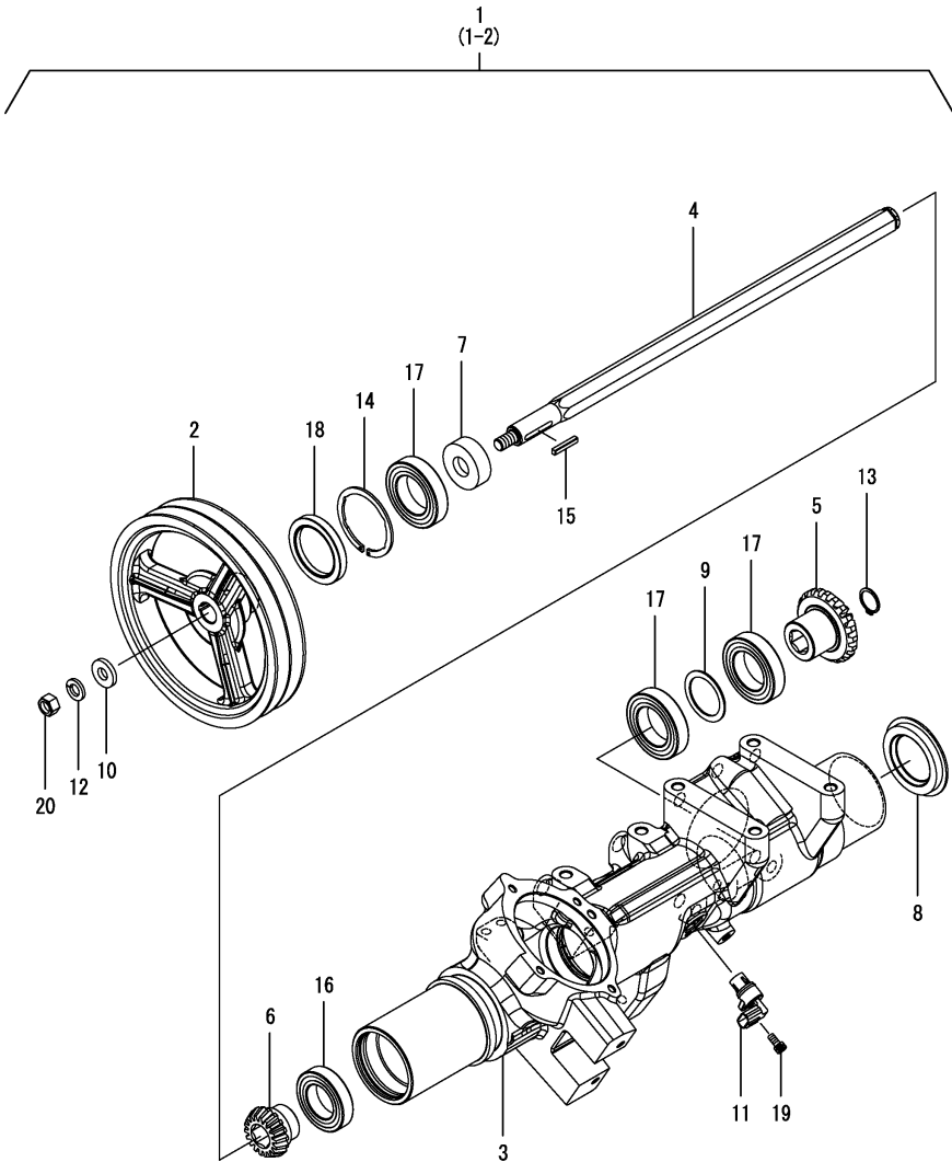
Fig.28. 7조구동케이스(1)
