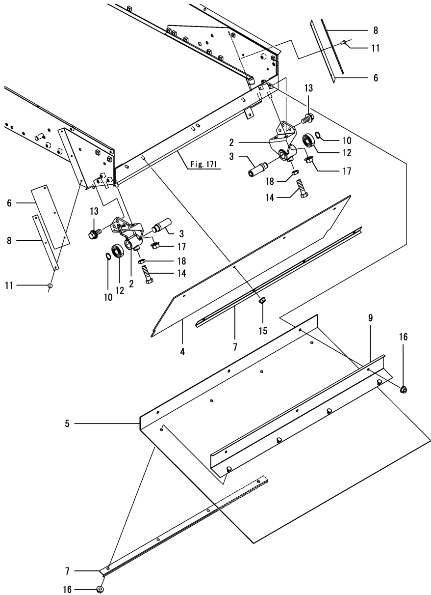
Fig.172. 요동선별프레임(2)
