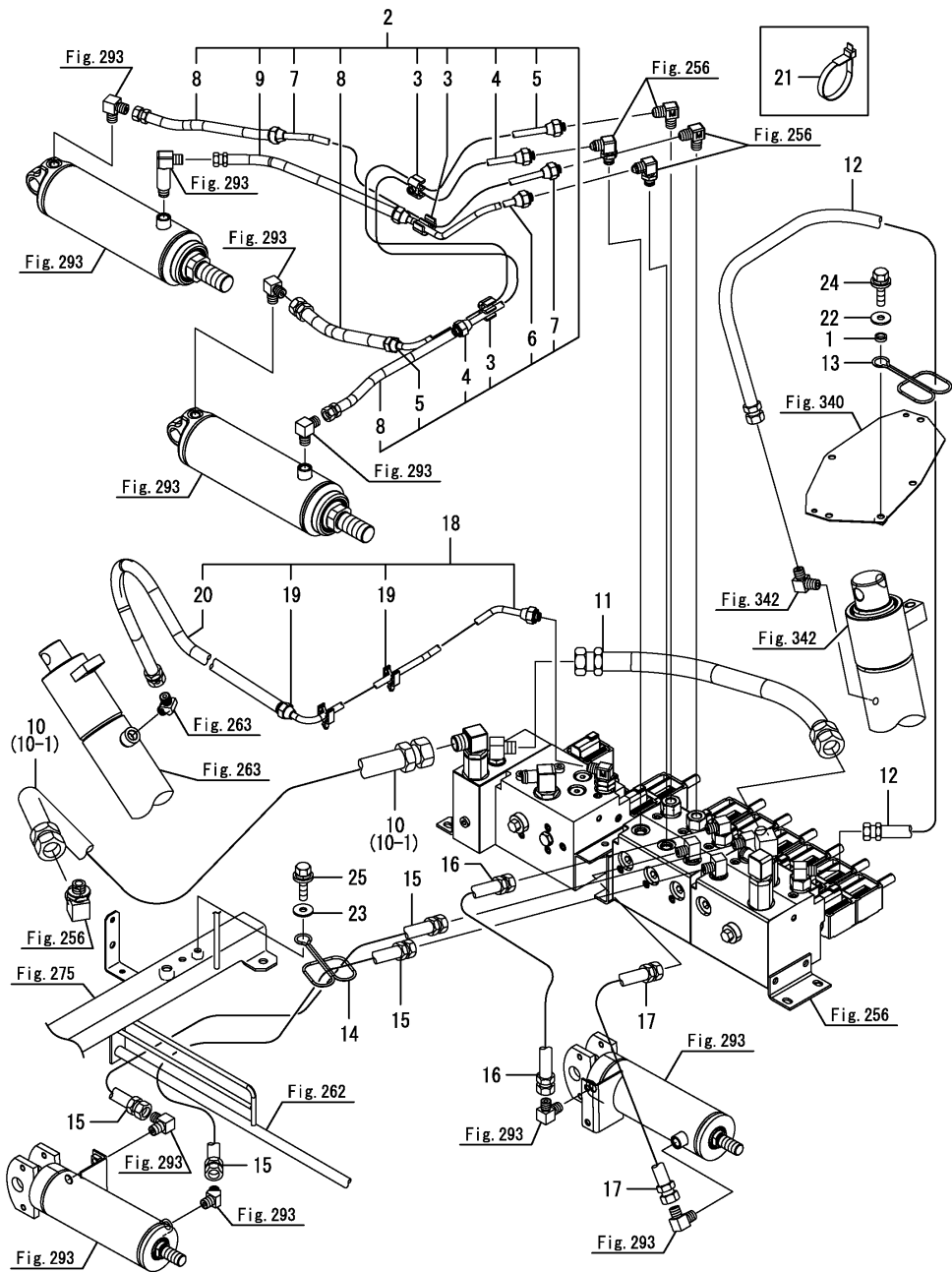
OCNP6-M05021 이동(2) Fig.261. 배관(1)(피칭 U.F.O.)
