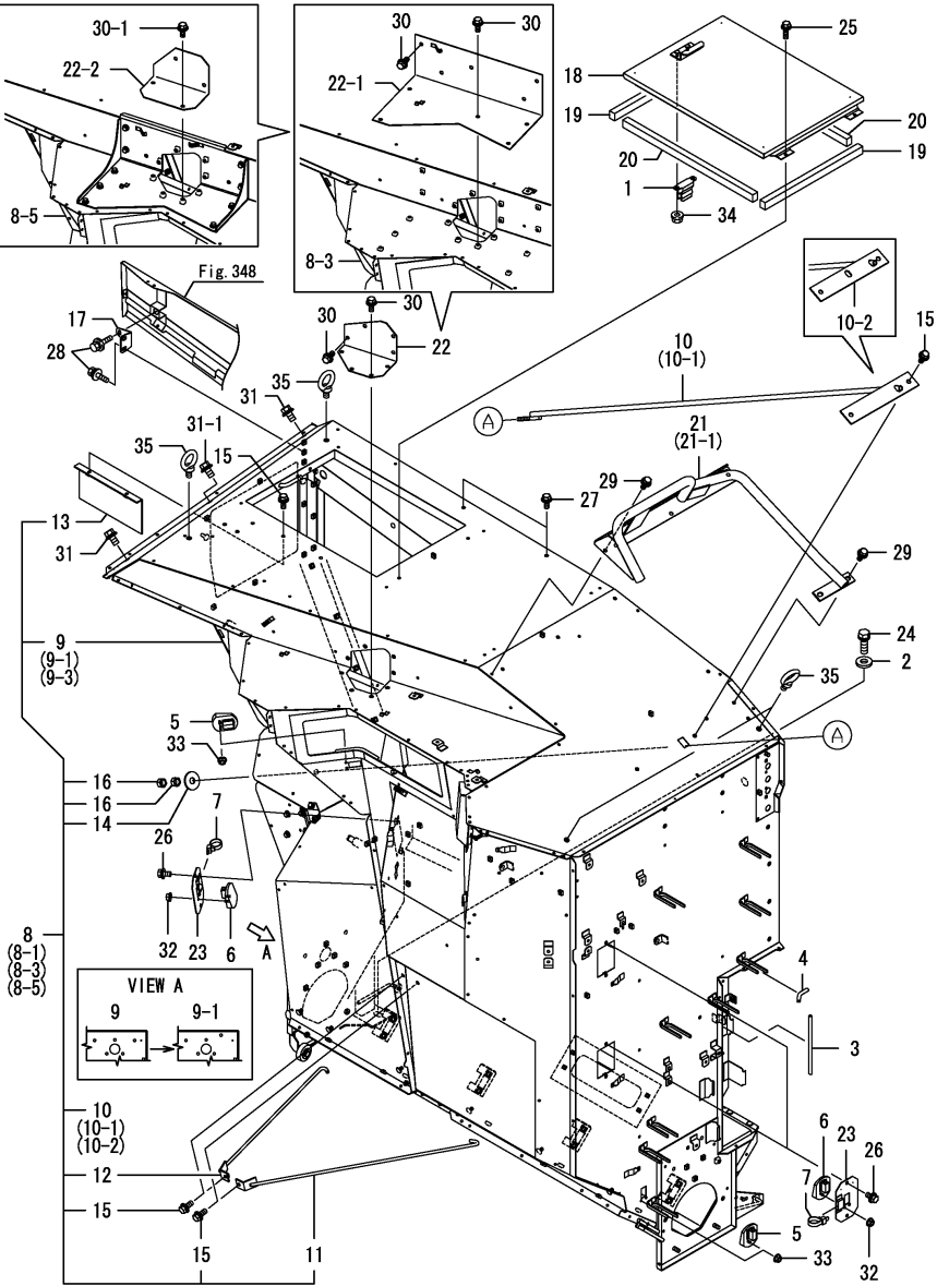
Fig.347. 곡물탱크(1)
