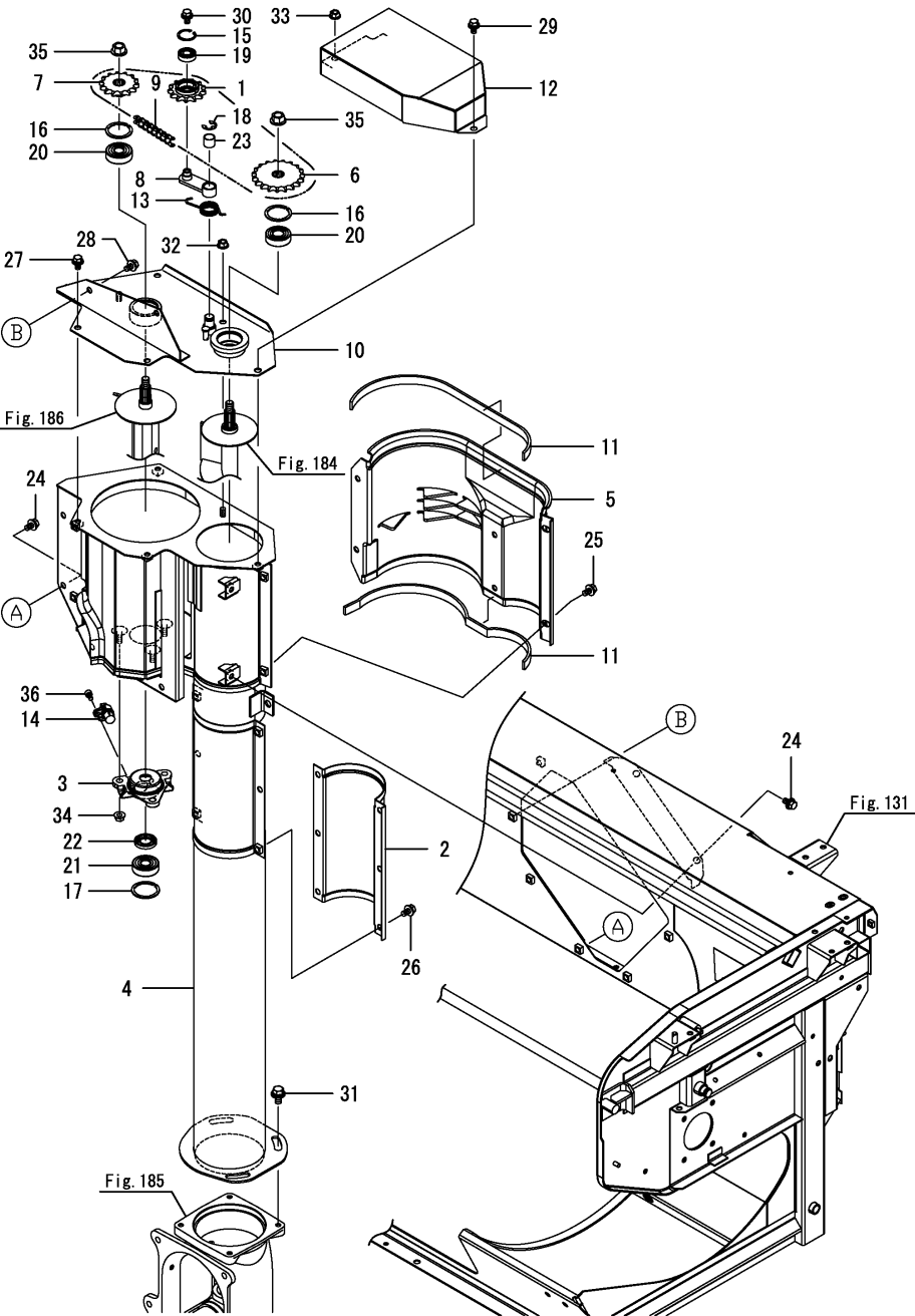
Fig.187. 2번처리통케이스
