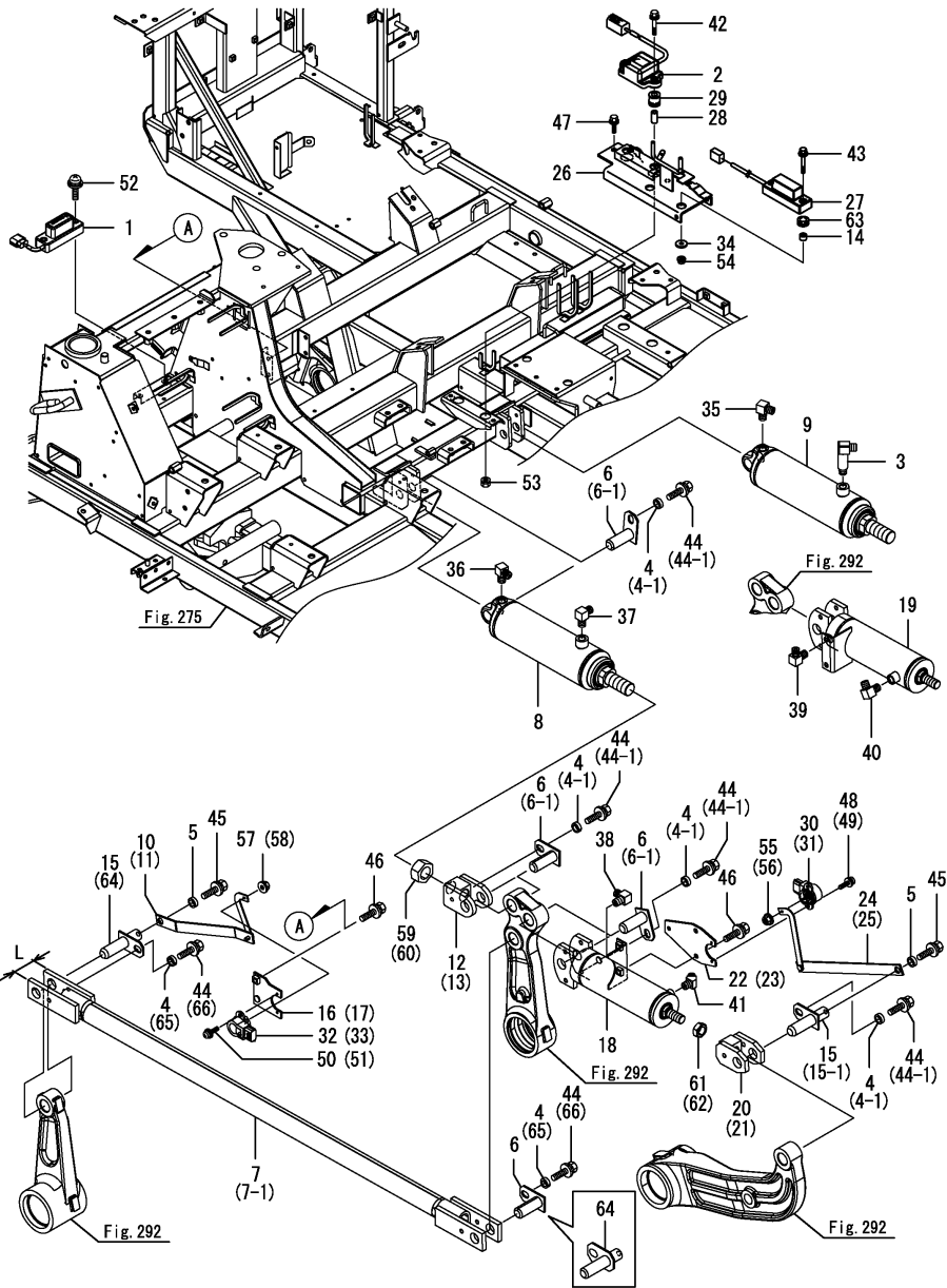
Fig.293. 스윙(2)(피칭 U.F.O.)
