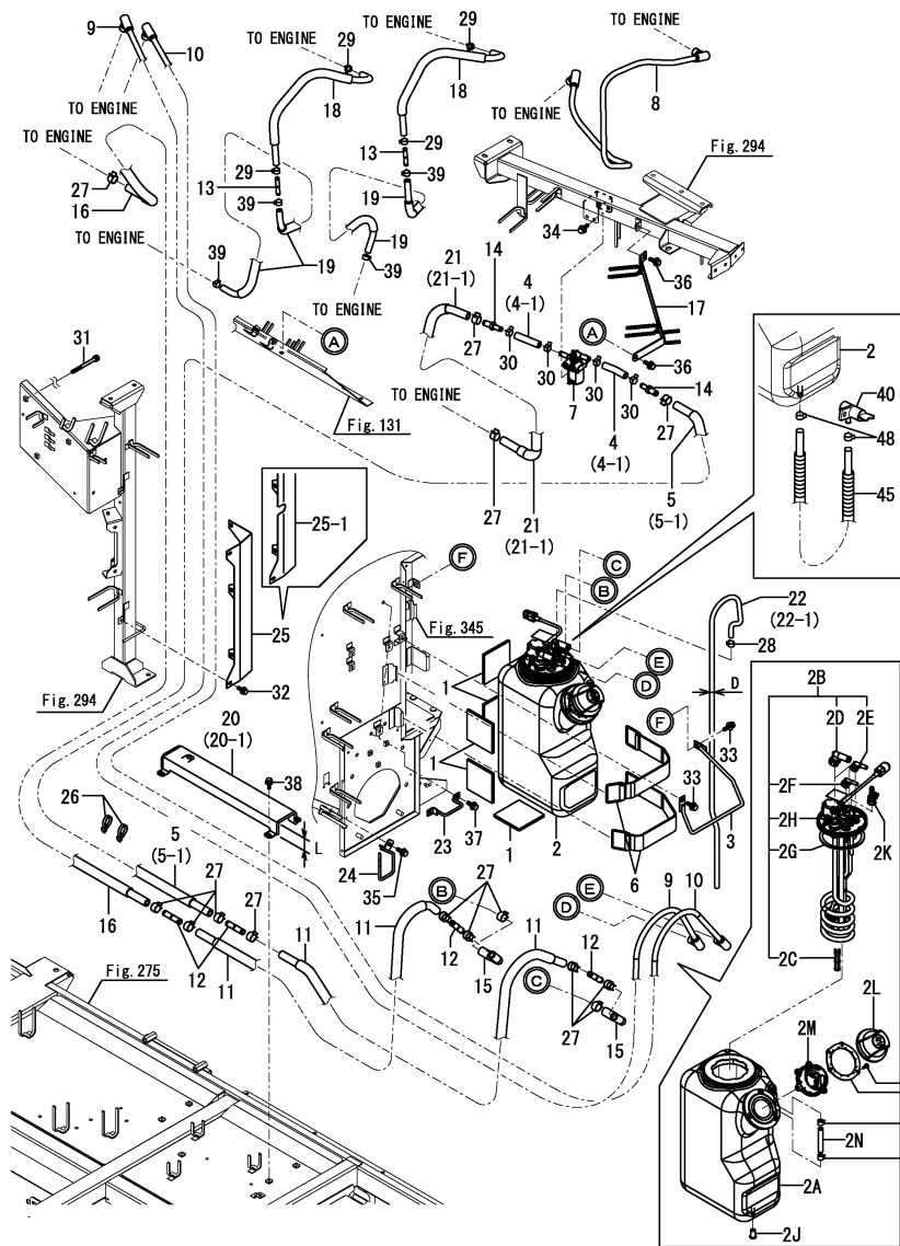
Fig.6. 요소수 탱크
