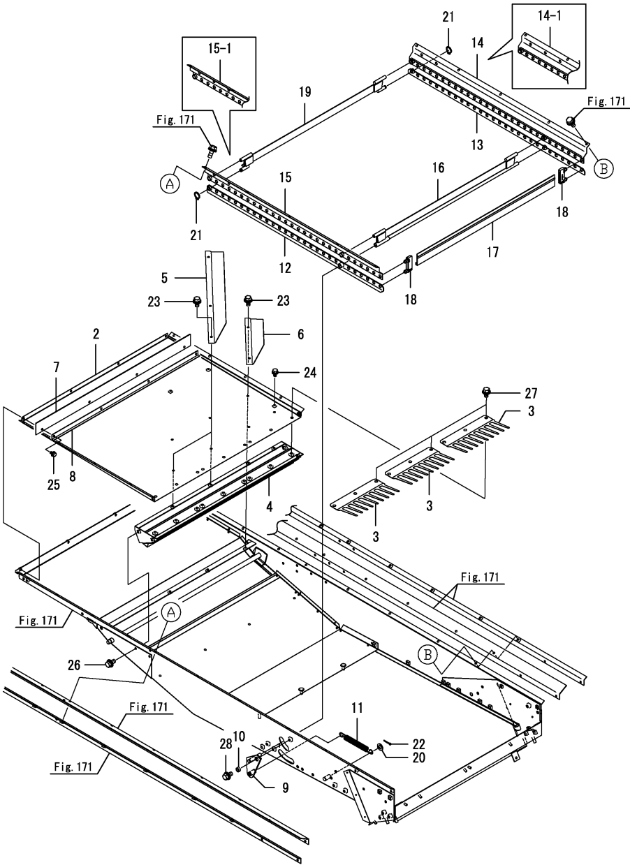
Fig.173. 요동선별프레임(3)
