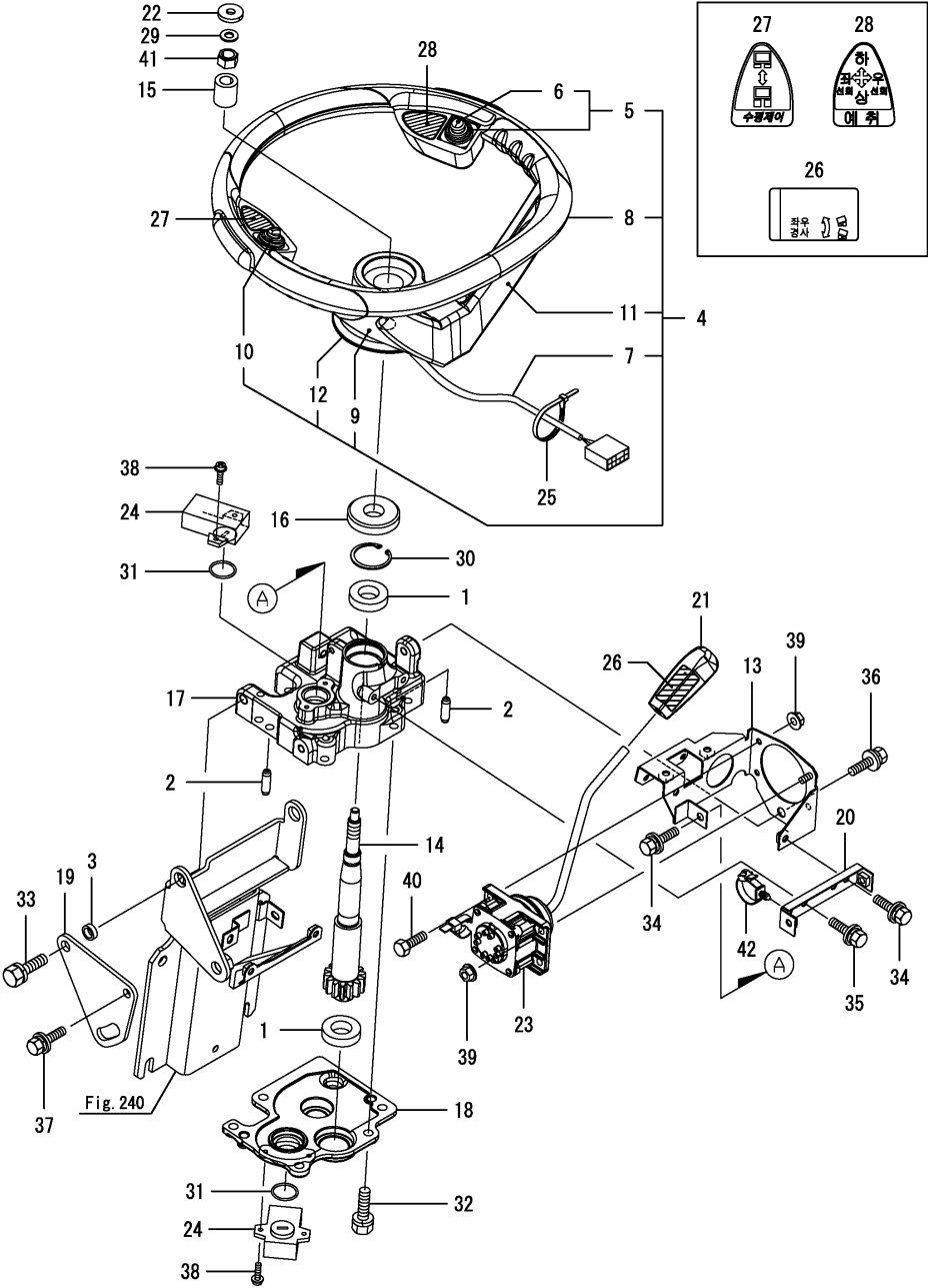
Fig.241. 스티어링(1)
