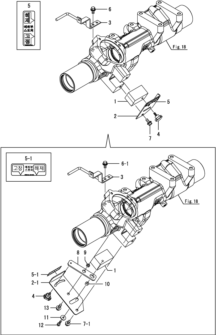
Fig.38. 투입 케이스
