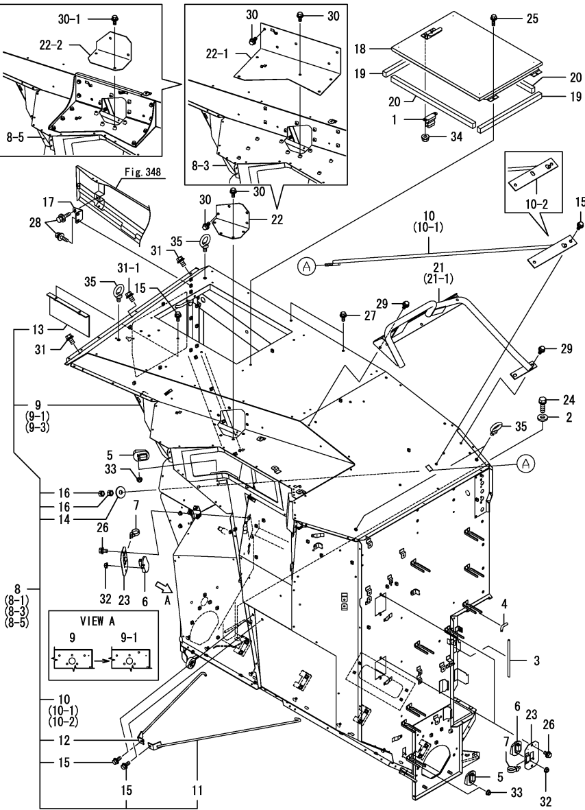
Fig.347. 곡물탱크(1)
