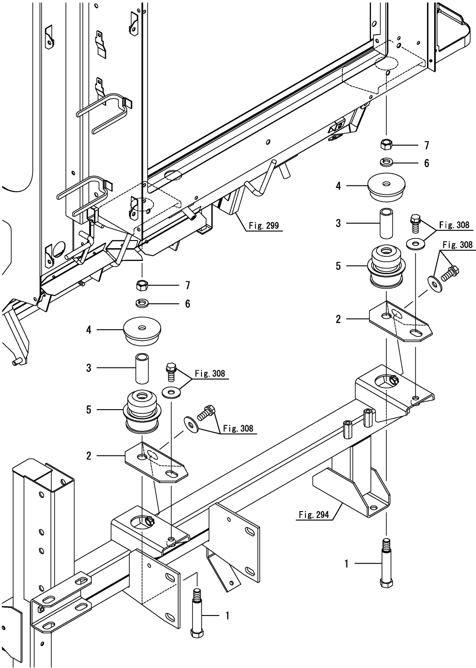
OCNP6-M05021 이동(2) Fig.267. 발판방진(뒤)
