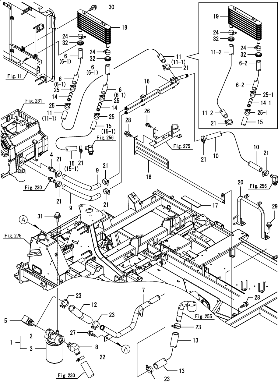
OCNP6-M05021 이동(2) Fig.262. 배관(2)(피칭 U.F.O.)
