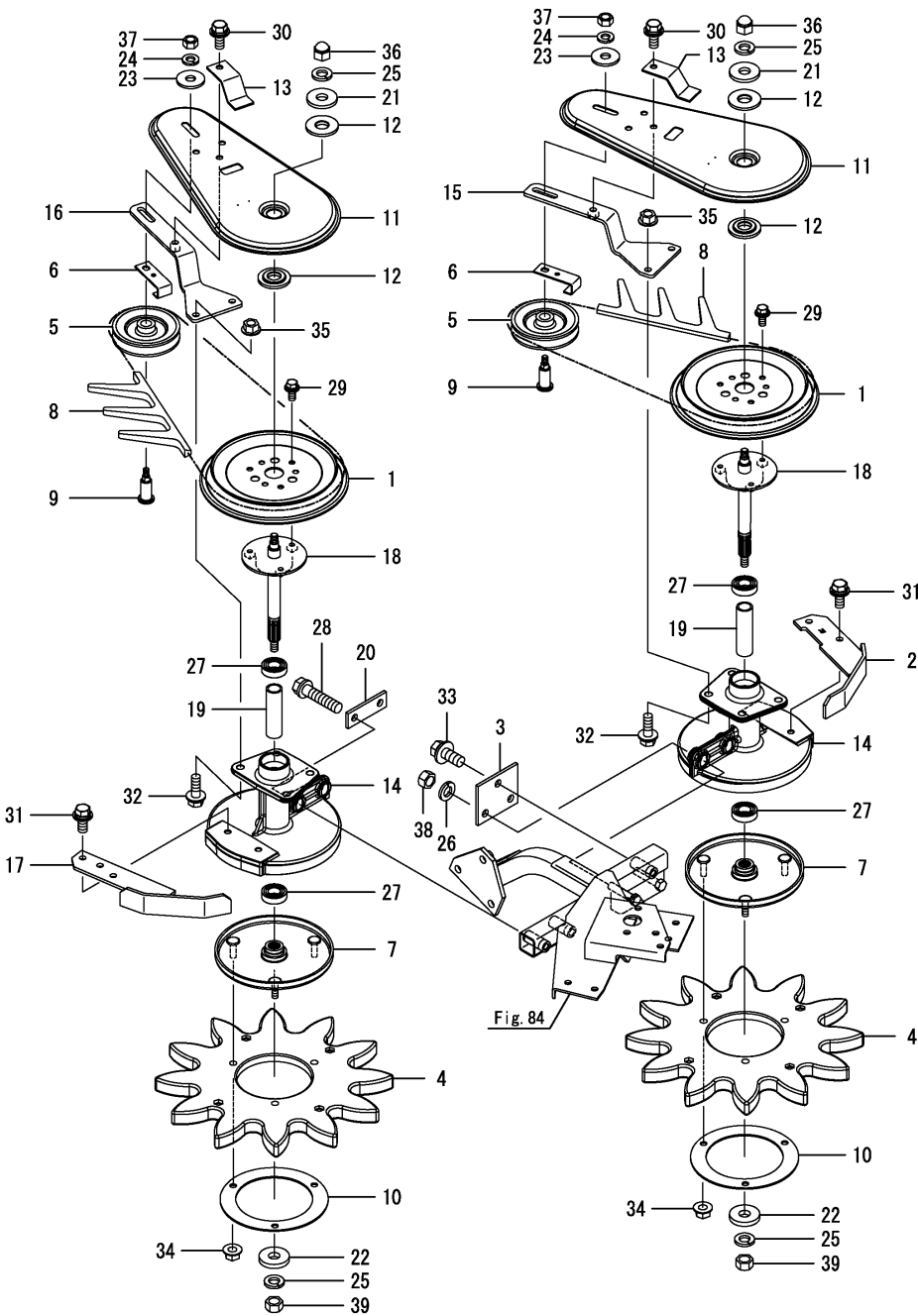
Fig.75. 스타휠(중-우)
