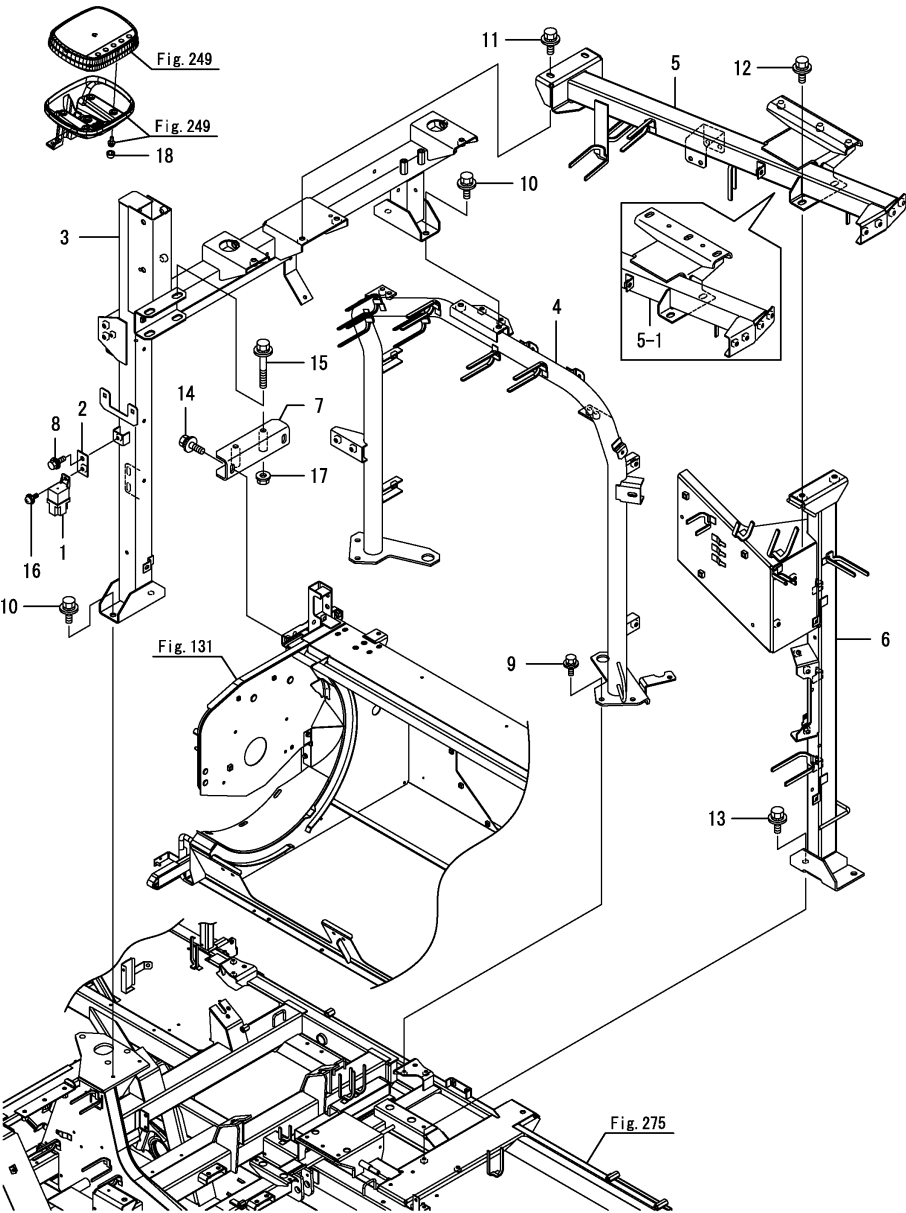
Fig.294. 바닥 프레임
