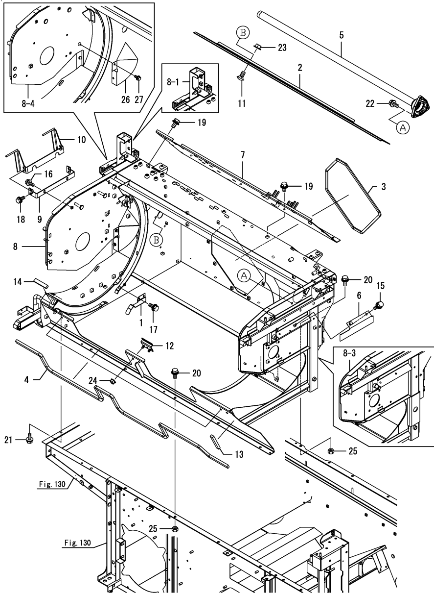
Fig.131. 상부분체(1)
