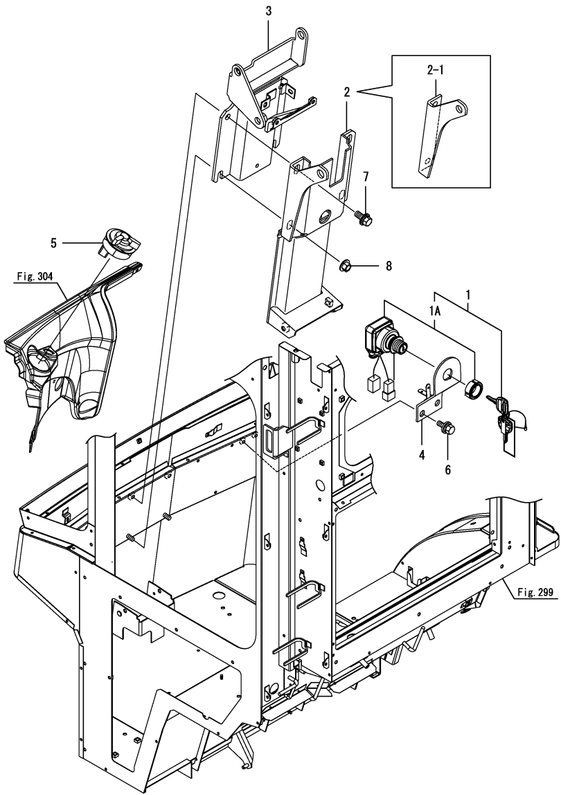
Fig.240. 스티어링칼럼
