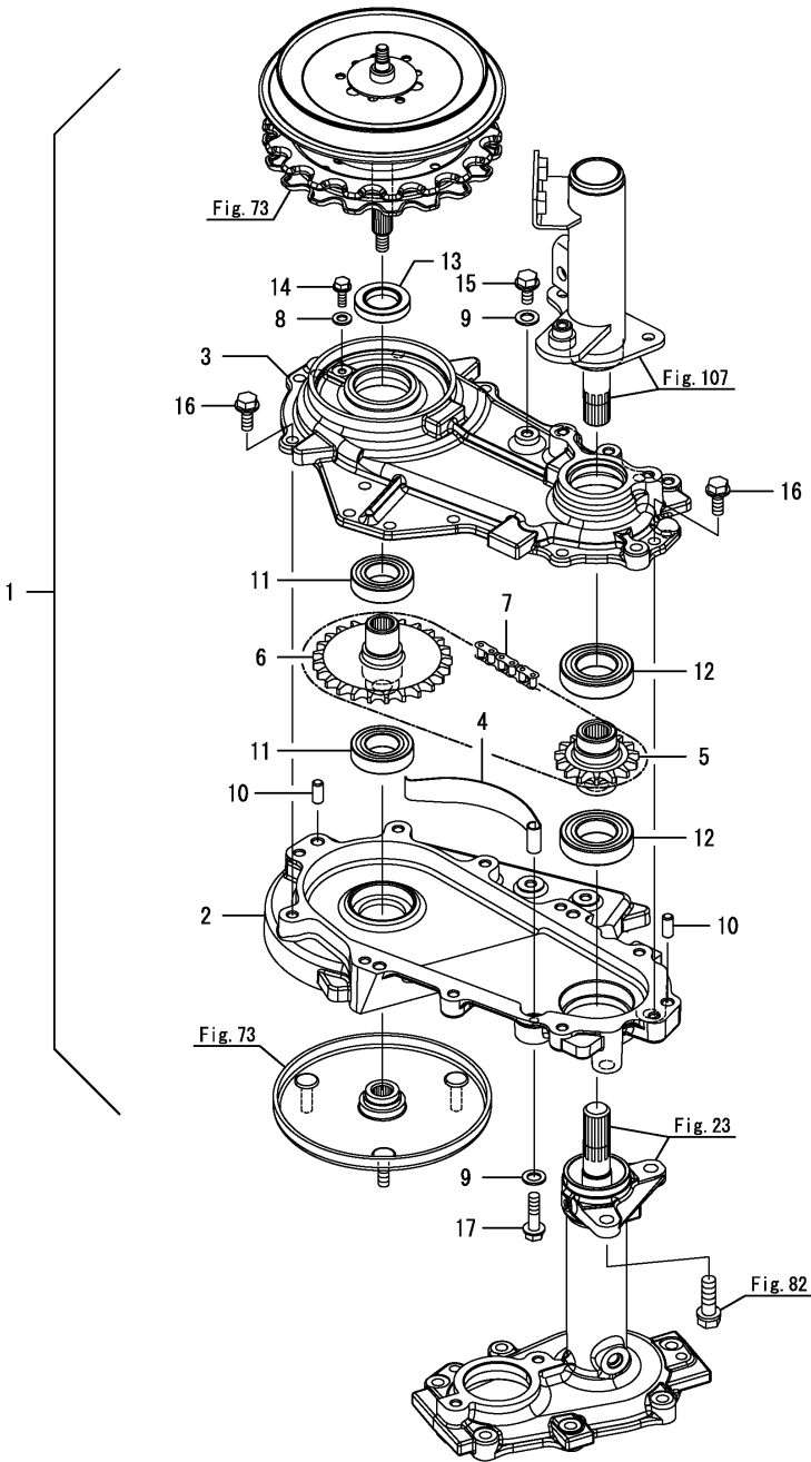
Fig.87. 레이크인 케이스
