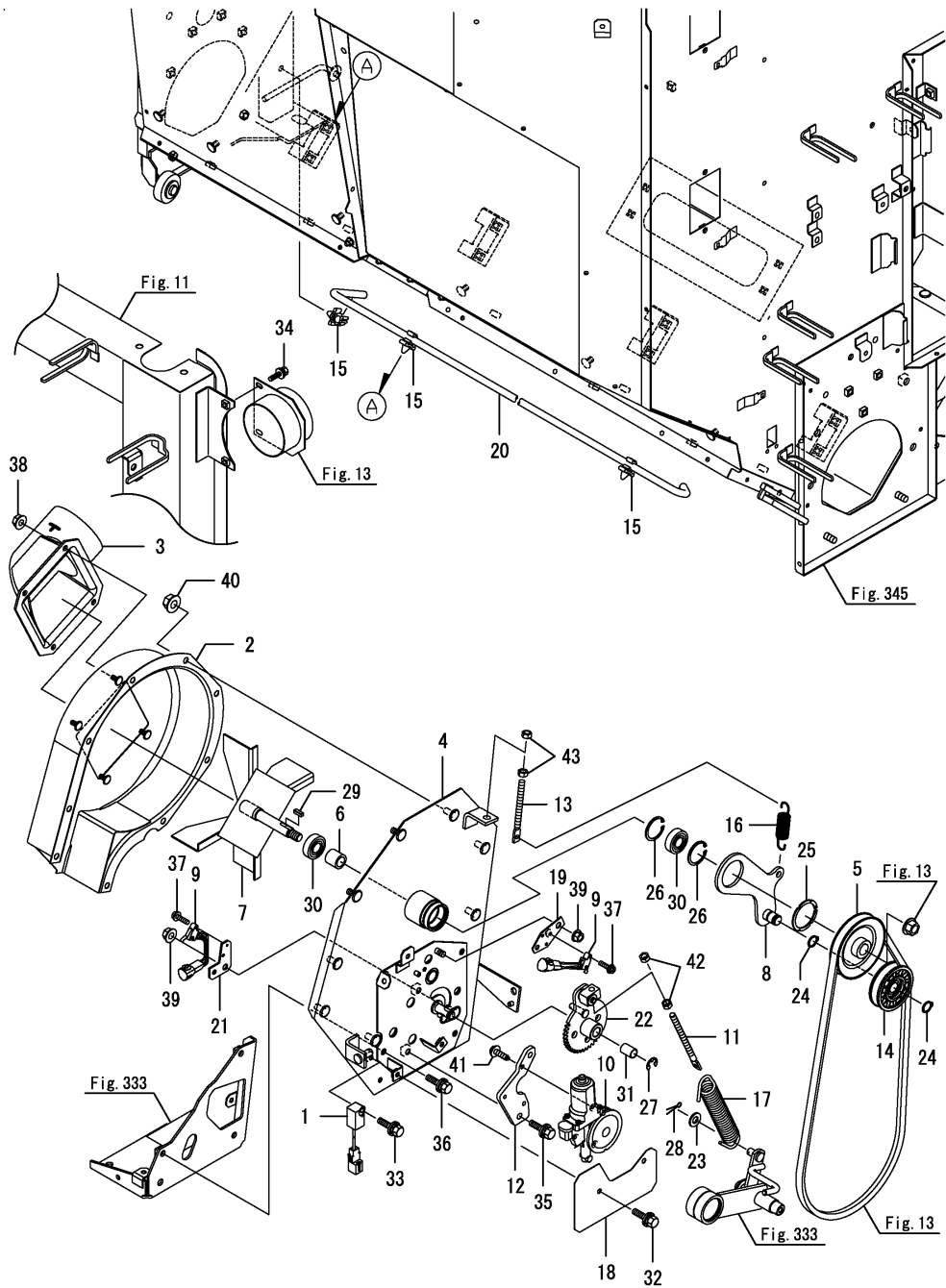
Fig.335. 오거 클러치
