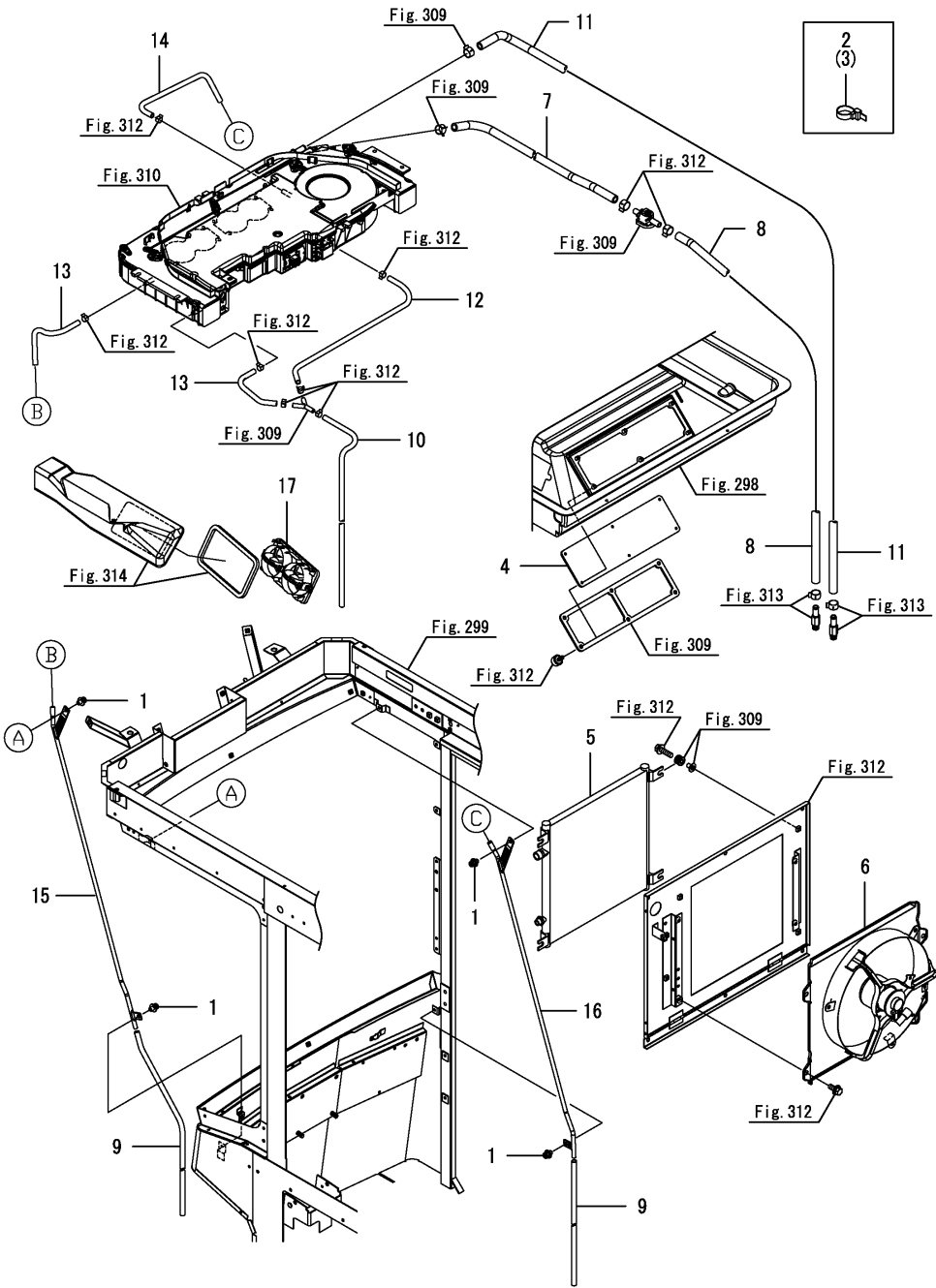
Fig.311. 에어컨(3)
