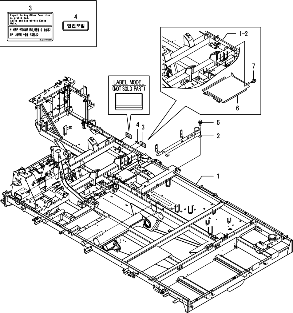
Fig.275. 새시프레임
