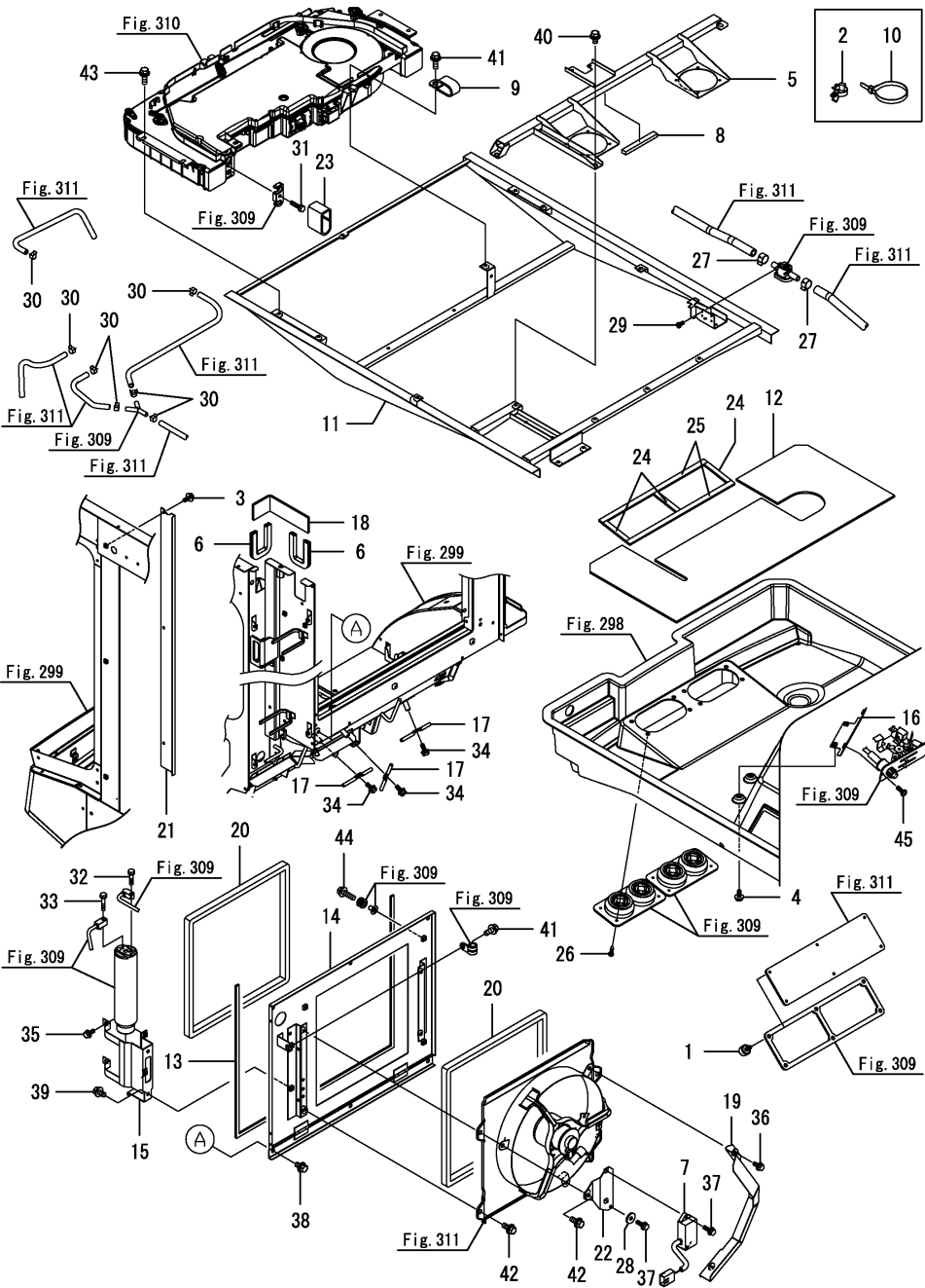
Fig.312. 에어컨취부(1)
