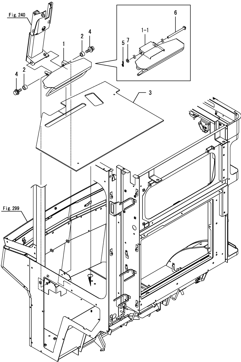
Fig.265. 단(1)
