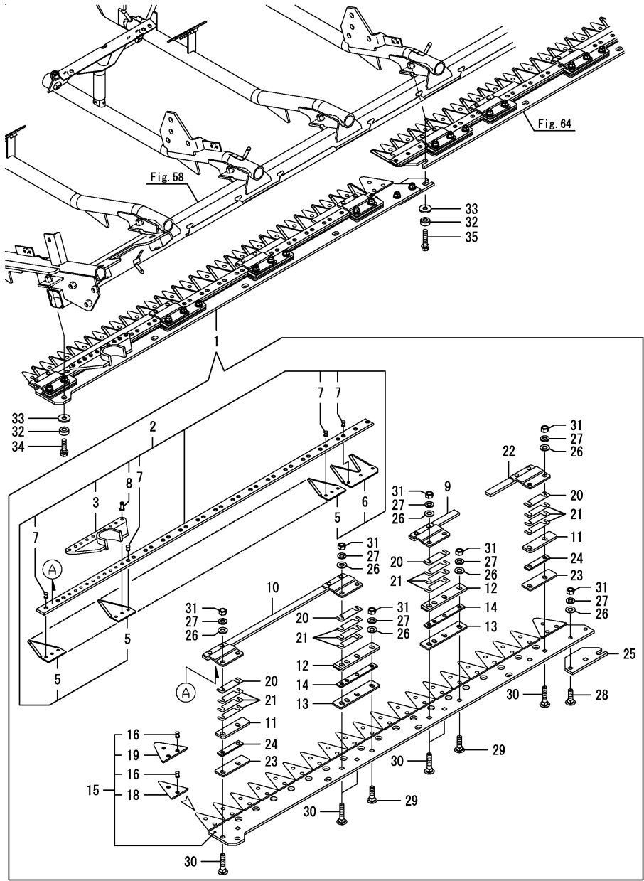
Fig.63. 예취날(좌)
