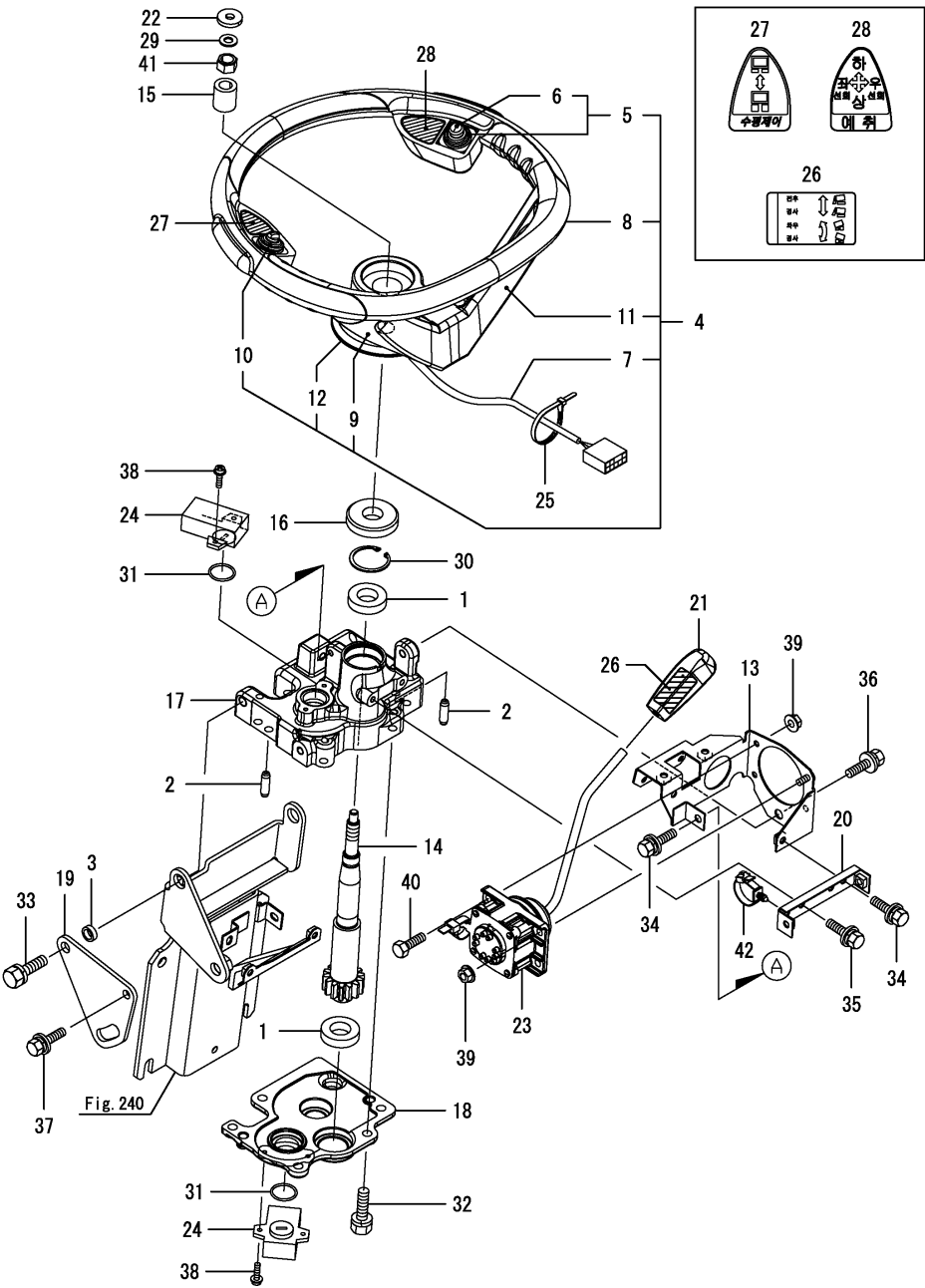
OCNP6-M05021 이동(2) Fig.243. 스티어링(1)(피칭 U.F.O.)
