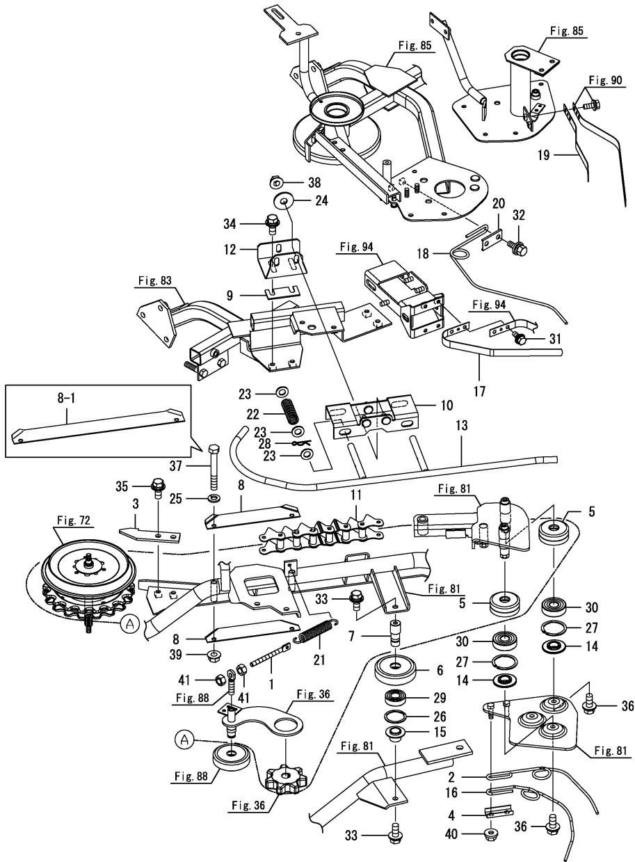
OCNP6-M05021 수확(2) Fig.92. 하단 이송 가이드(왼쪽)
