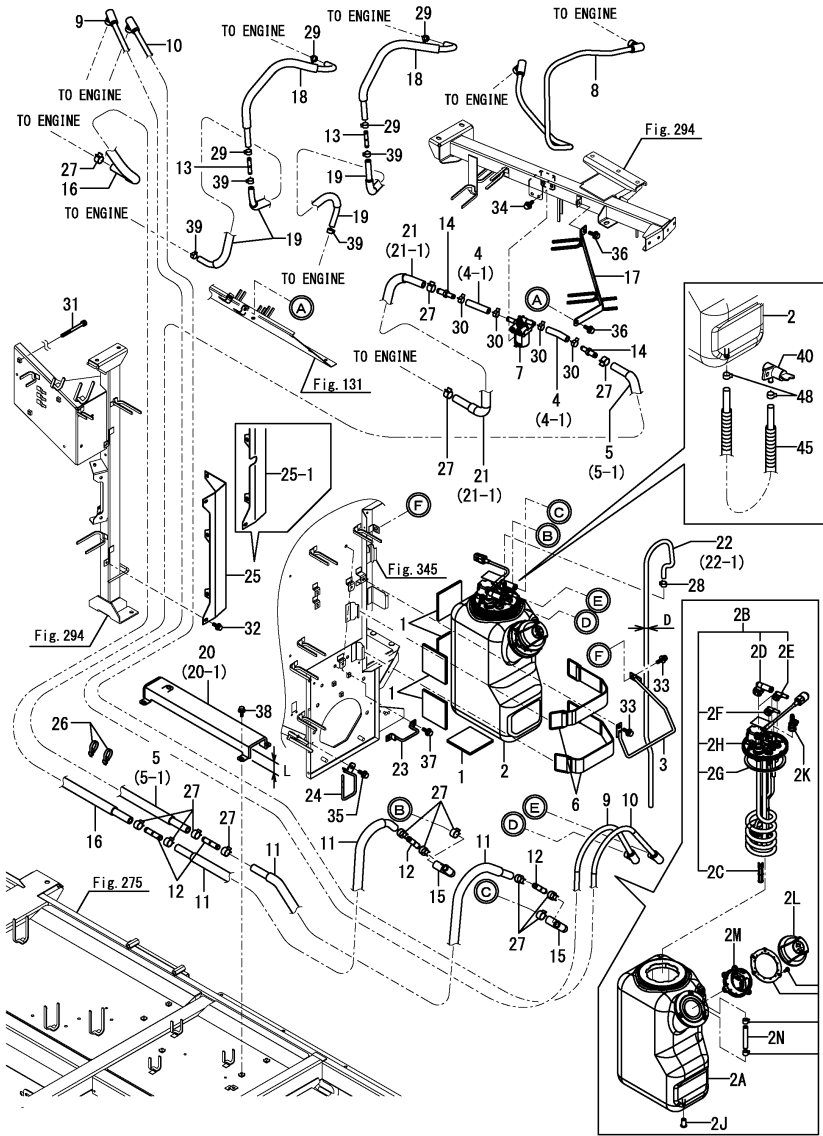
Fig.6. 요소수 탱크
