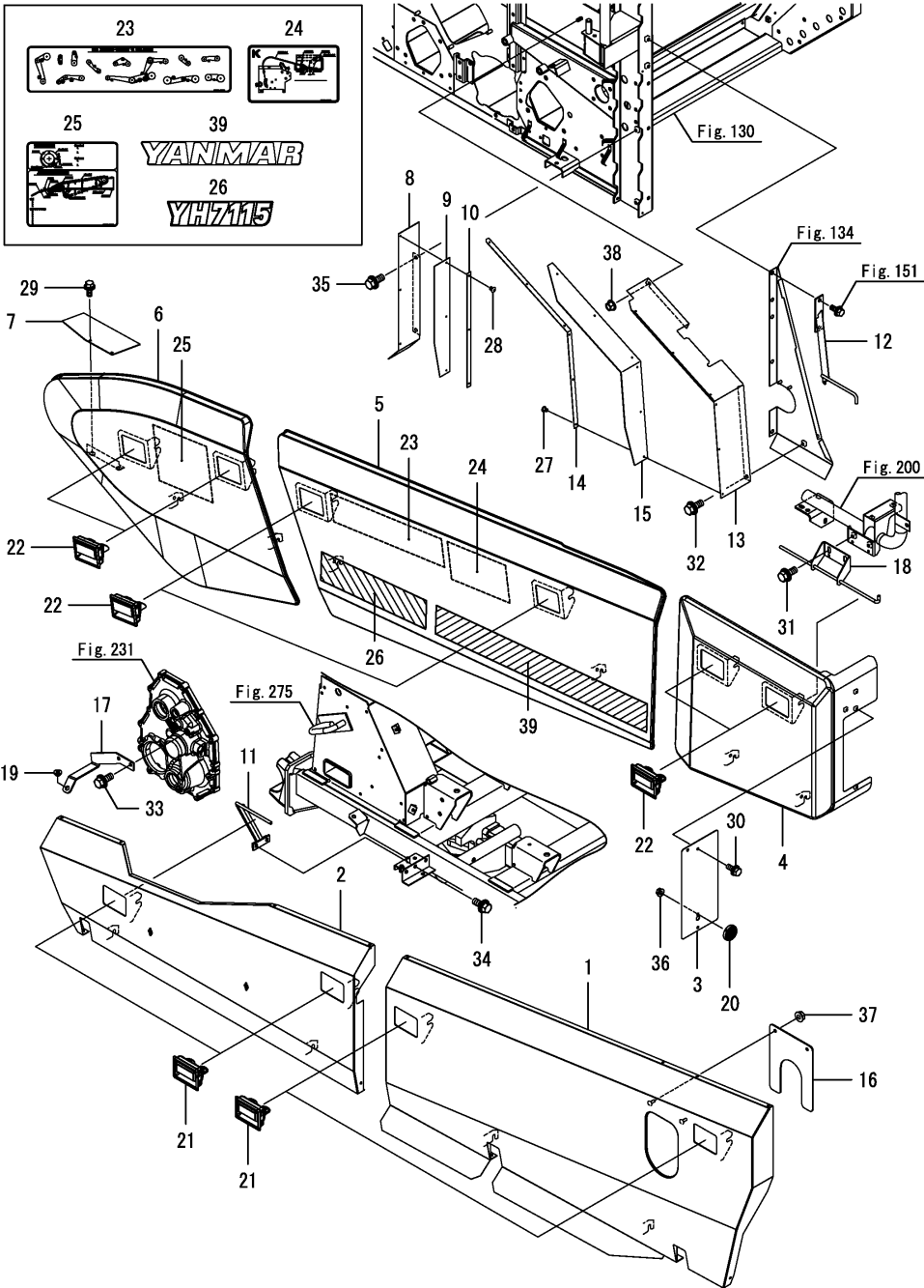
Fig.153. 탈곡통커버(앞)(사이드)
