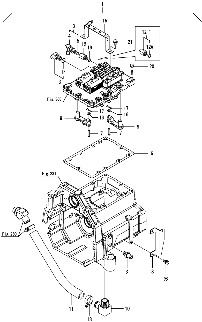
Fig.230. 카운터케이스(1)
