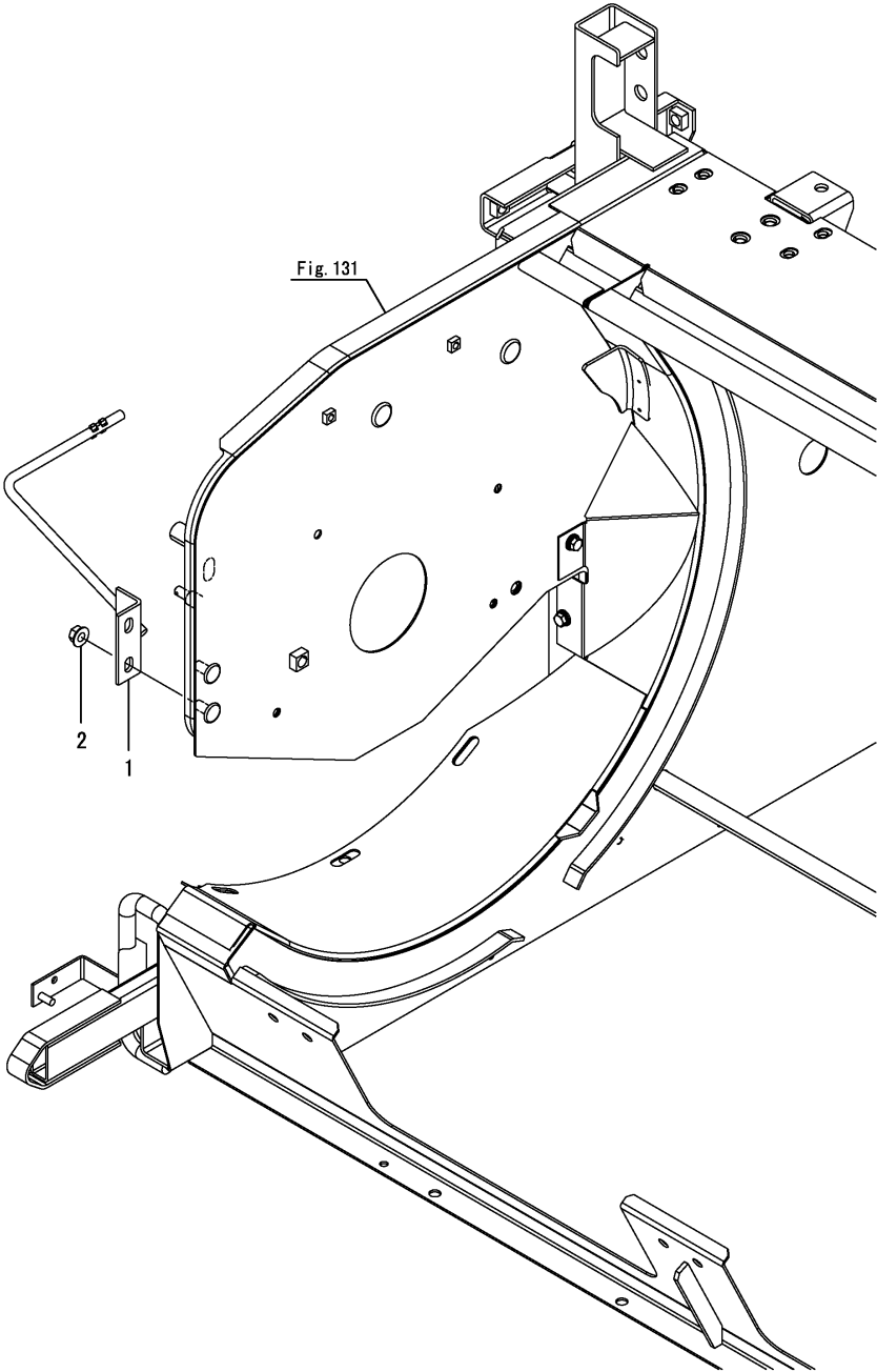
Fig.157. 탈곡통커버(앞)
