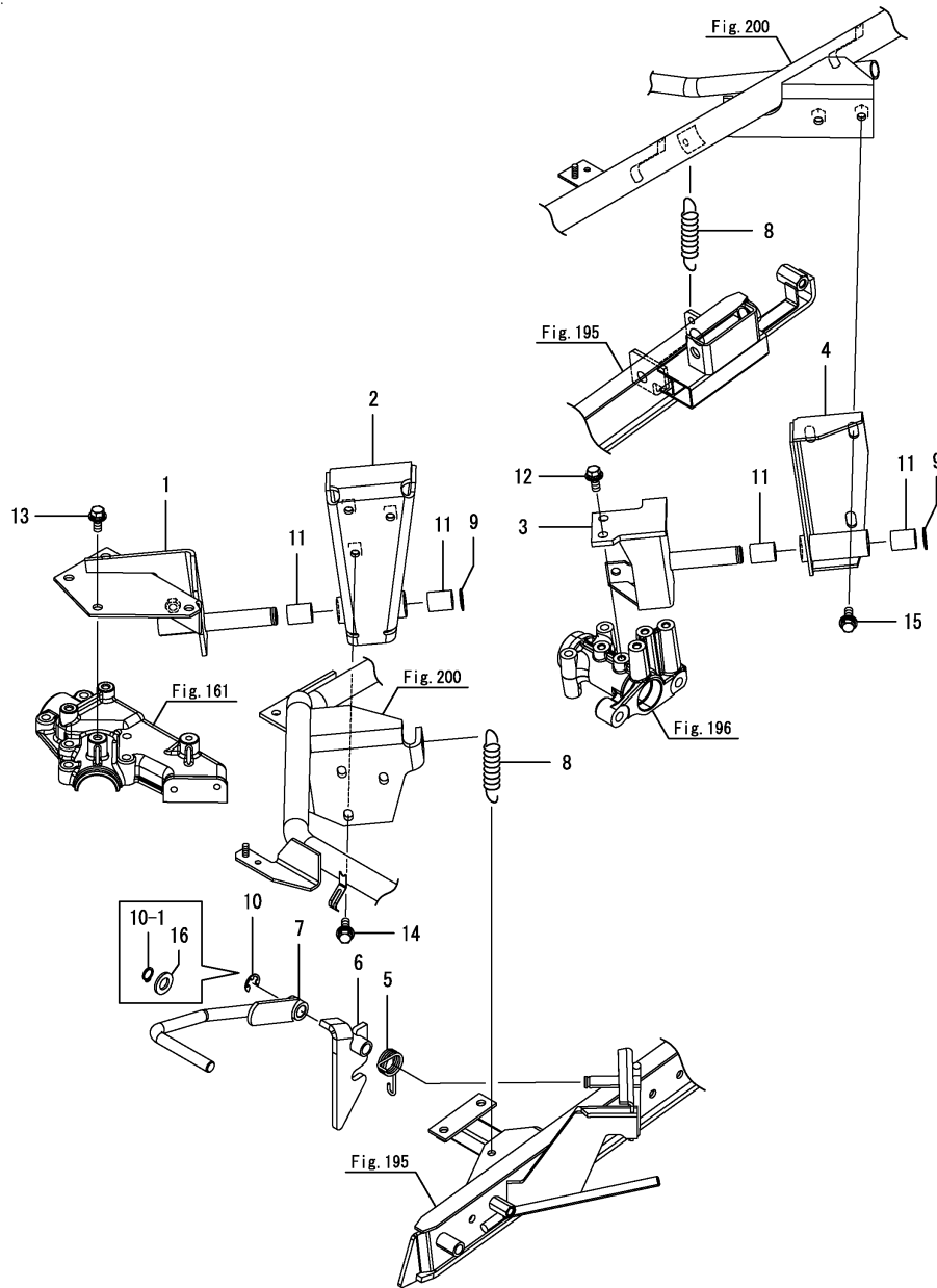
Fig.202. 짚배출오픈
