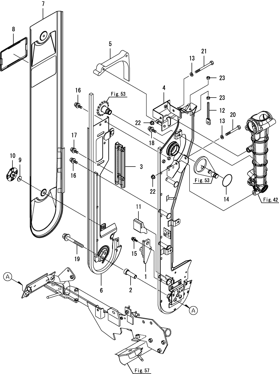
Fig.48. 픽업 케이스(오른쪽)
