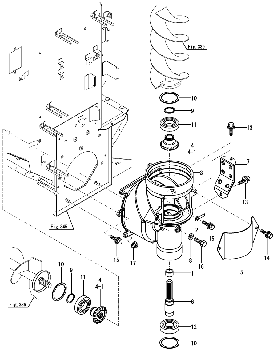
Fig.337. 하부컨베이어연결
