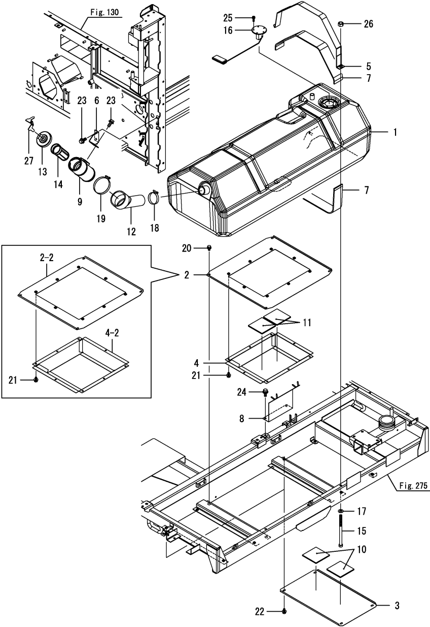
Fig.4. 연료탱크(1)
