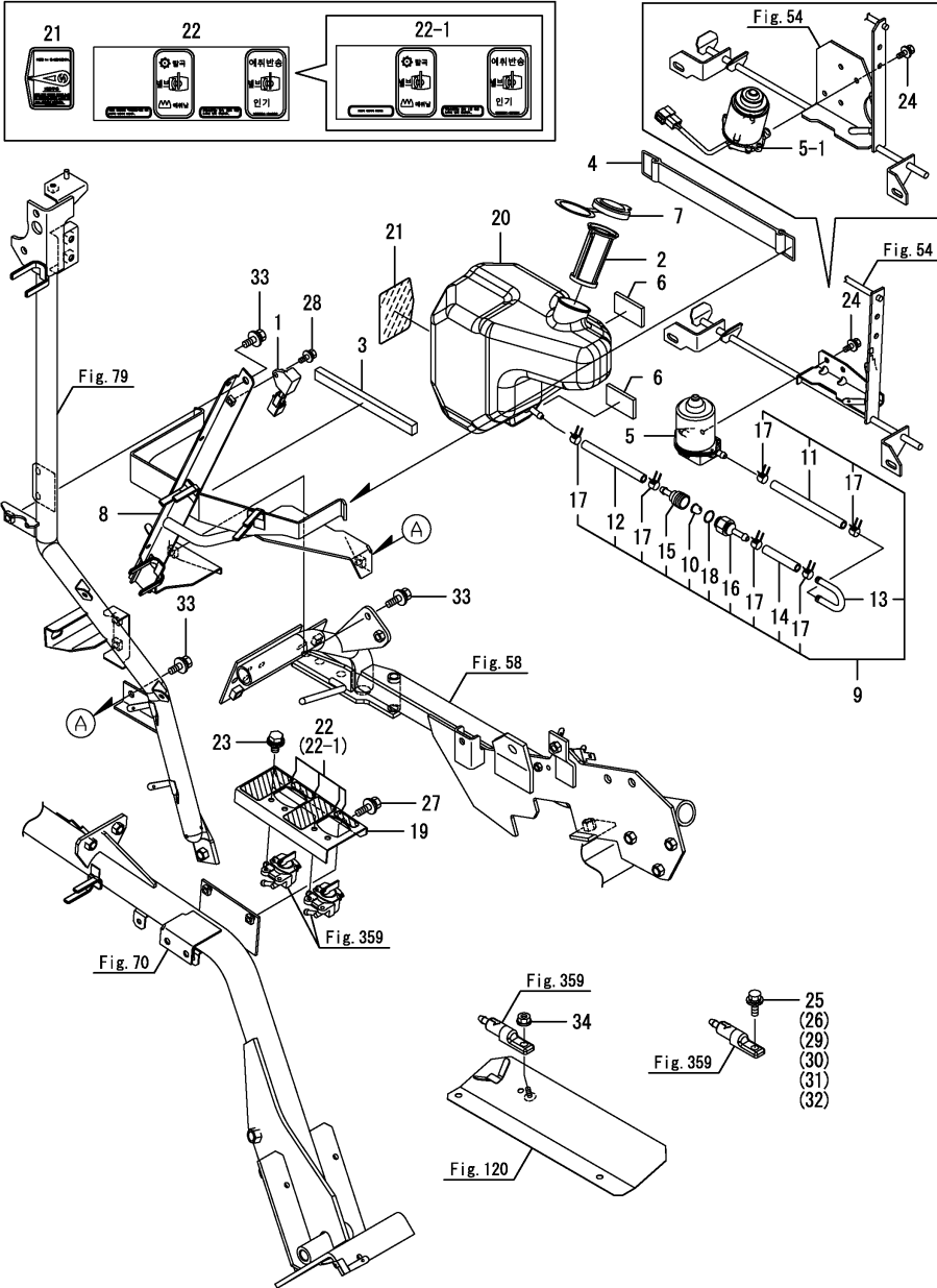
Fig.358. 주유장치(1)
