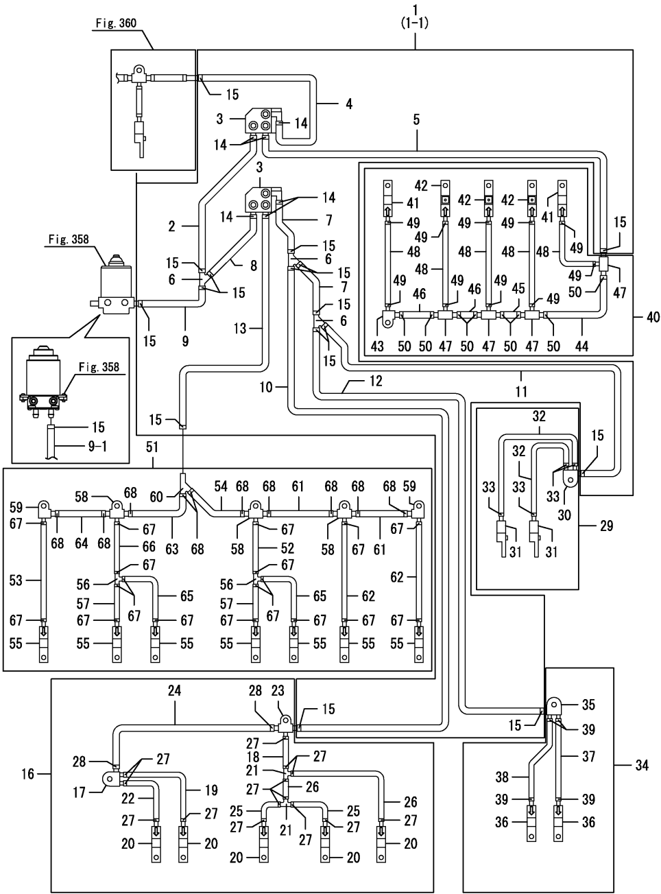
Fig.359. 주유장치(2)
