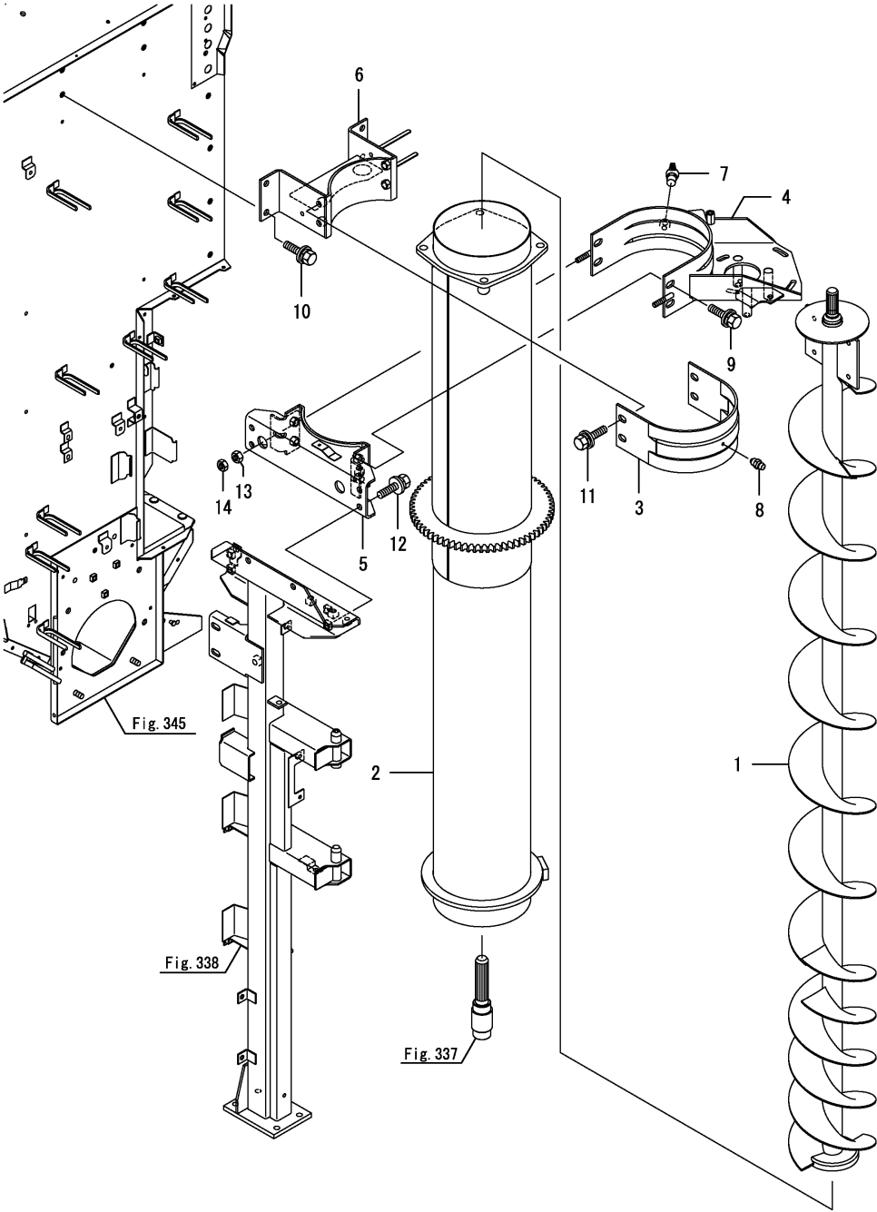
Fig.339. 수직 컨베이어
