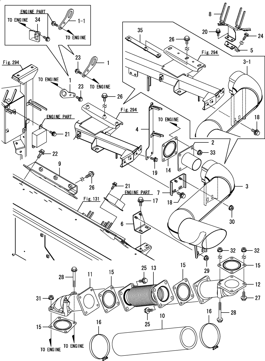
Fig.10. 머플러
