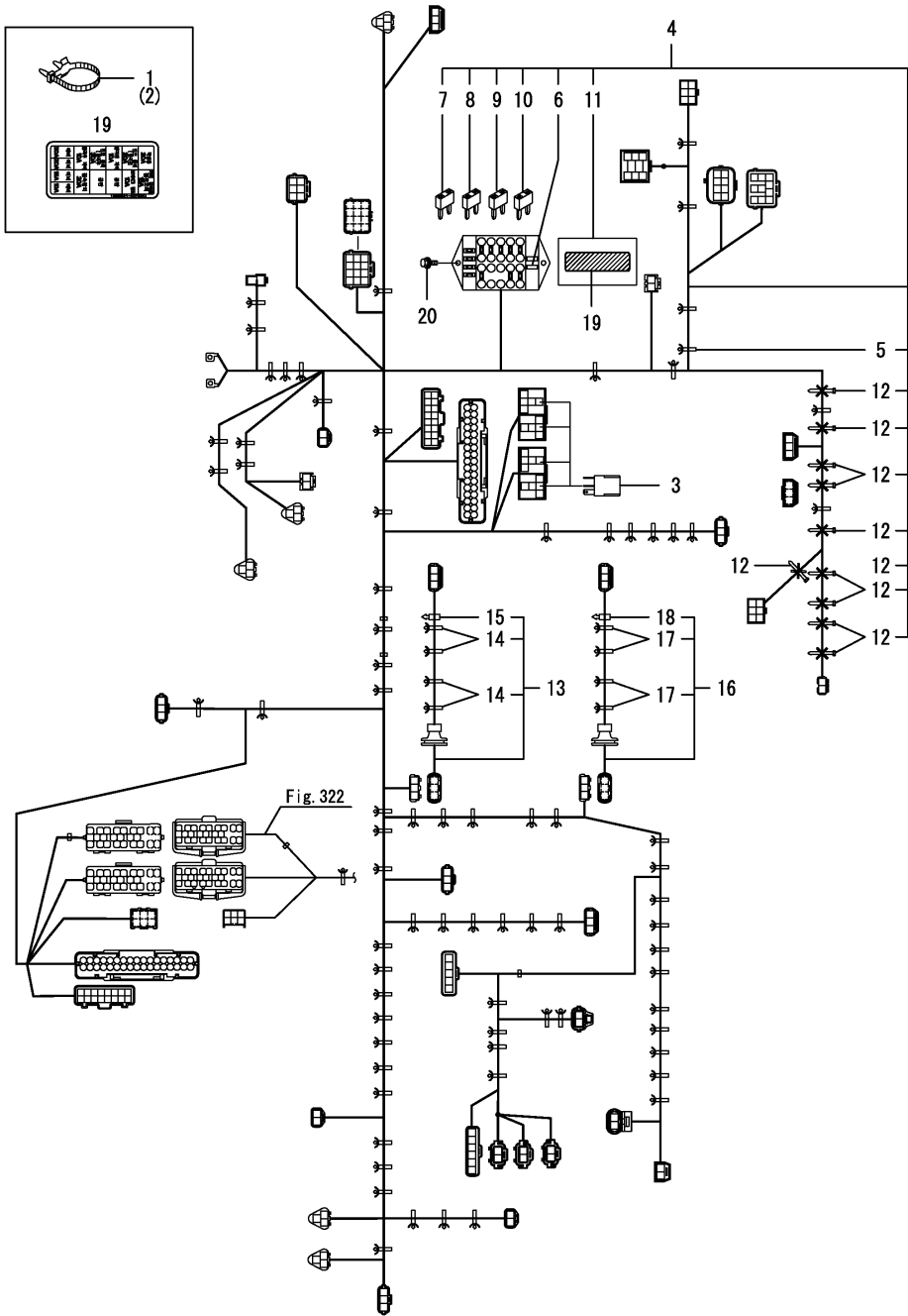
Fig.329. 배선(탈곡)
