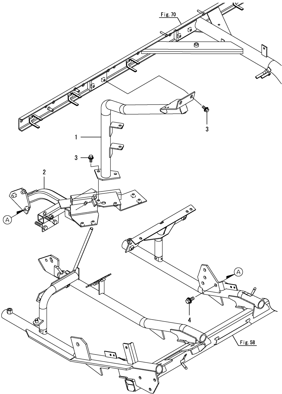
Fig.83. 끌어모음프레임(중-좌)
