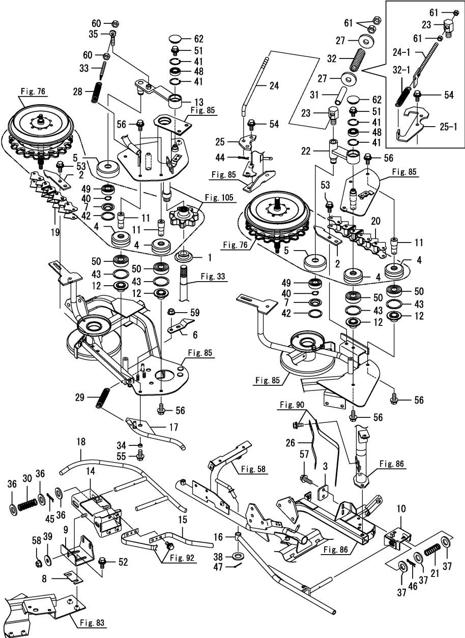
OCNP6-M05021 수확(2) Fig.94. 하부반송가이드(중-우)
