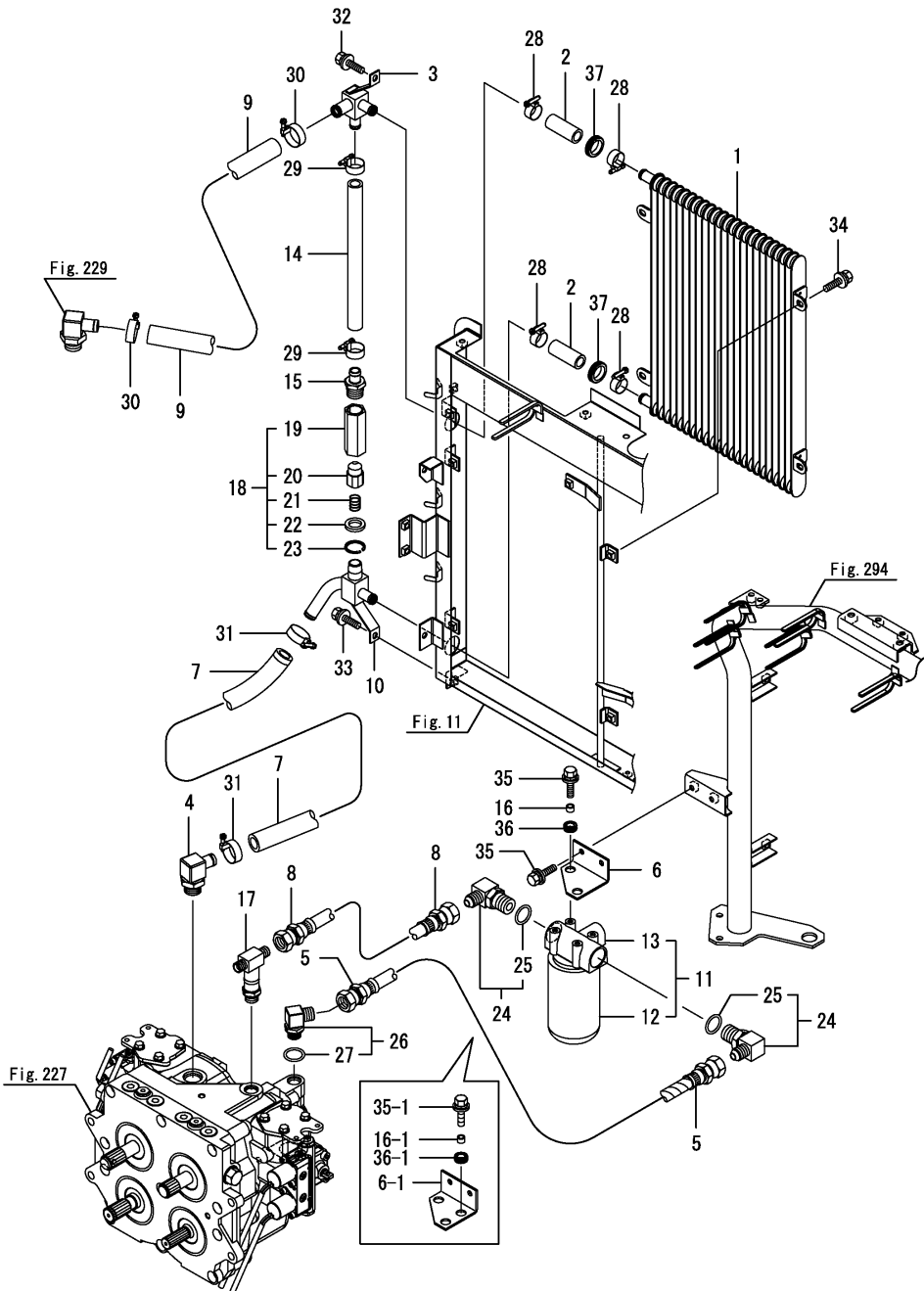
OCNP6-M05021 이동(2) Fig.258. 배관(H.S.T.)
