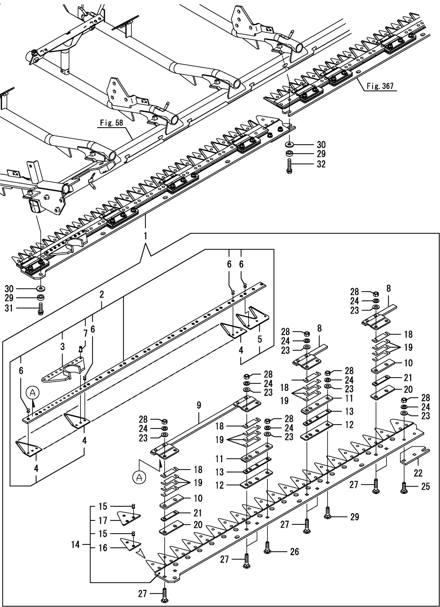
OCNP6-M05021 수확(1) Fig.366. (63A)수확 에지(좌측)
