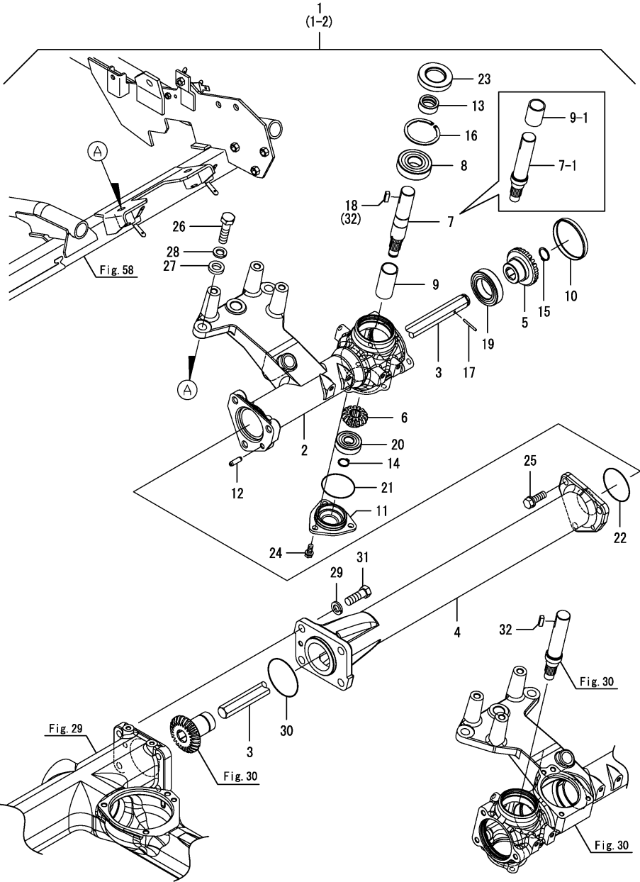
Fig.34. 7조구동케이스(7)
