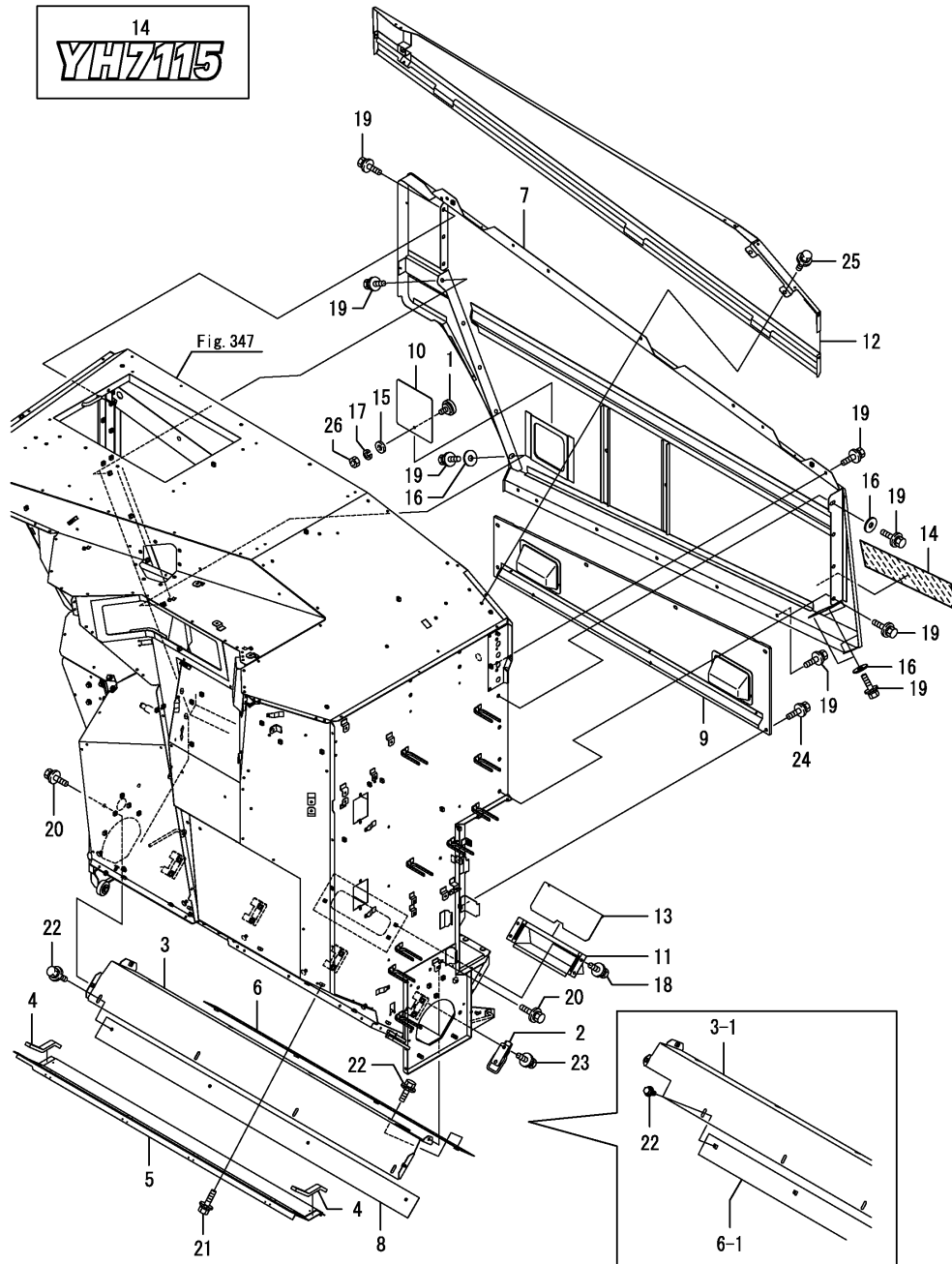
Fig.348. 곡물탱크(2)
