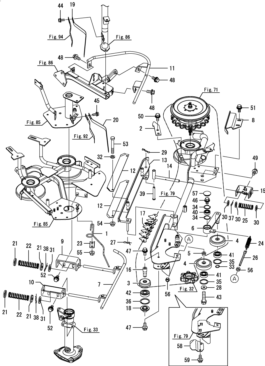
Fig.90. 하단 이송 가이드(오른쪽)
