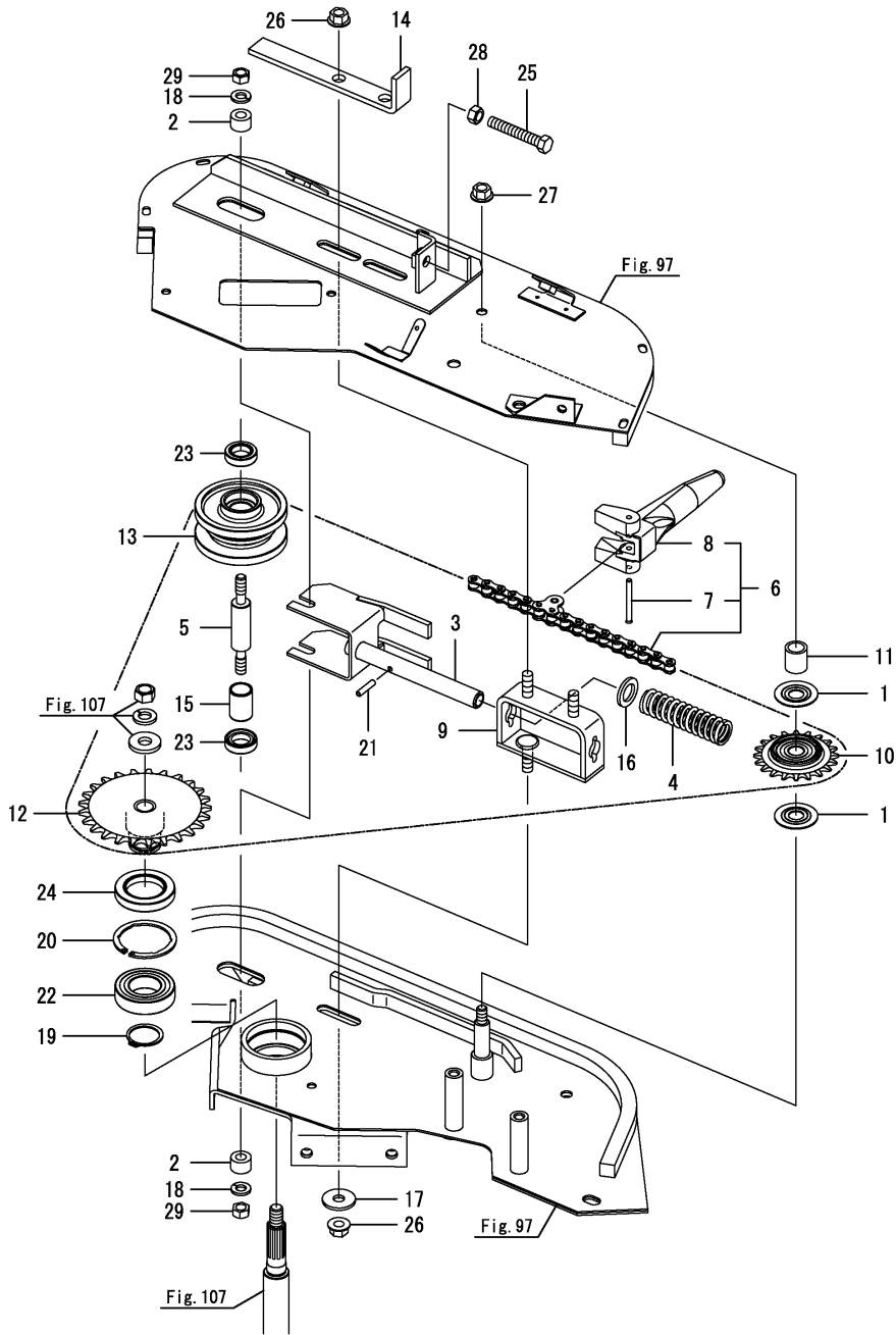
Fig.104. 상반송롤러(중)
