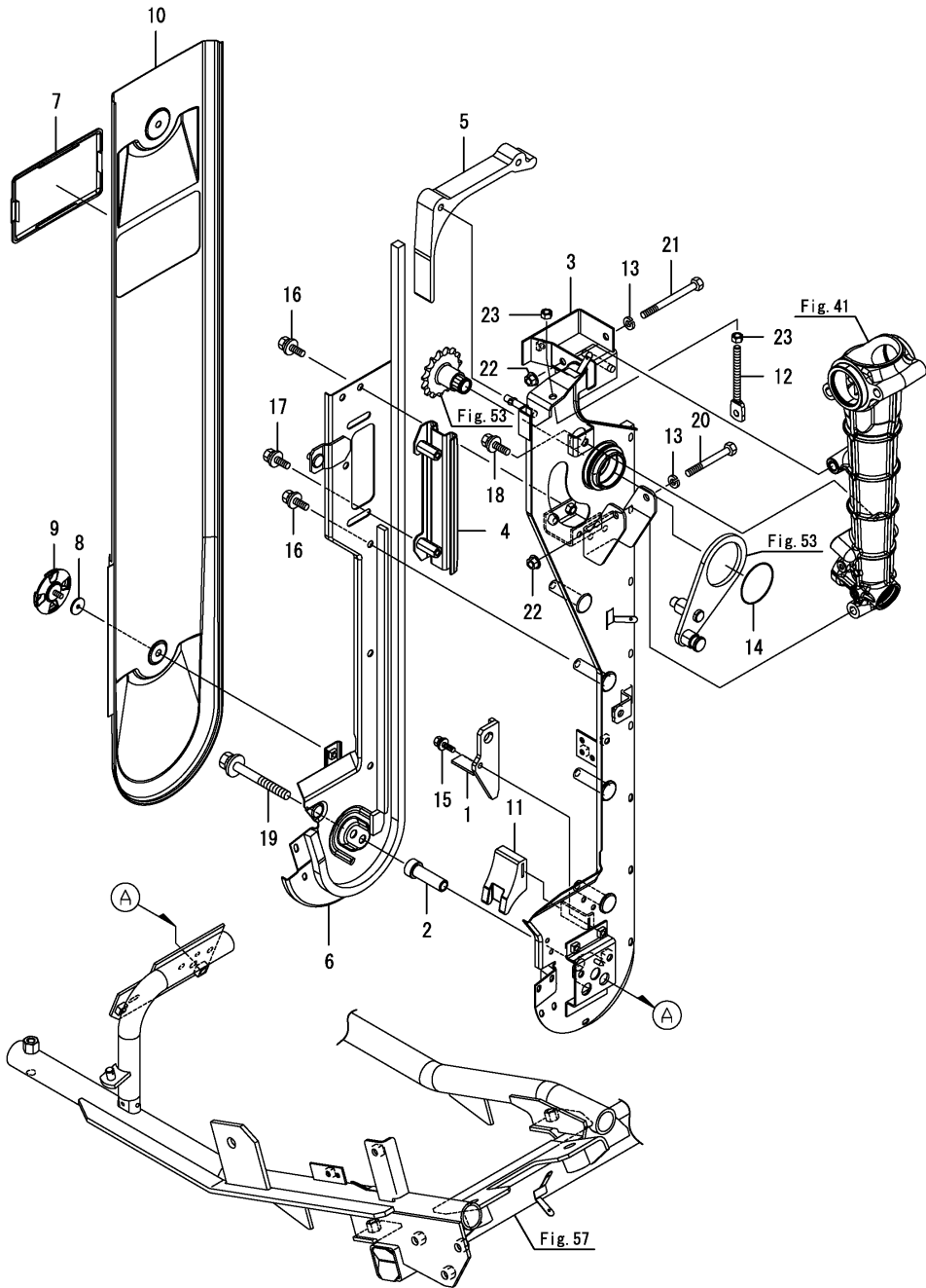
Fig.49. 픽업 케이스(왼쪽)
