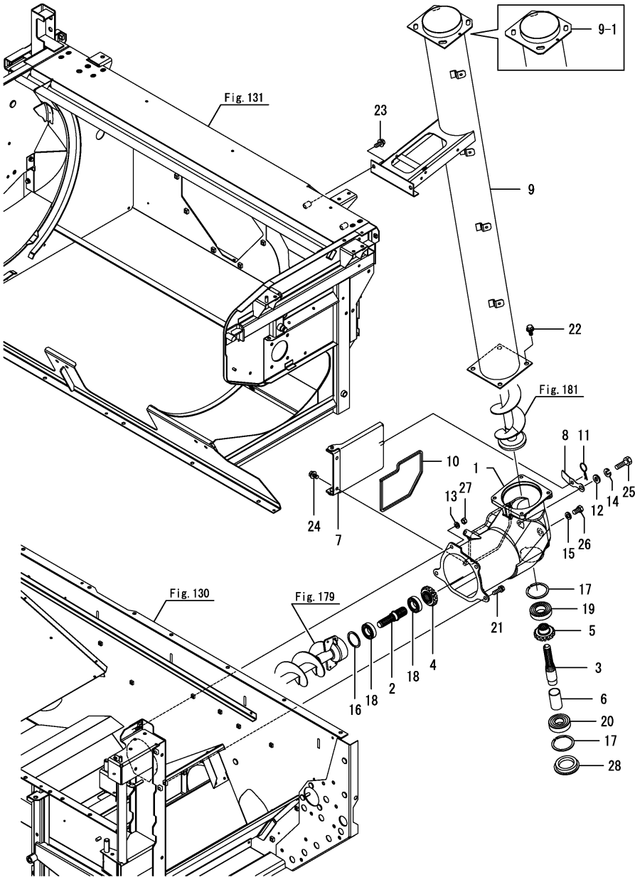
Fig.180. 컨베이어케이스
