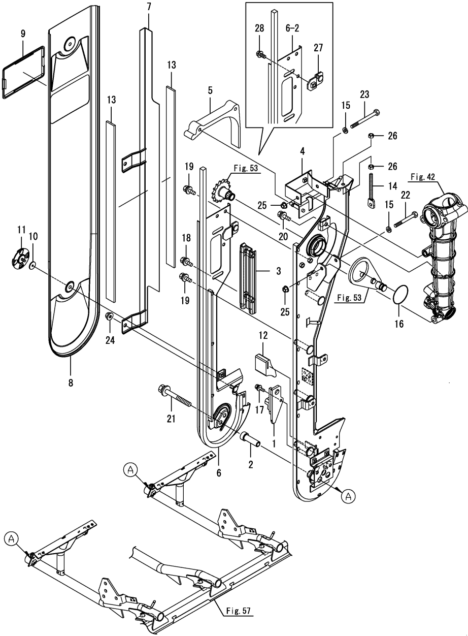
Fig.50. 픽업 케이스(중앙)(1)
