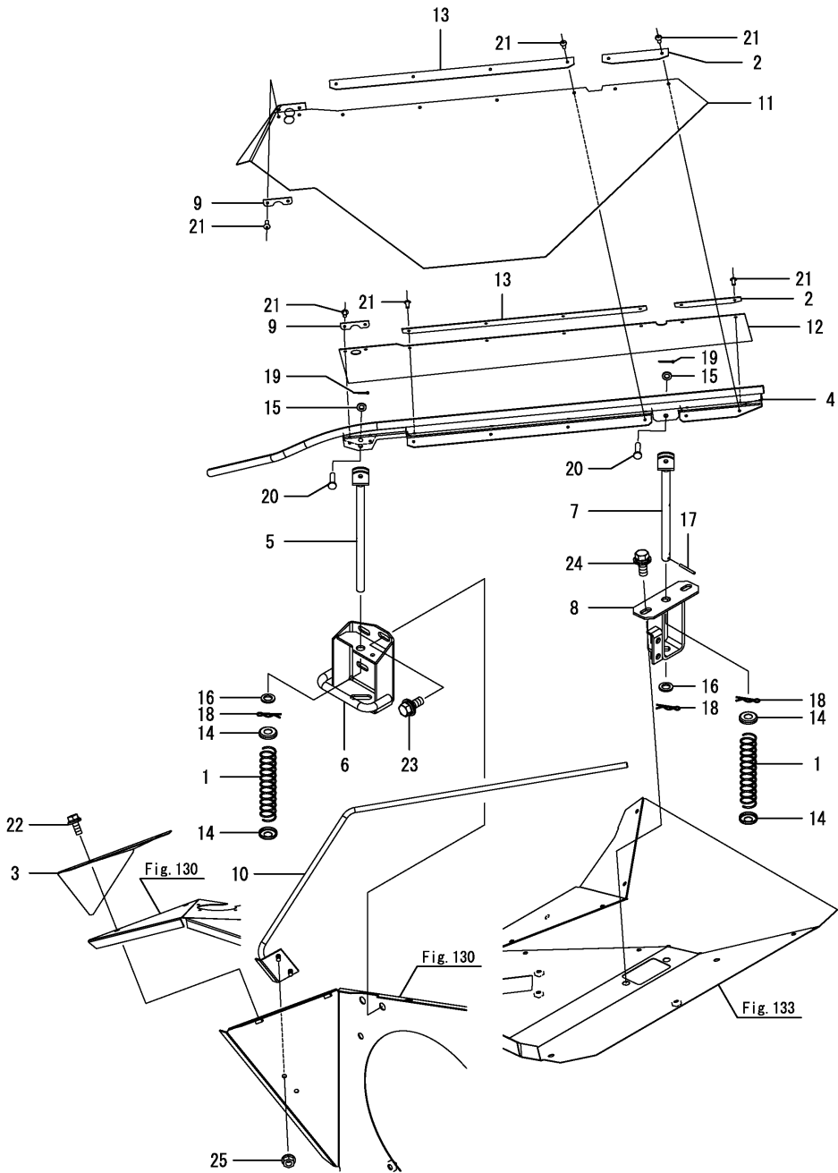
OCNP6-M05021 탈곡(2) Fig.197. 짚배출잡이
