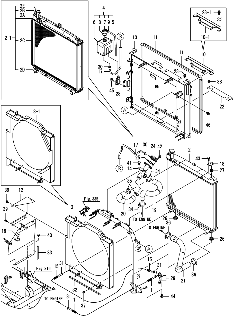
Fig.11. 라디에이터
