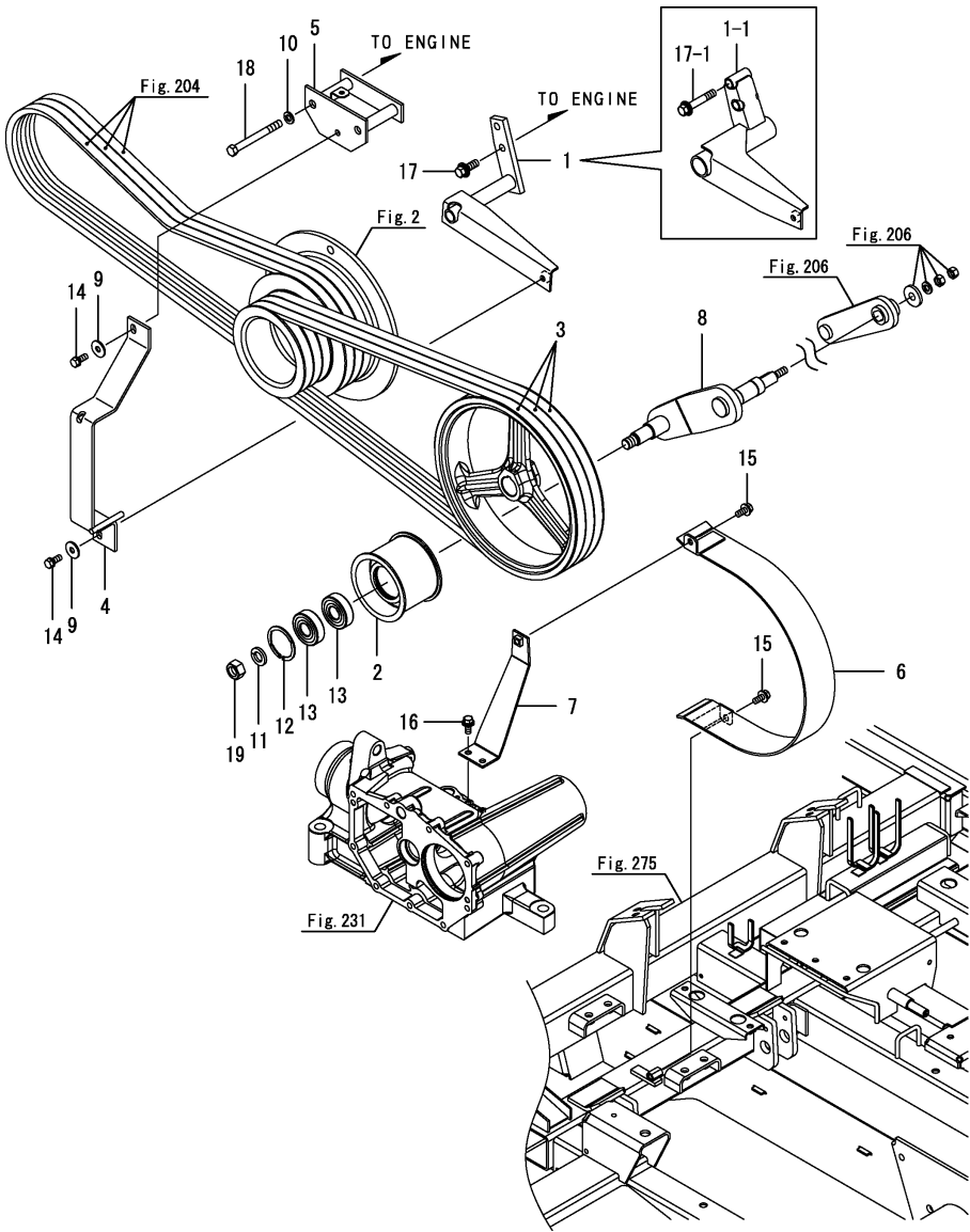
Fig.205. 탈곡구동(1)
