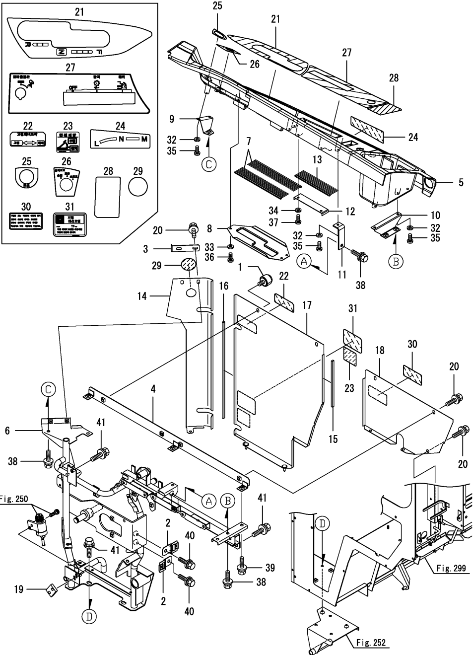
Fig.247. 측면 컬럼(1)(피칭 U.F.O.)
