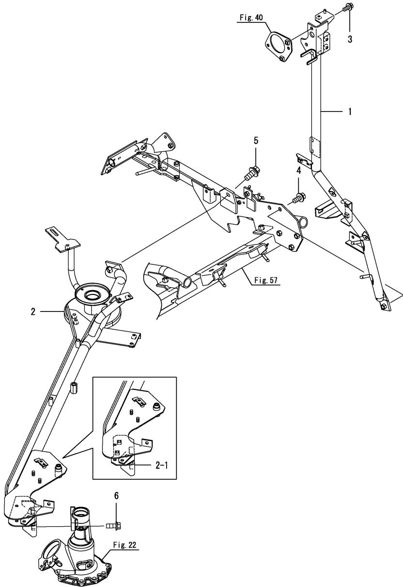
Fig.78. 끌어모음프레임(우)
