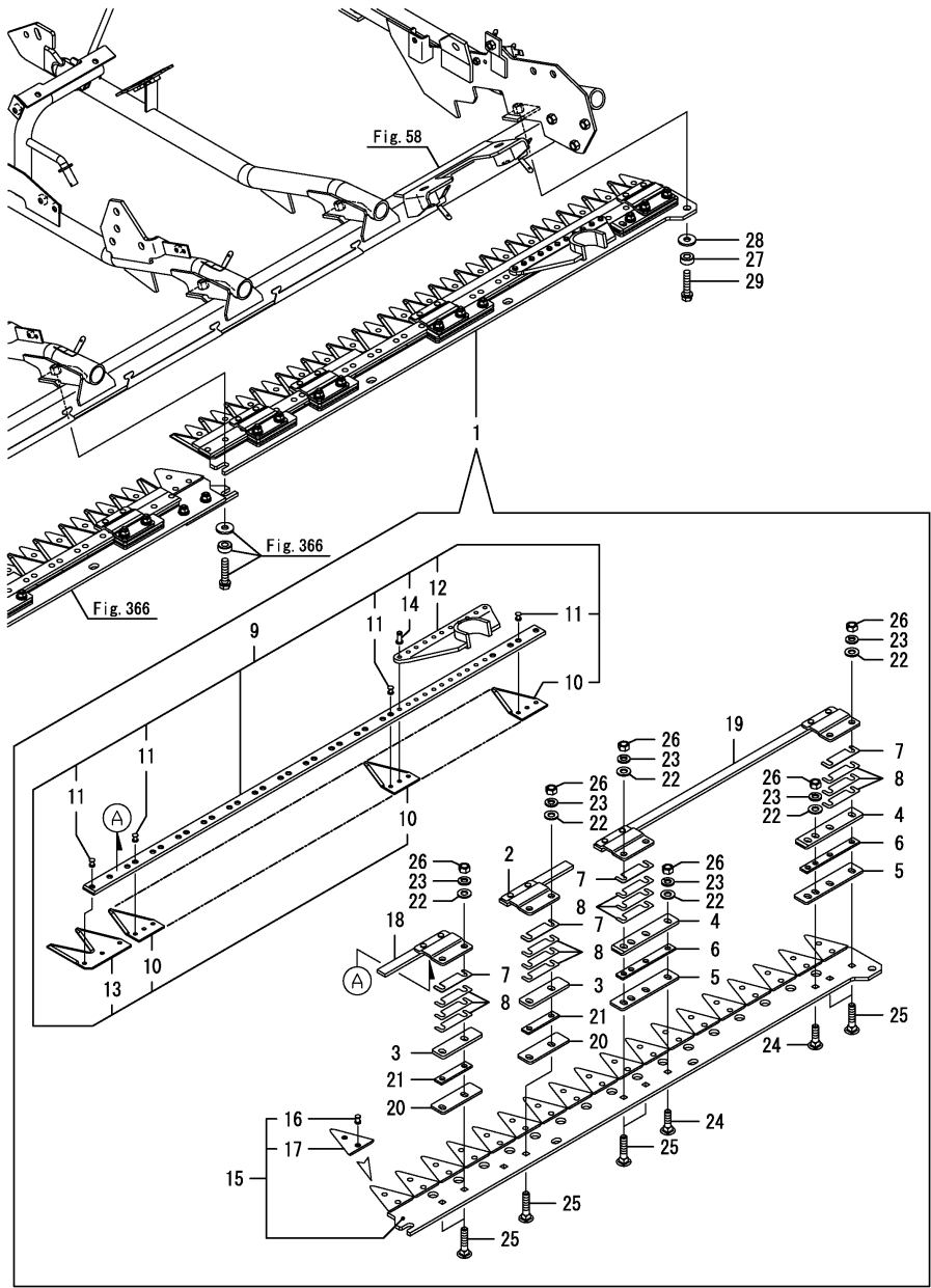
Fig.367. (64A)수확 에지(우측)
