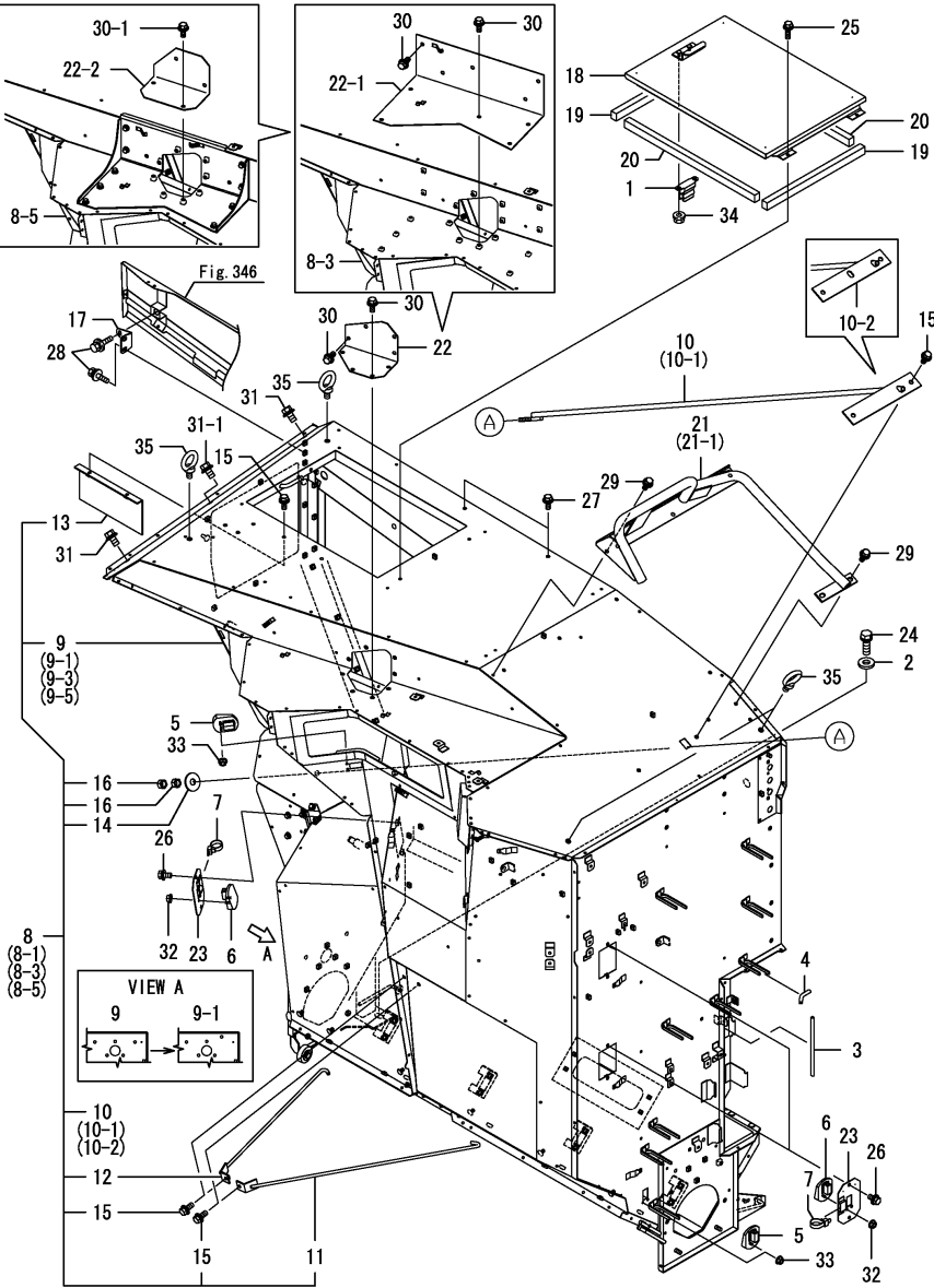
Fig.345. 곡물탱크(1)
