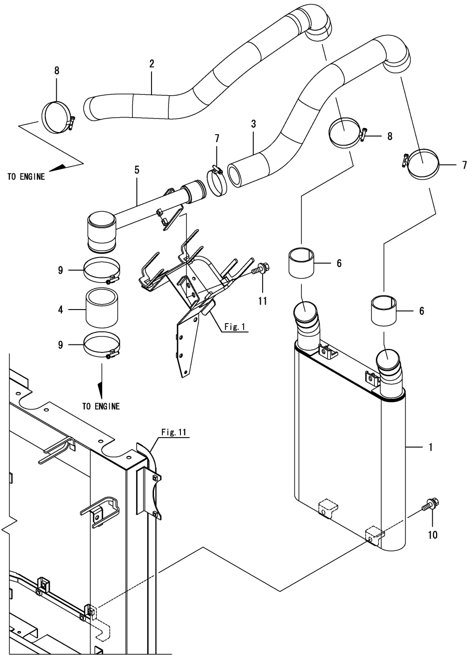
Fig.9. 인터쿨러
