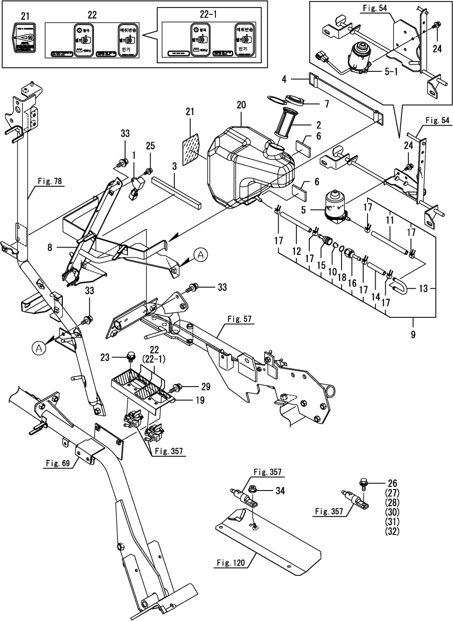
Fig.356. 주유장치(1)
