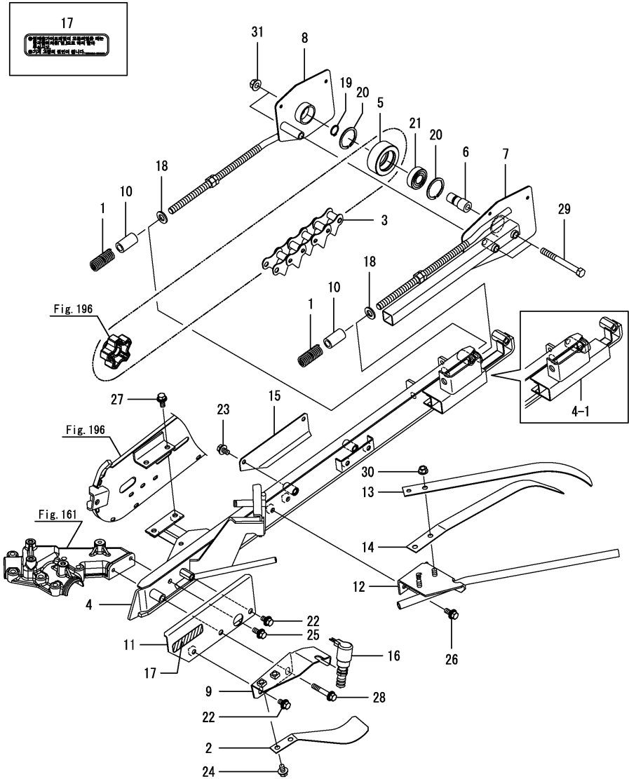
OCNP6-M05021 탈곡(2) Fig.195. 짐배출체인
