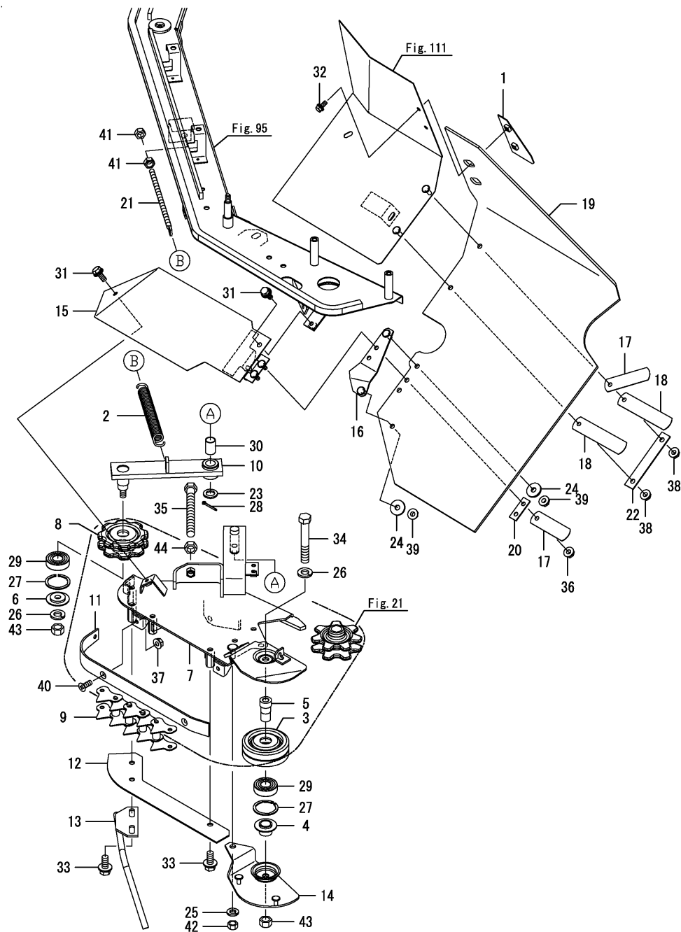
Fig.123. 보조반송케이스
