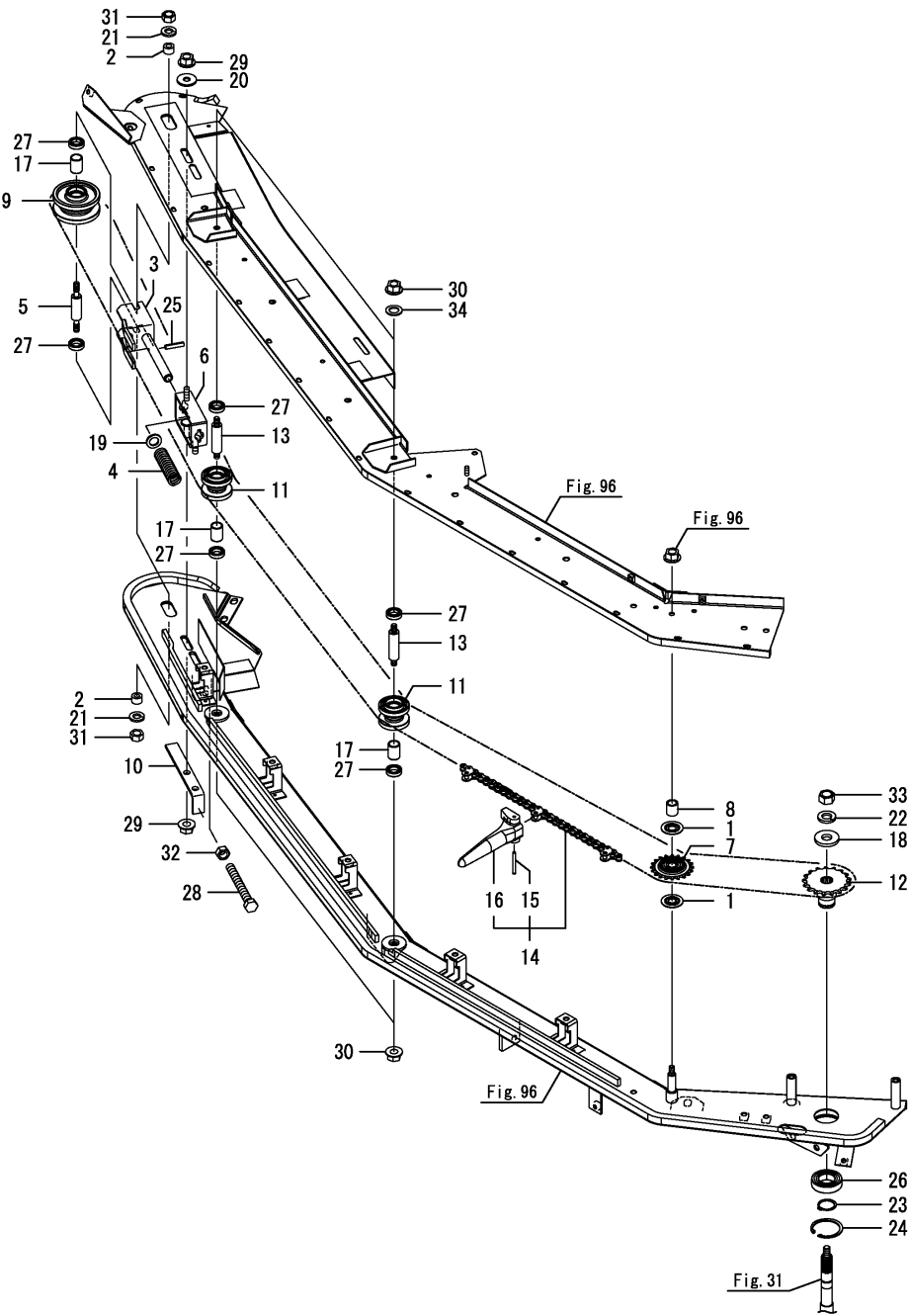
Fig.101. 상반송롤러(우)
