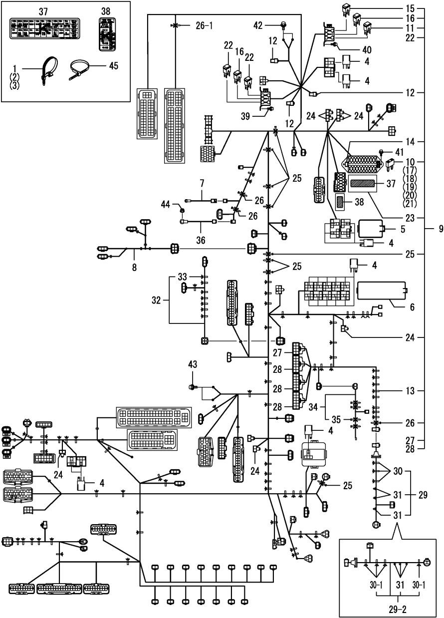
Fig.323. 와이어 하네스(주행)(피칭 U.F.O.)
