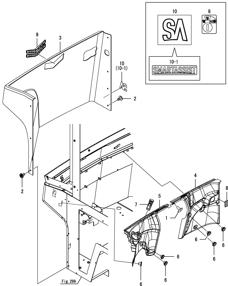
Fig.304. 캐빈의장(앞-하)
