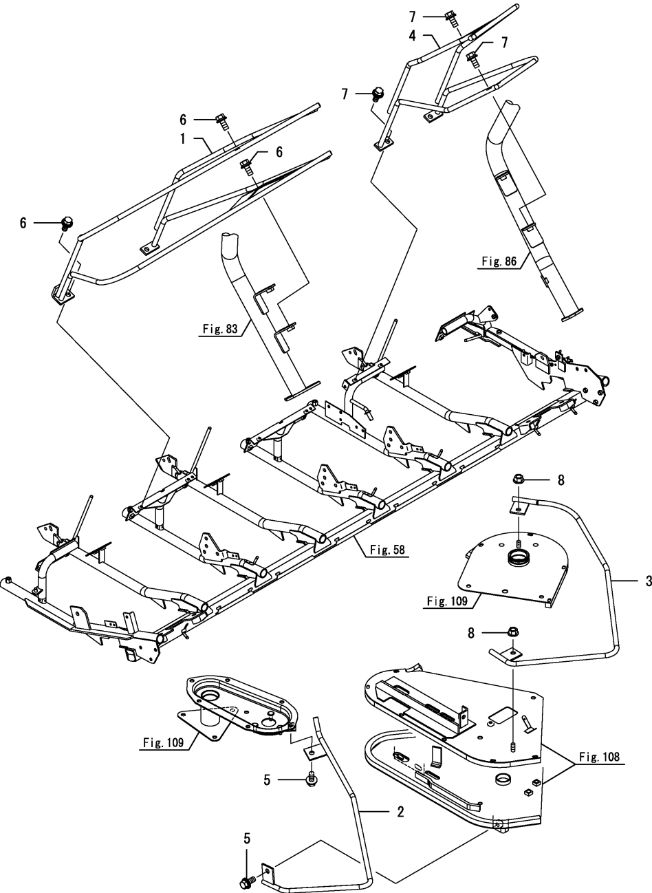
Fig.114. 상반송가이드(중)
