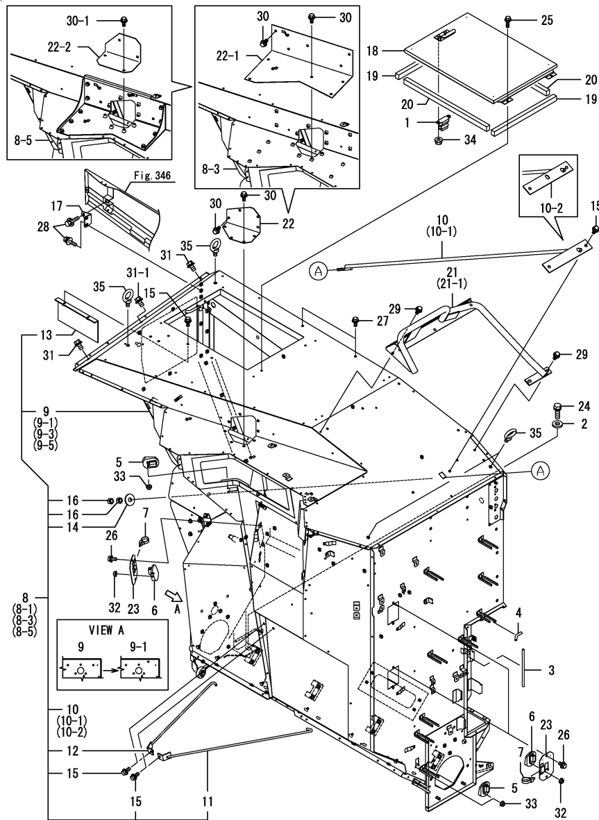
Fig.345. 곡물탱크(1)
