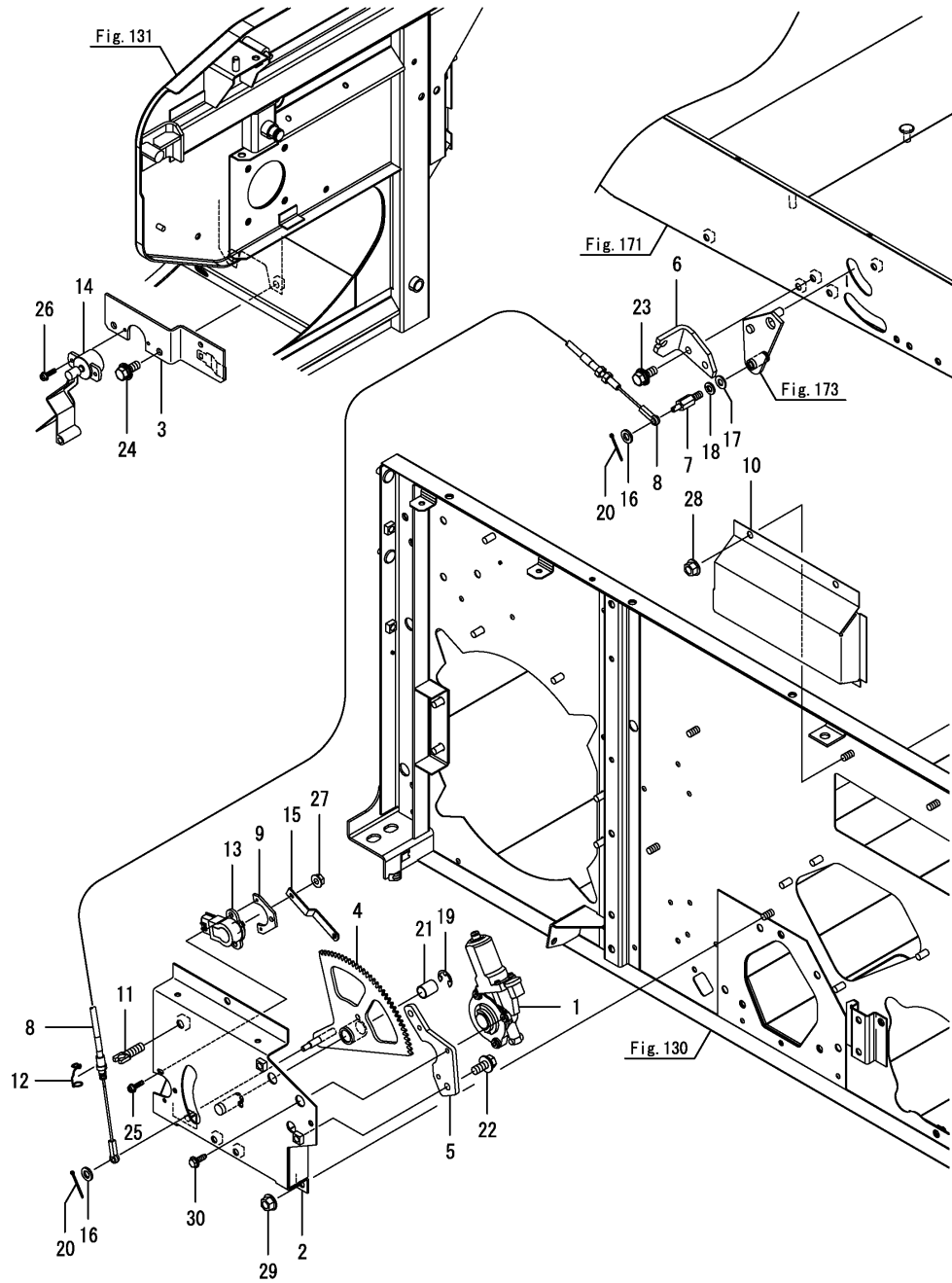
Fig.174. 요동선별조작
