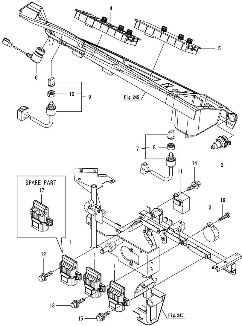
Fig.246. 사이드칼럼(2)
