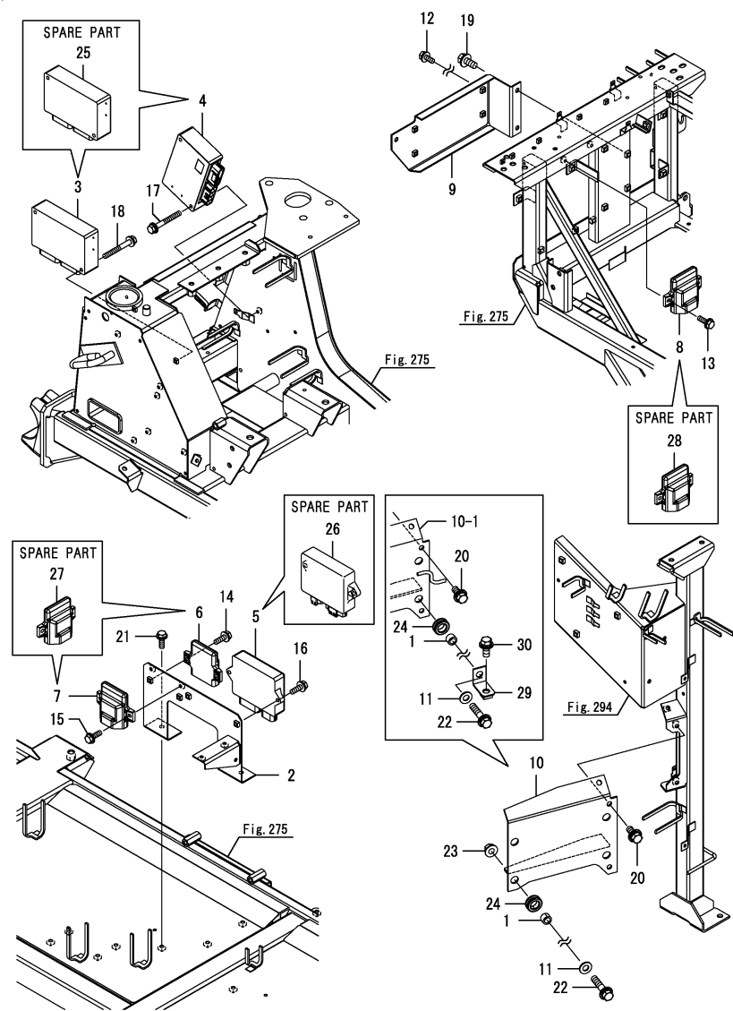
OCNP6-M05021 이동(3) Fig.278. 컨트롤(새시)(피칭 U.F.O.)
