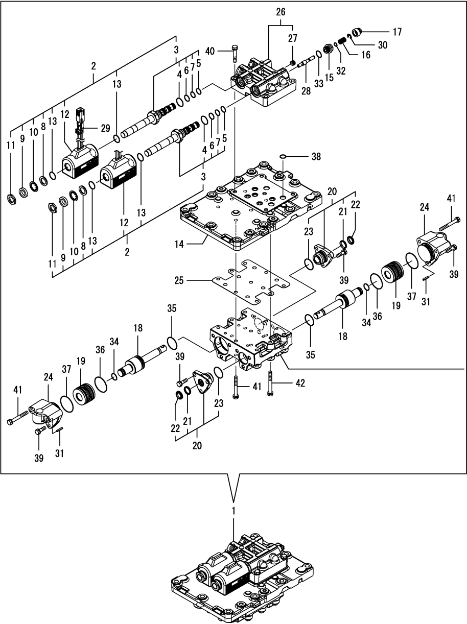
Fig.368. 카운터케이스(10)
