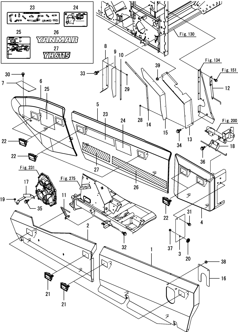
Fig.152. 탈곡통커버(앞)(사이드)
