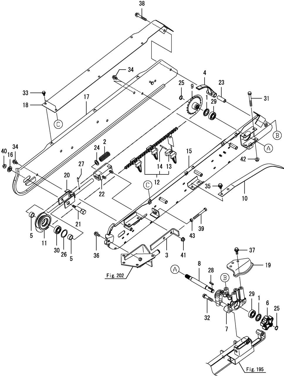
Fig.196. 쟁배출반송(이삭끝)
