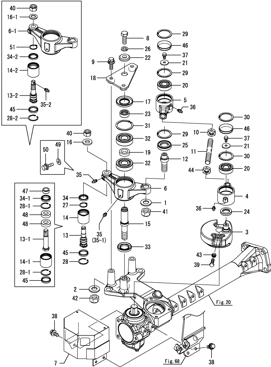
Fig.59. 예취날구동(좌)
