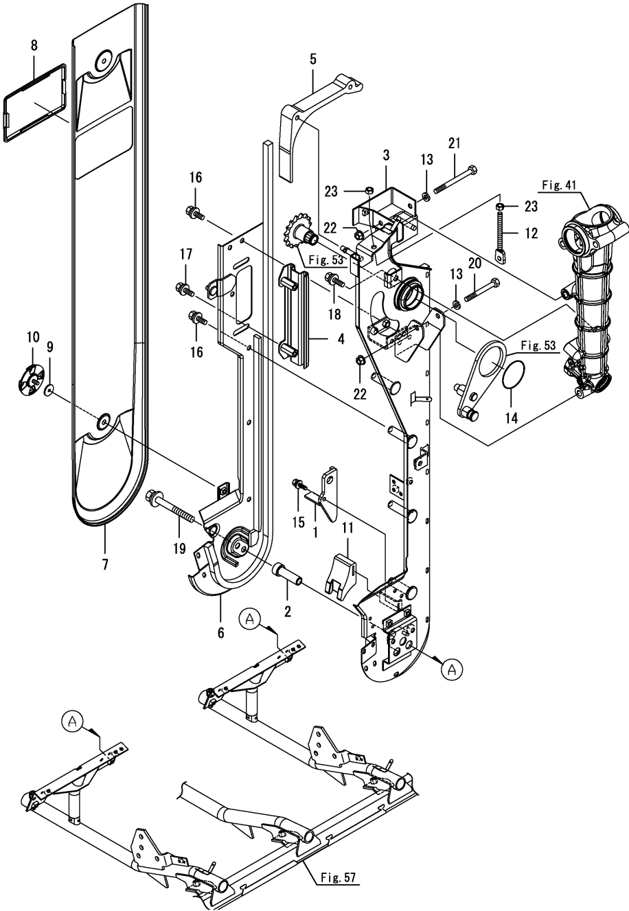
Fig.51. 픽업 케이스(중앙)(2)
