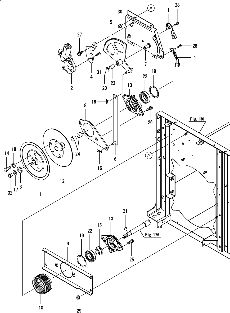
OCNP6-M05021 탈곡(1) Fig.143. 풍구 벨트
