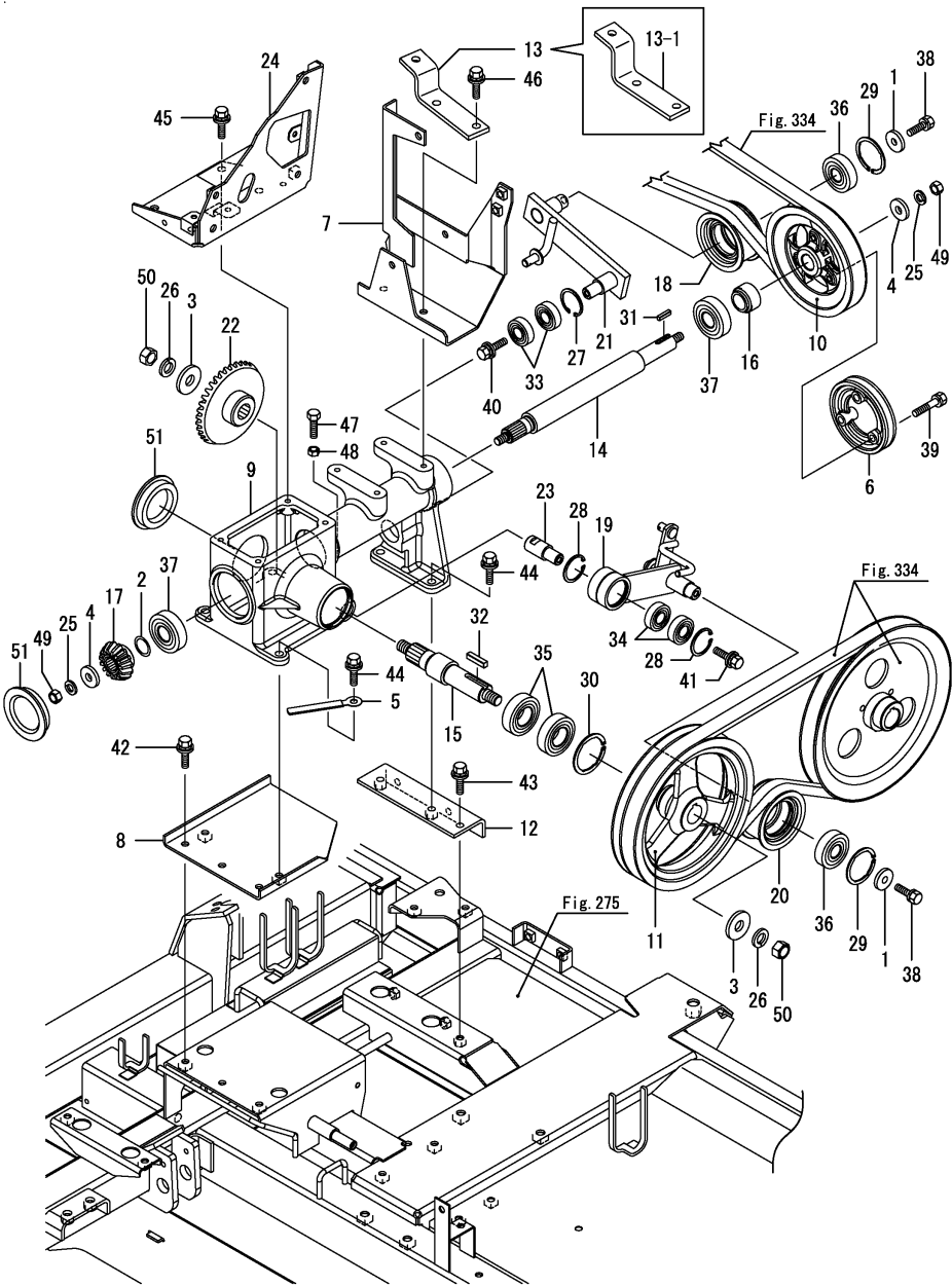
Fig.333. 오거입력
