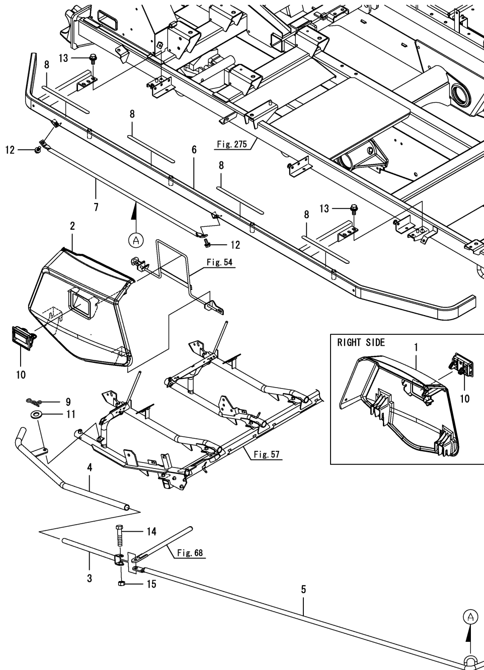
Fig.15. 예취(2)
