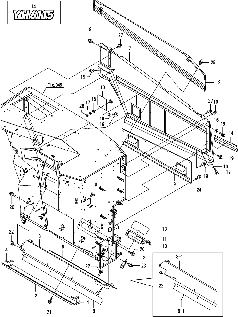
Fig.346. 곡물탱크(2)
