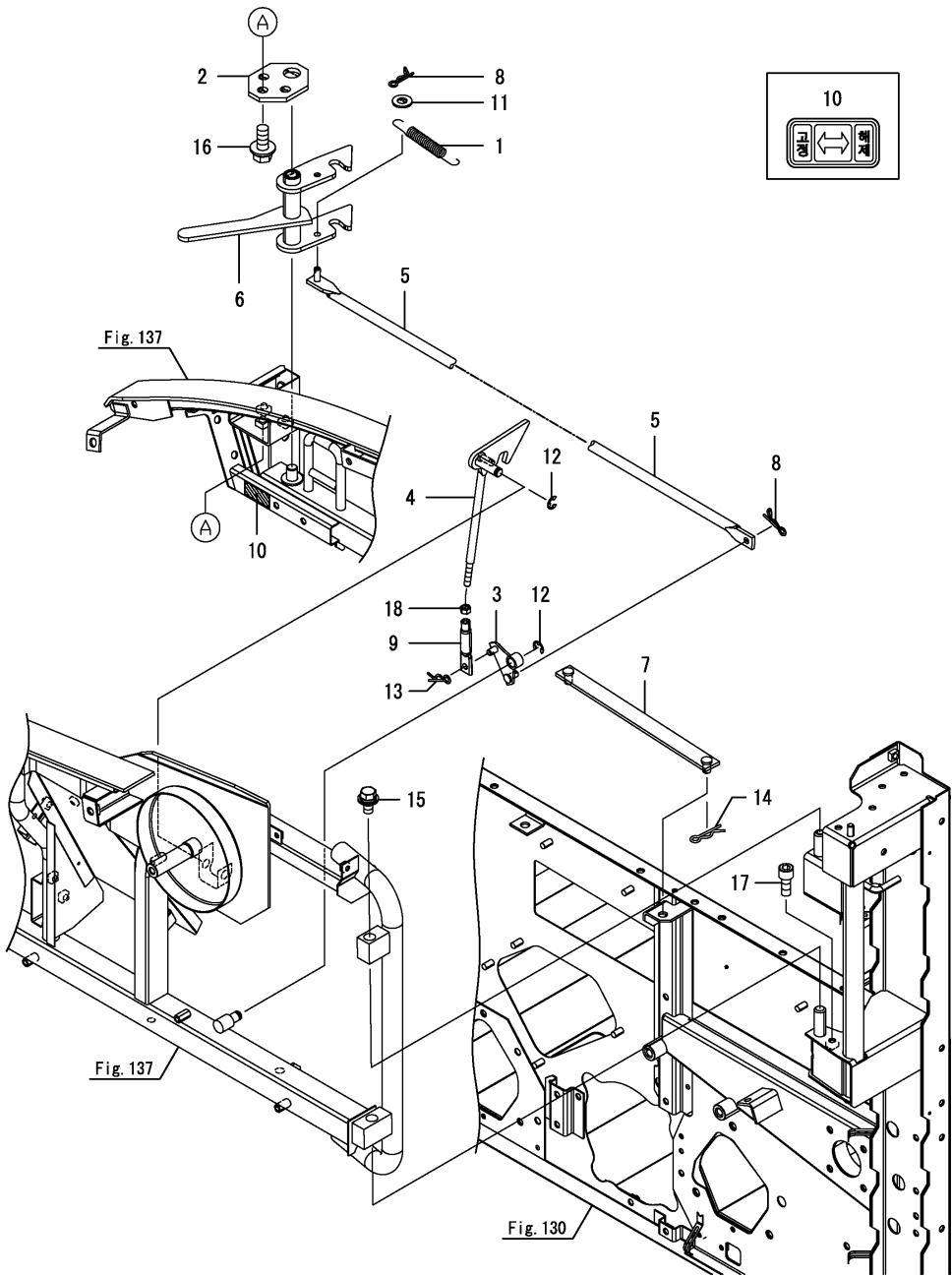
Fig.138. 탈곡실프레임(좌)(2)
