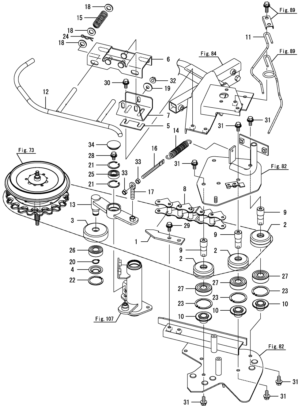
Fig.93. 하부반송가이드(중-좌)
