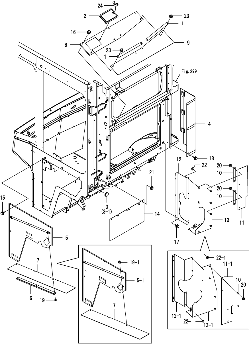
Fig.305. 캐빈시일(1)
