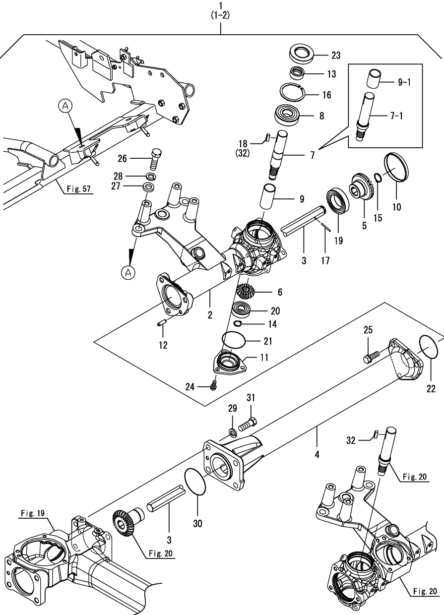
Fig.24. 6조구동케이스(7)
