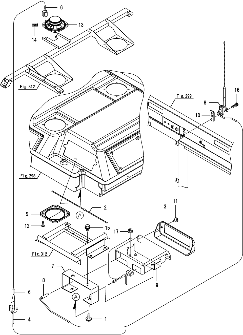
Fig.307. 스테레오
