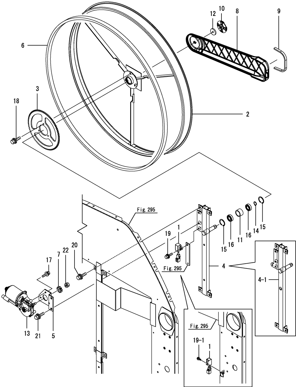
Fig.12. 회전 스크린
