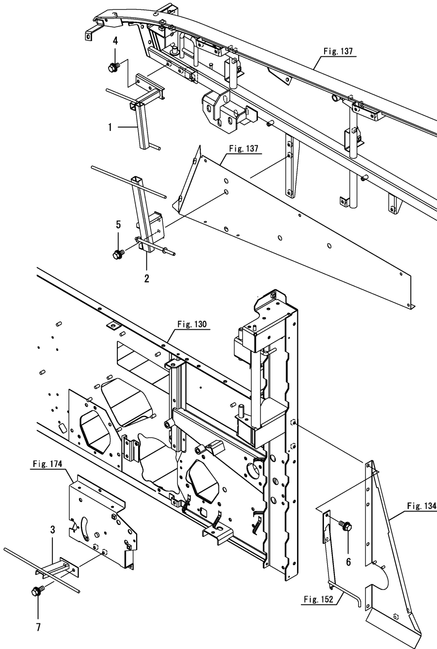
Fig.151. 사이드커버(좌)
