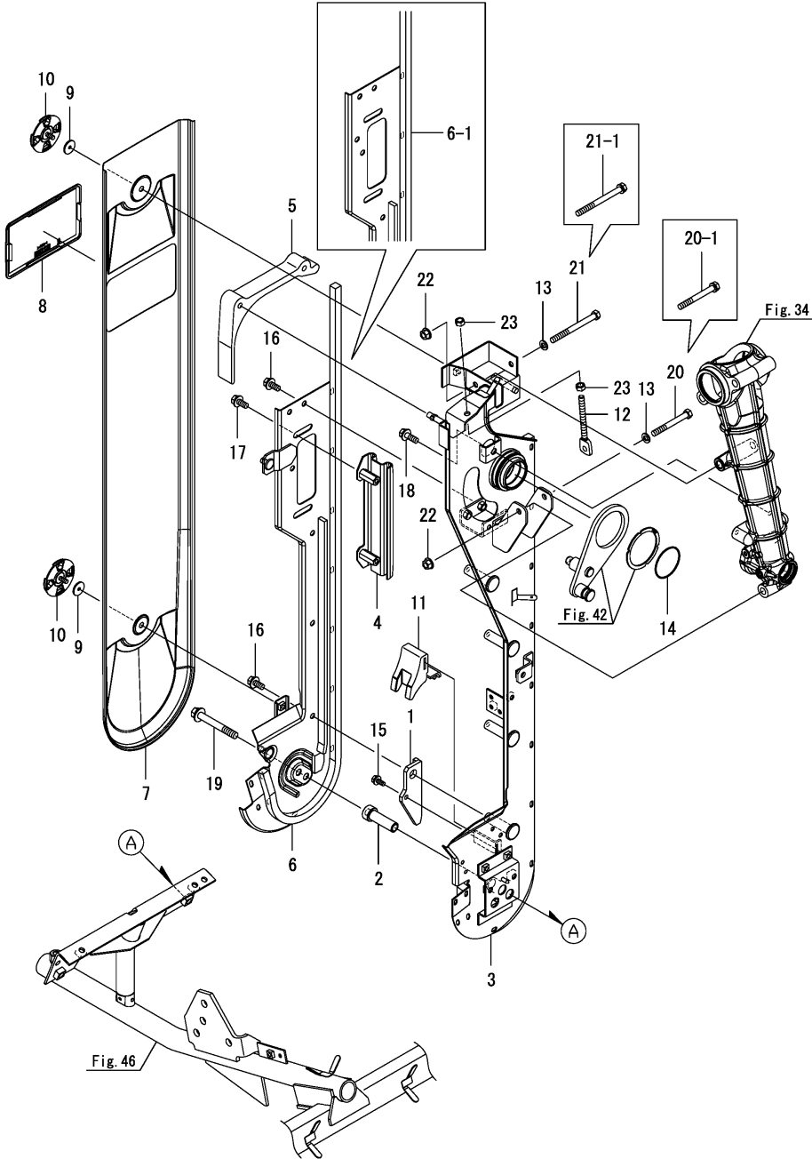
Fig.41. 인기케이스(중)
