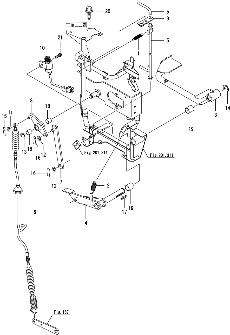
Fig.204. 브레이크조작
