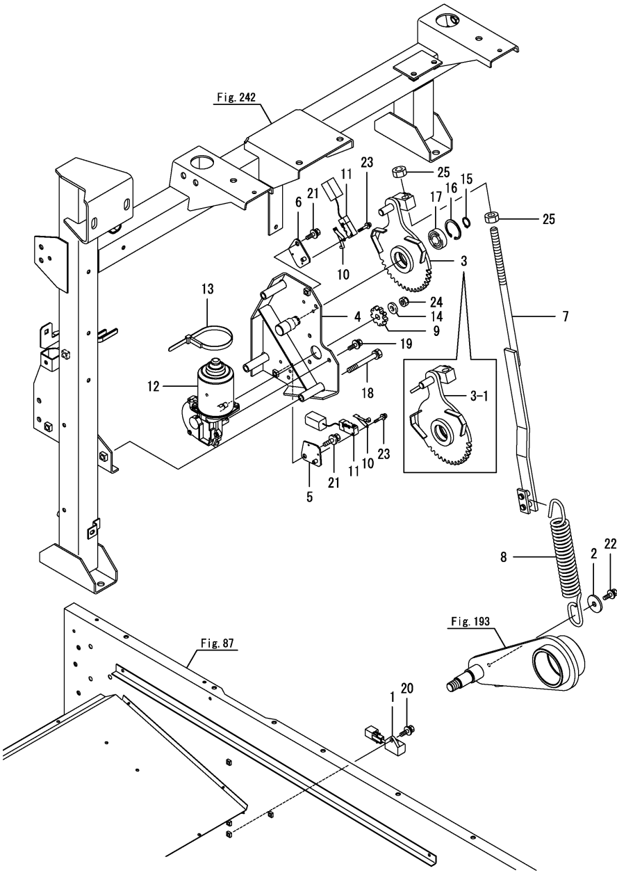
Fig.163. 탈곡구동(2)
