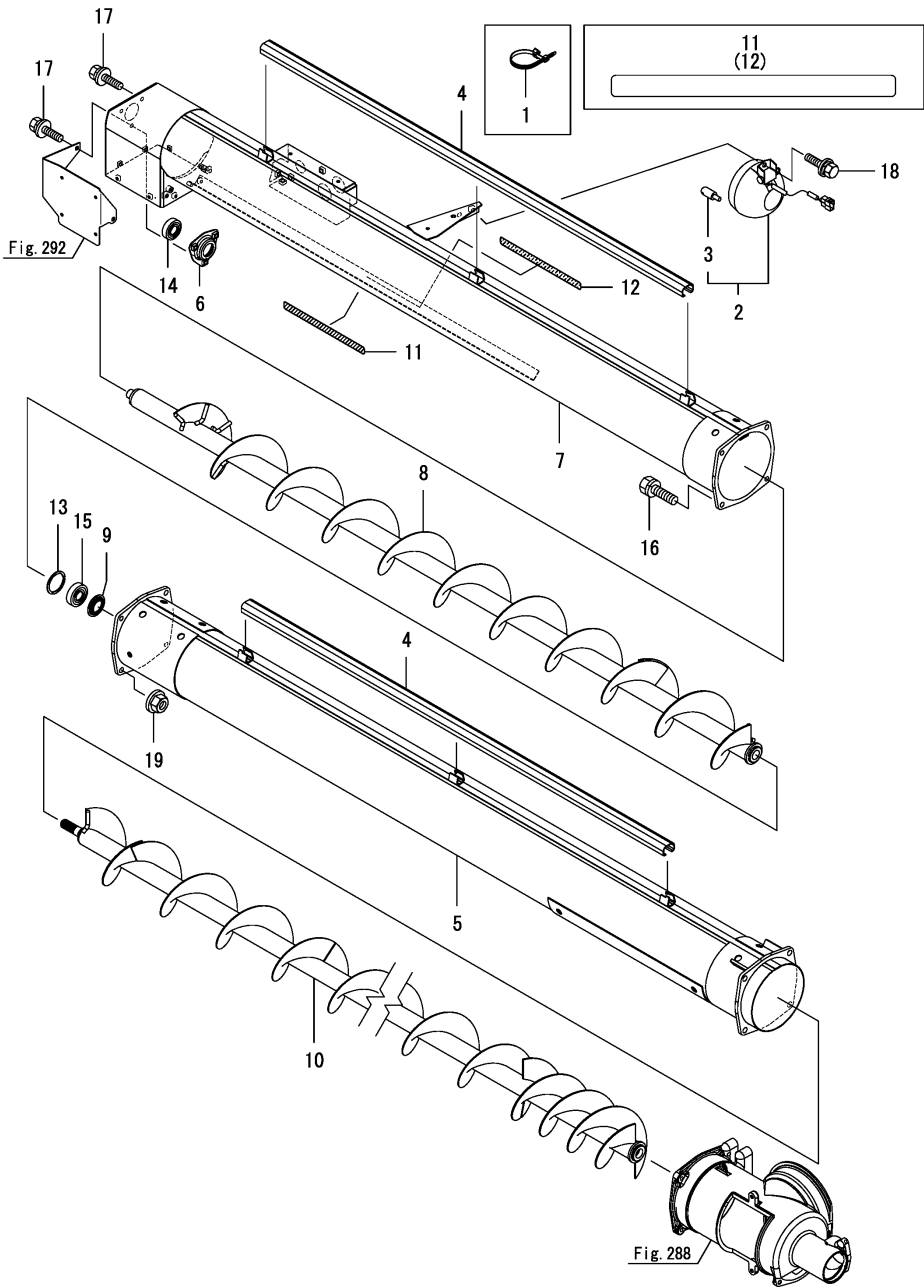
Fig.291. 오거(측면)
