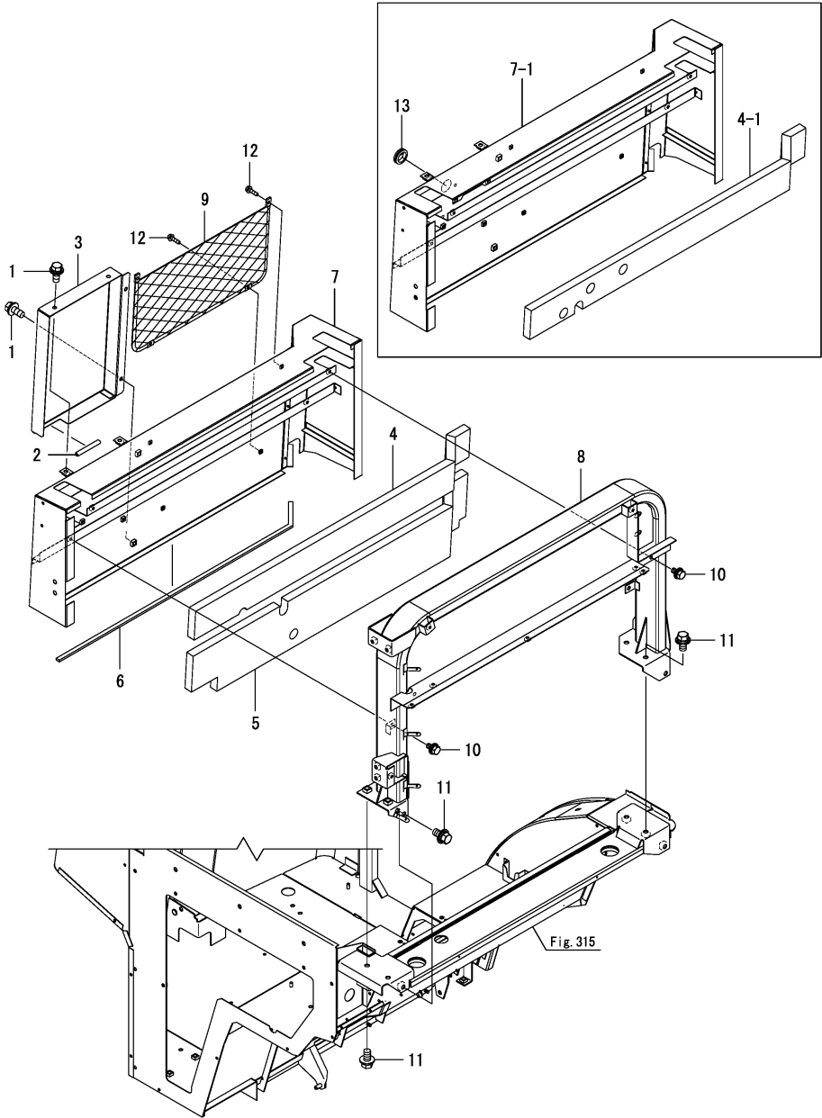
OCNP6-M07371 이동(2) Fig.316. 후방 칼럼(바닥)
