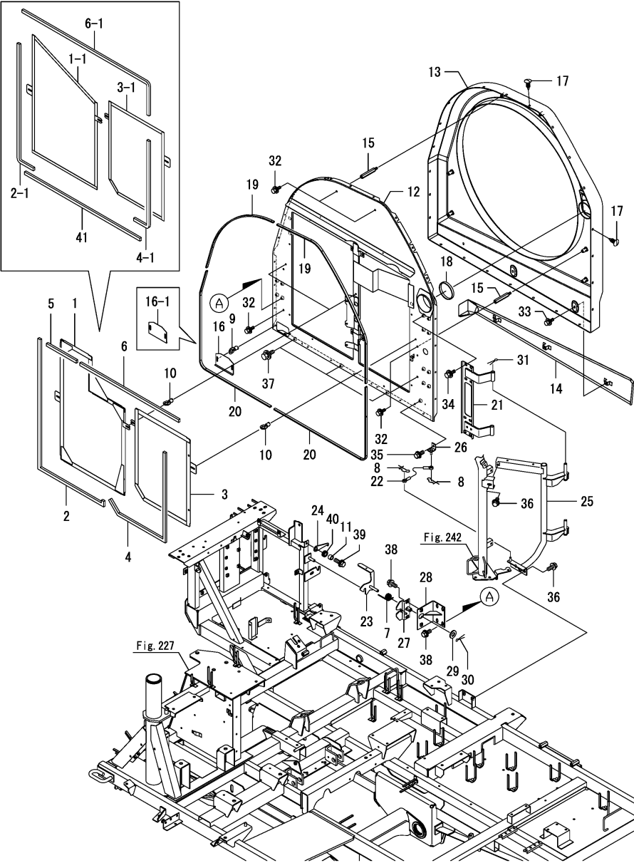
Fig.243. 엔진실 커버
