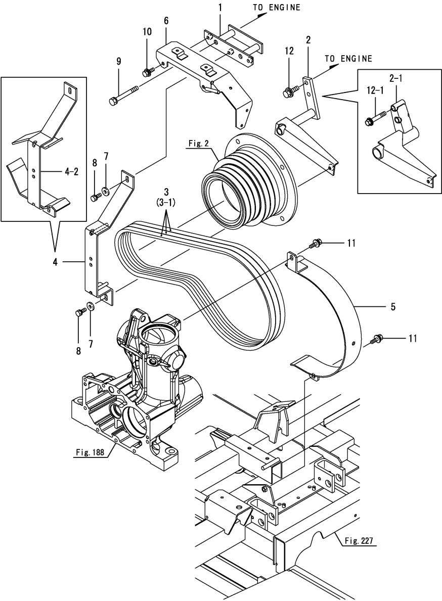
Fig.162. 탈곡구동(1)
