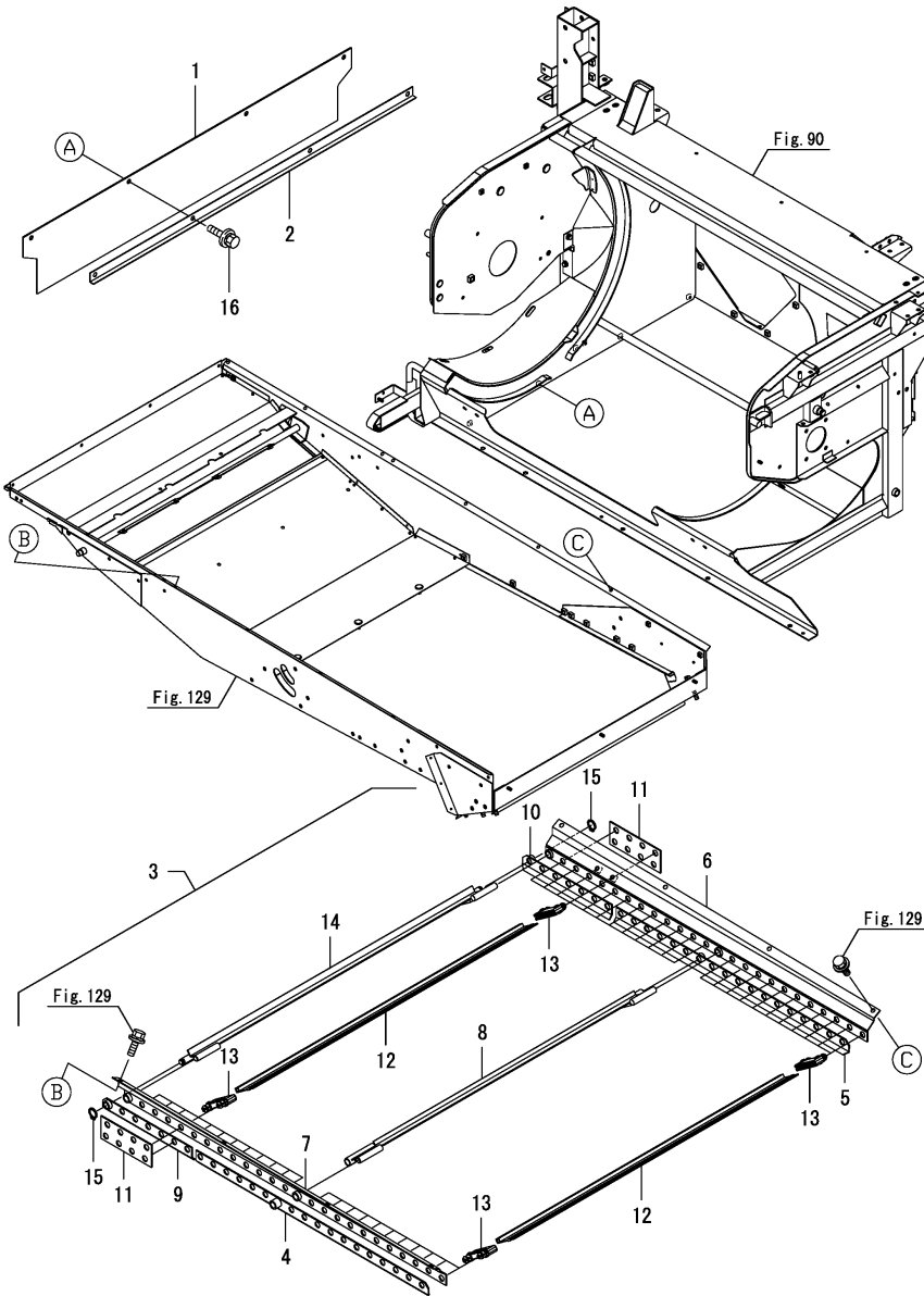
Fig.128. 요동선별프레임(1)
