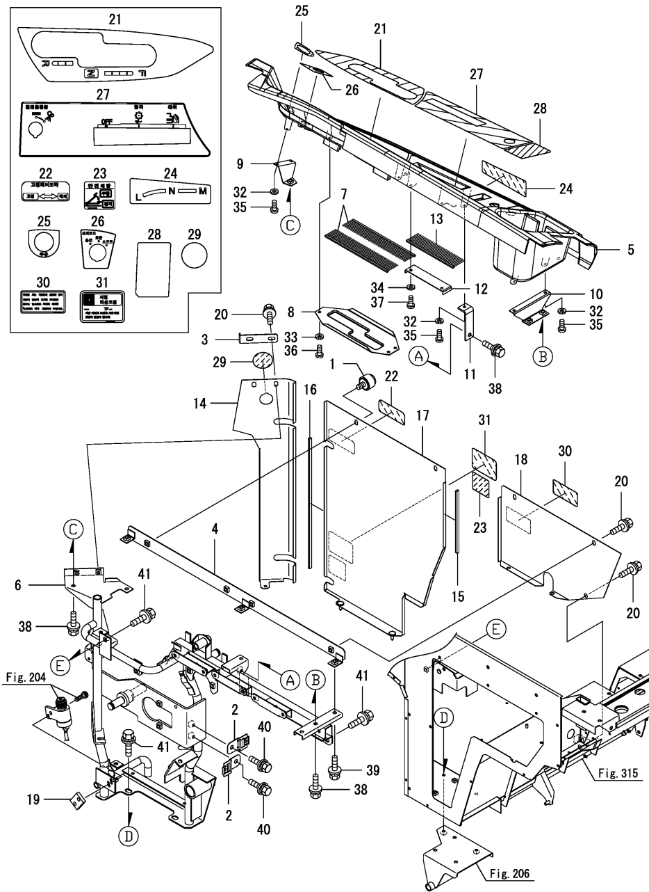
Fig.311. 사이드 칼럼(바닥)(1)
