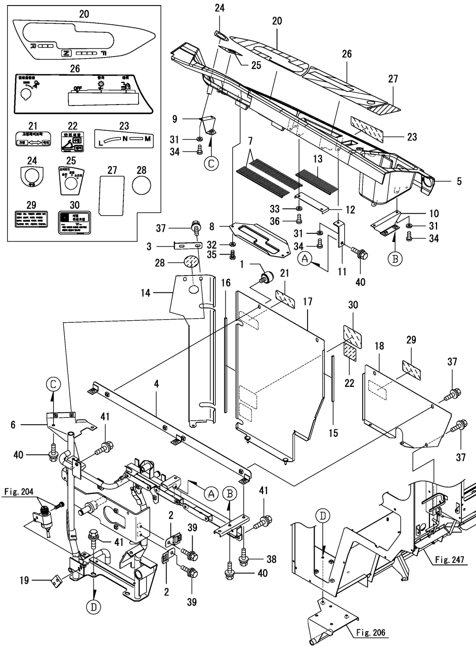
Fig.201. 사이드칼럼(1)
