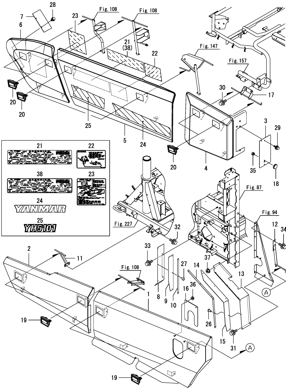
Fig.109. 사이드커버
