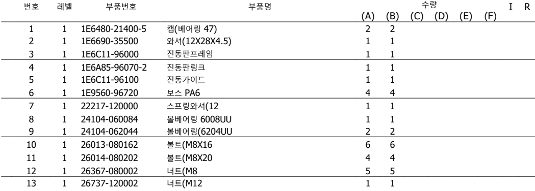
(A)=YH5101-KR (B)=YH5101-AKR (C)=
