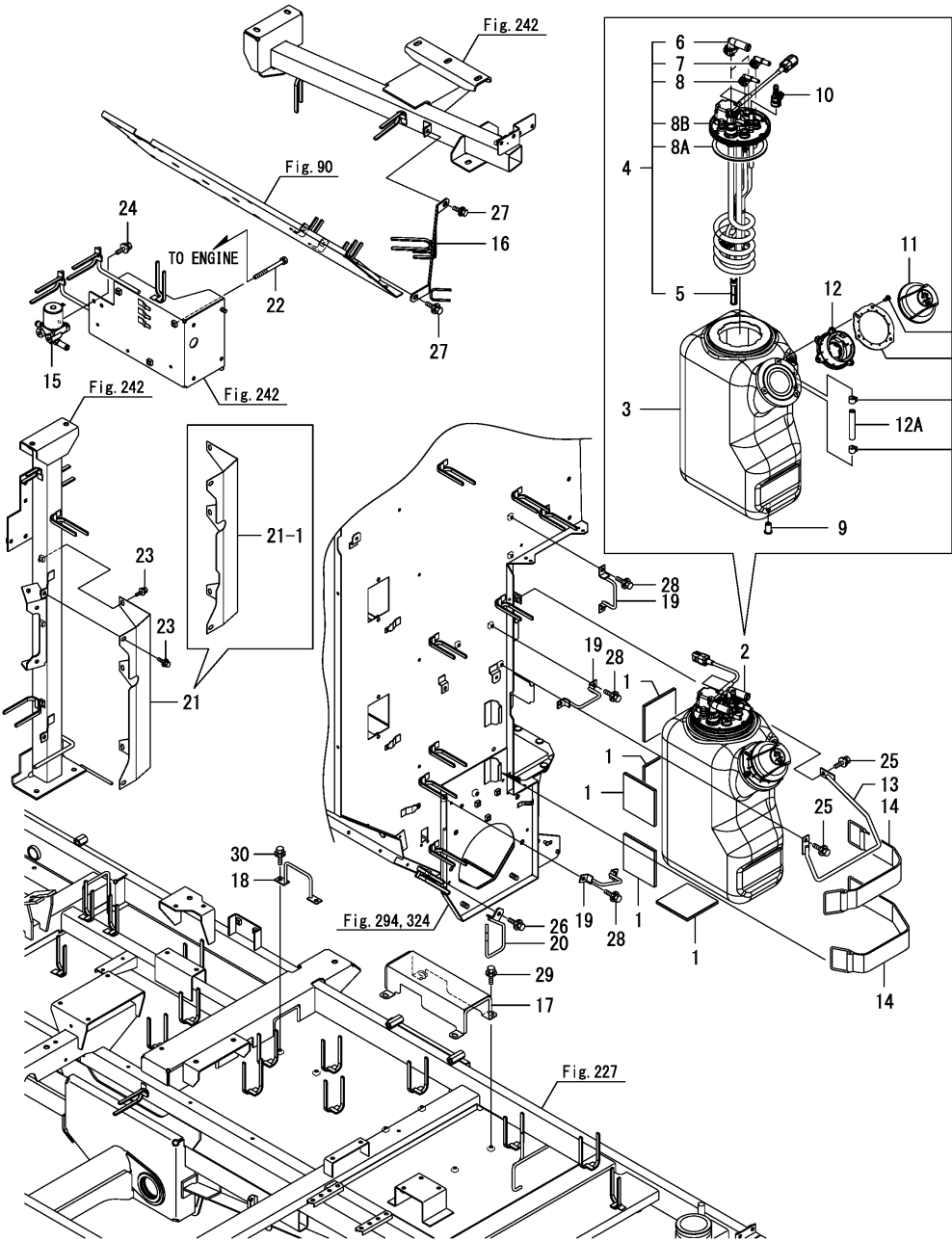
Fig.6. 요소 탱크(1)
