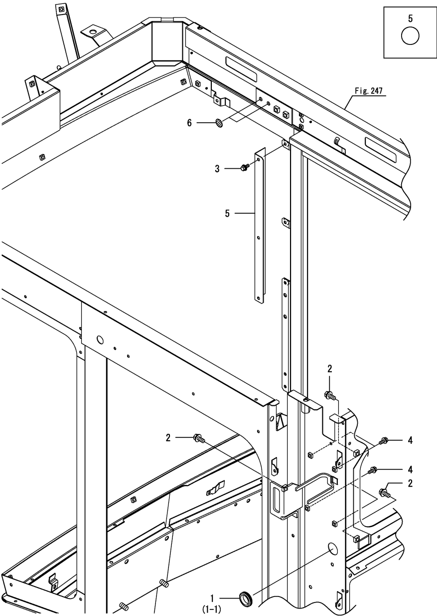
Fig.280. 모니터 없음
