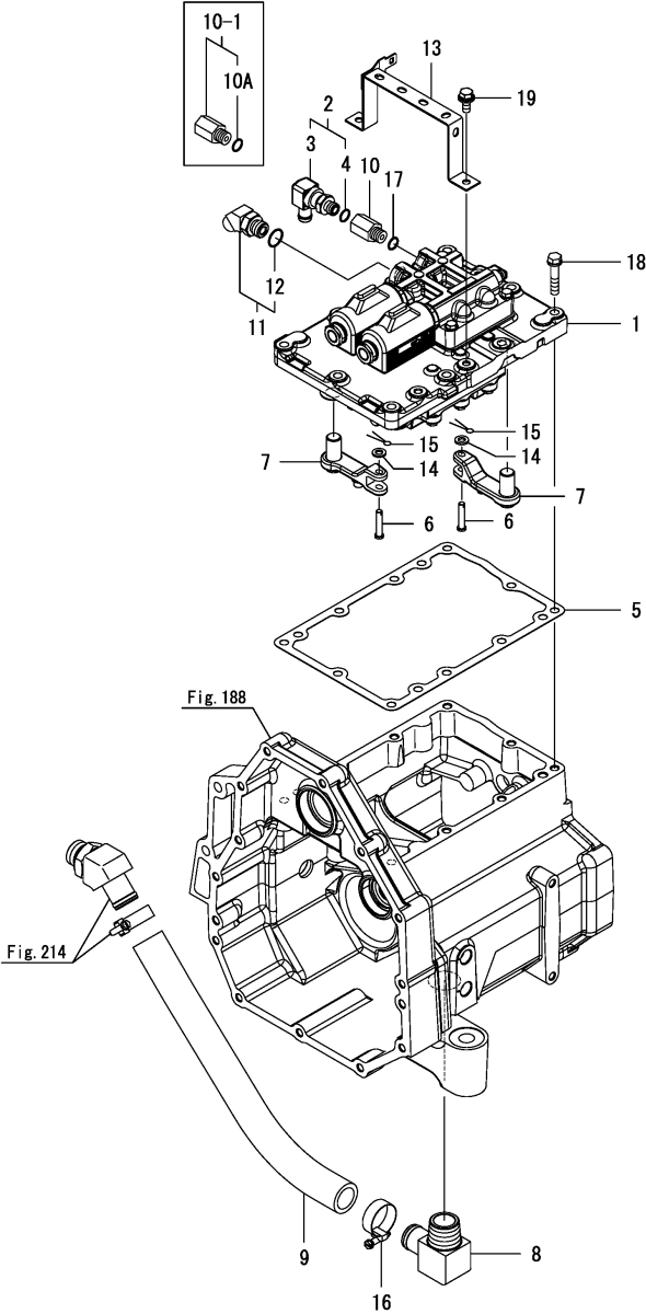
Fig.189. 카운터케이스(2)
