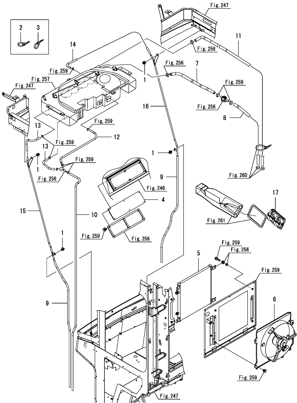
Fig.258. 에어컨(3)
