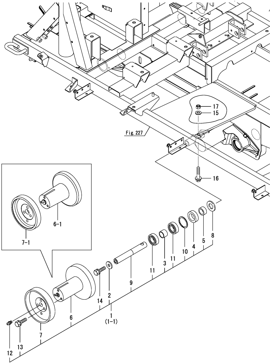
Fig.238. 캐리어 롤러
