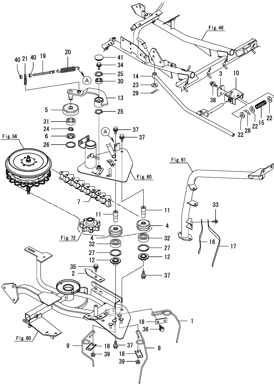
OCNP6-M07371 수확(2) Fig.65. 하부반송가이드(중-좌)
