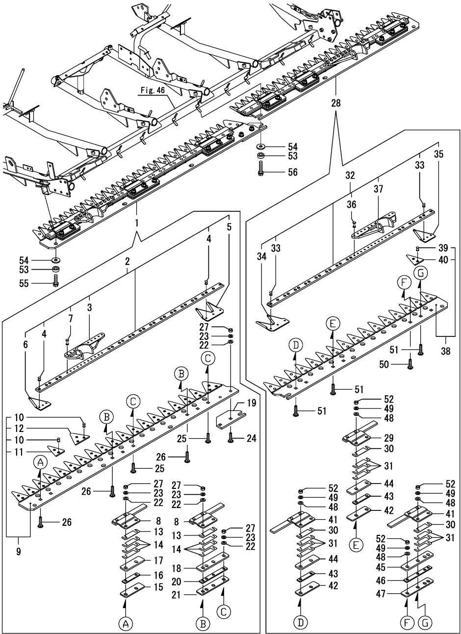
Fig.49. 예취날
