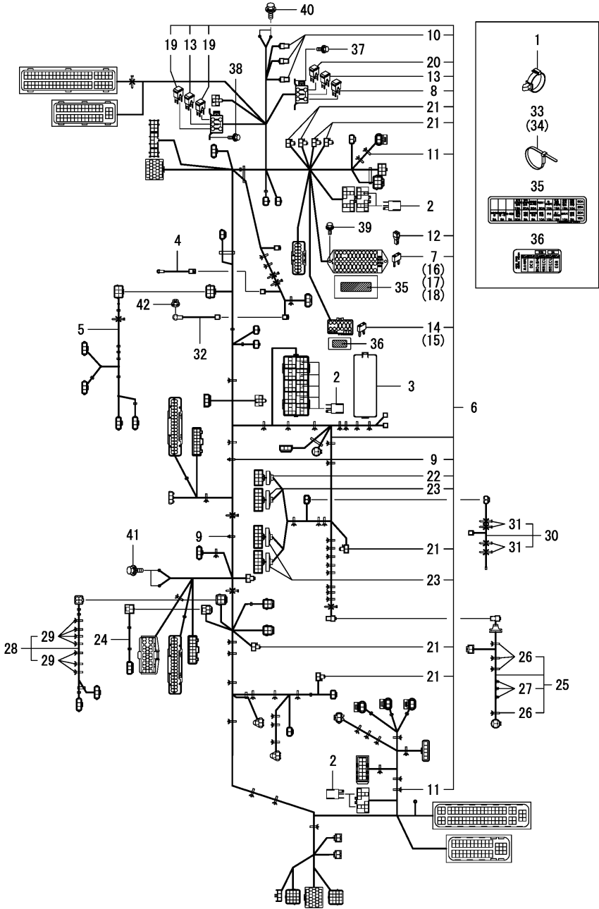
Fig.344. 배선 하네스(주행)(바닥)
