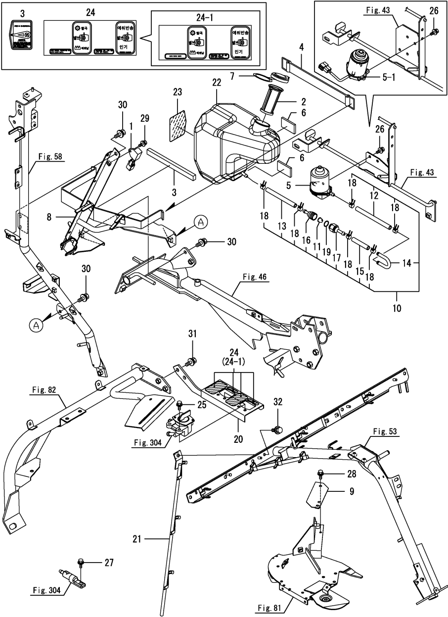
Fig.303. 주유장치(1)
