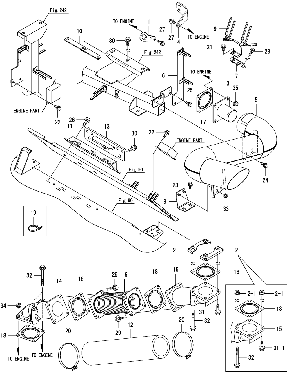
Fig.11. 머플러
