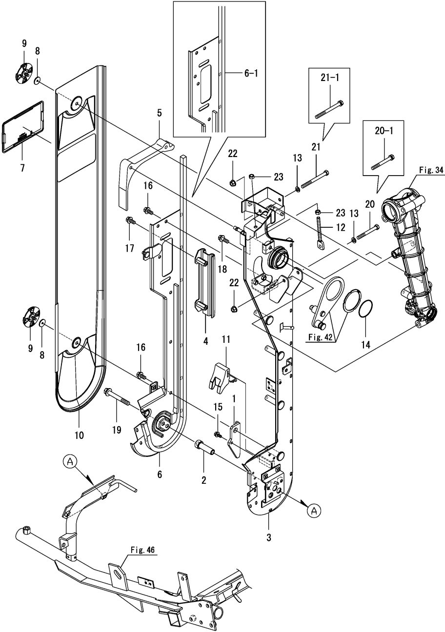
Fig.38. 픽업 케이스(왼쪽)
