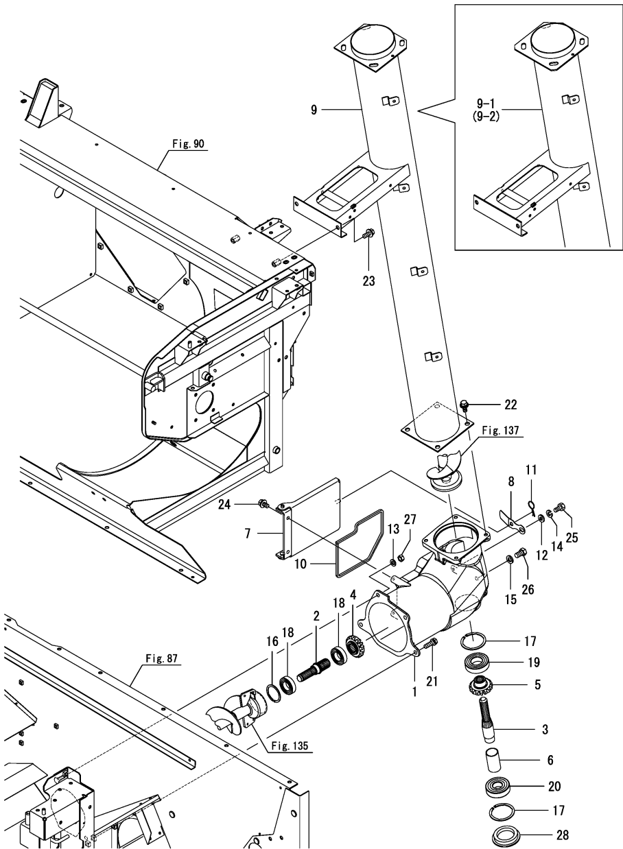
Fig.136. 컨베이어케이스
