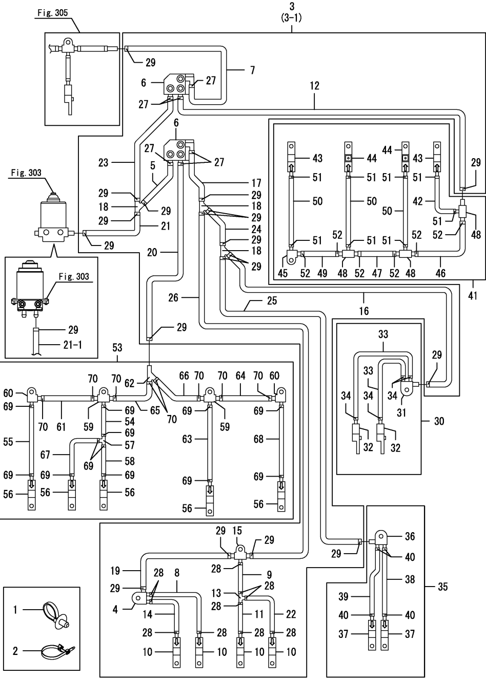
Fig.304. 주유장치(2)
