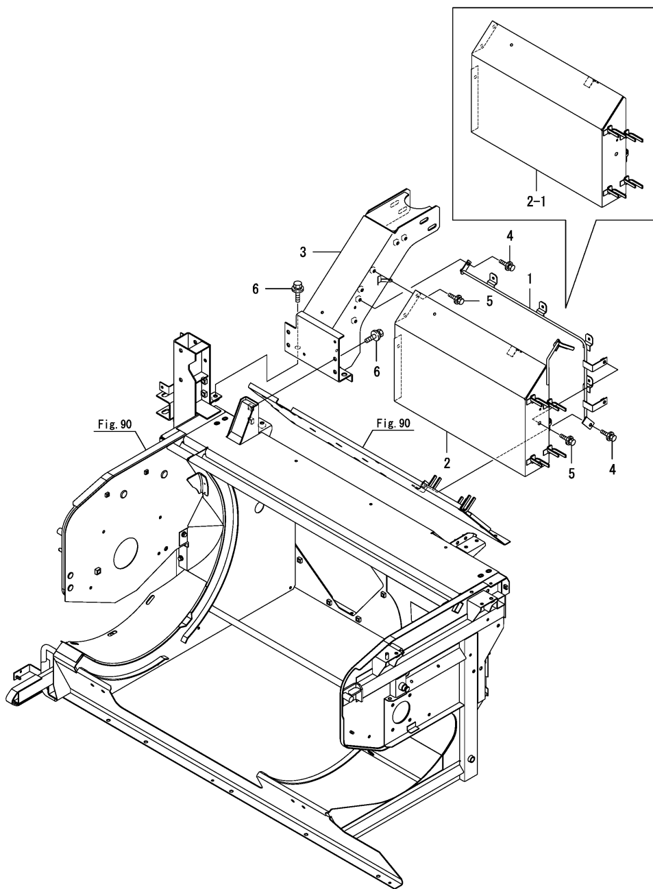
Fig.296. 탱크 고정(1)
