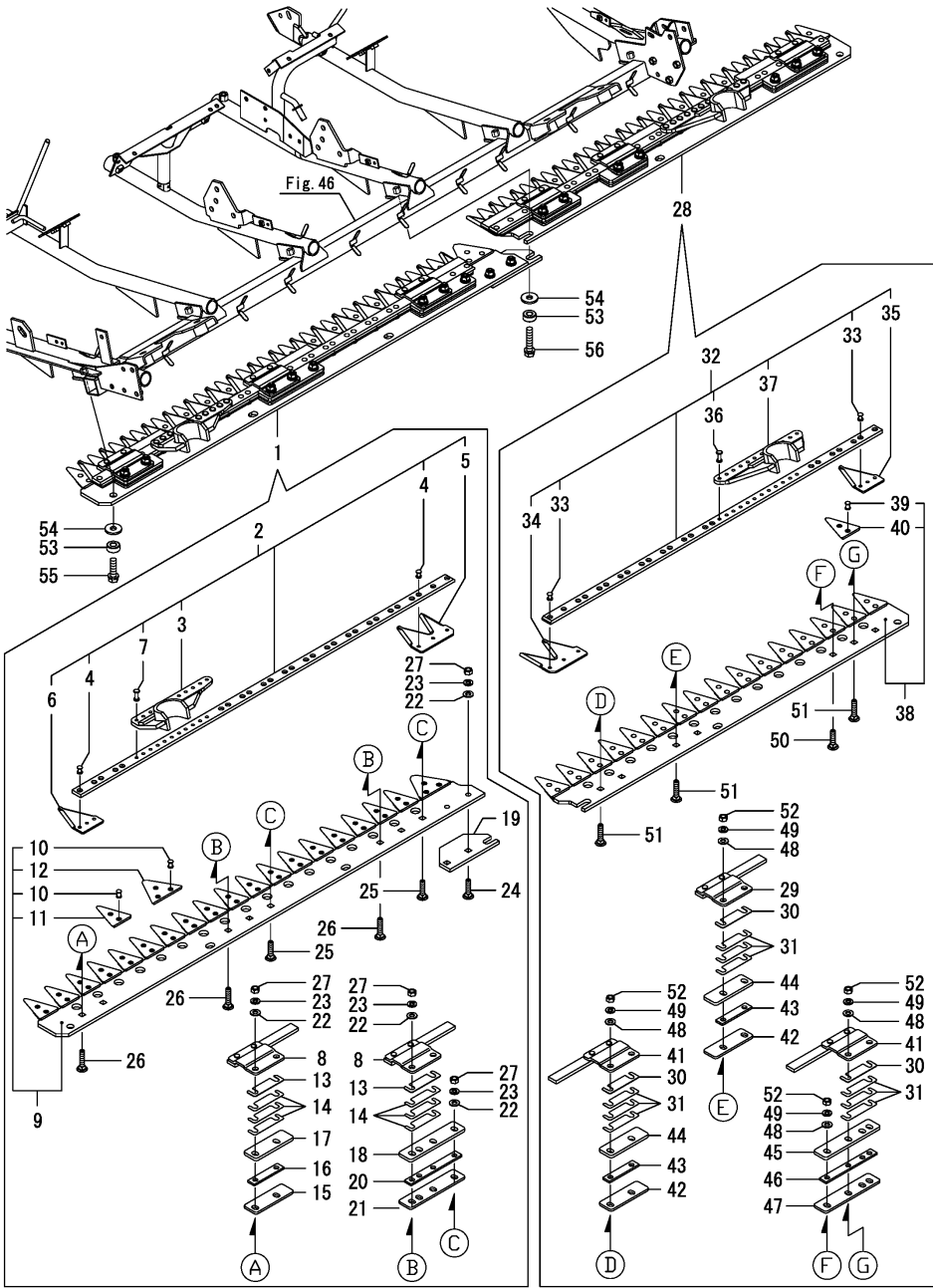
Fig.49. 예취날
