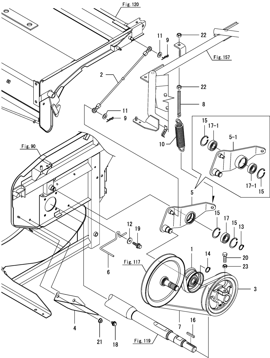
Fig.112. 쥘 방출 벨트
