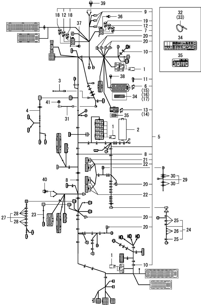
Fig.343. 배선(주행)
