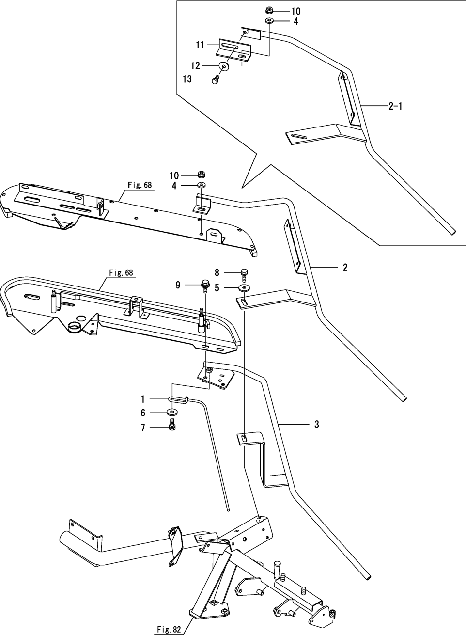
Fig.76. 상부잡이가이드
