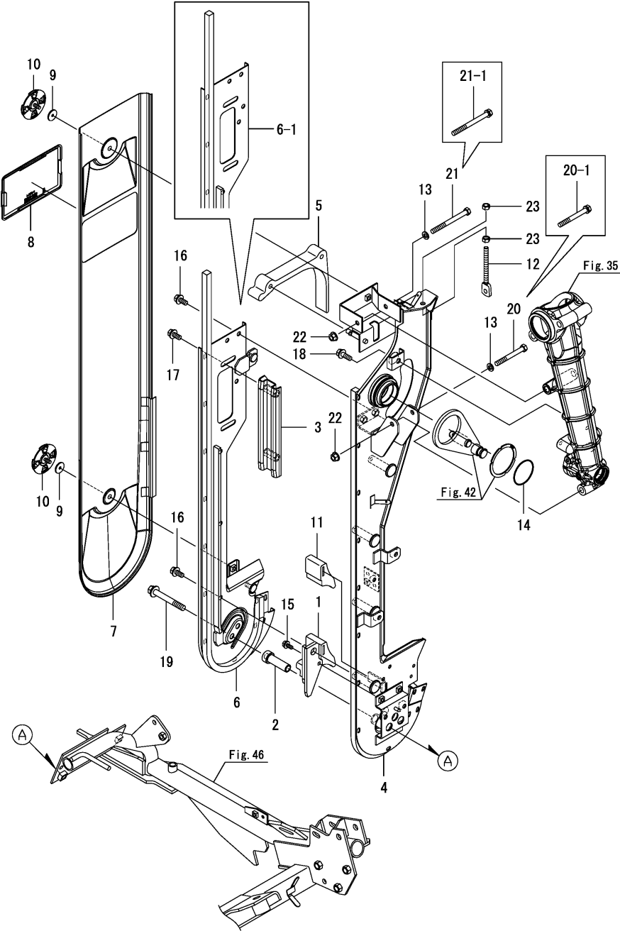
Fig.37. 픽업 케이스(오른쪽)
