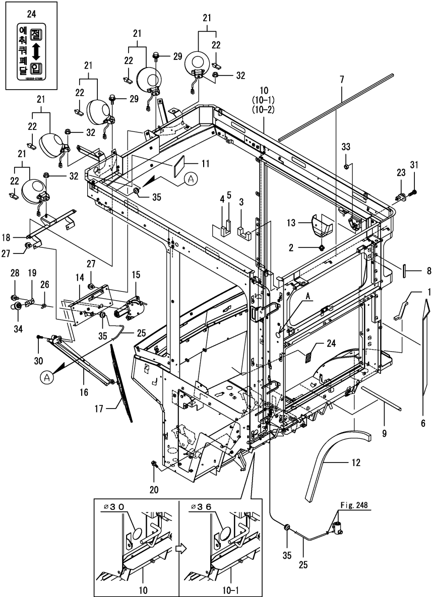
OCNP6-M07371 캐빈부 Fig.247. 캐빈(몸체)
