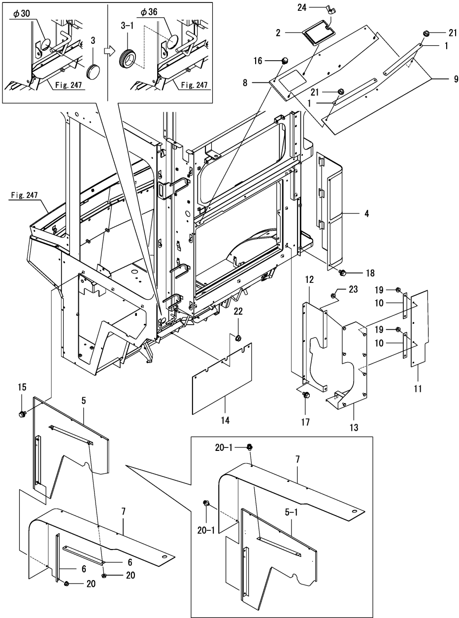
Fig.253. 캐빈시일(1)
