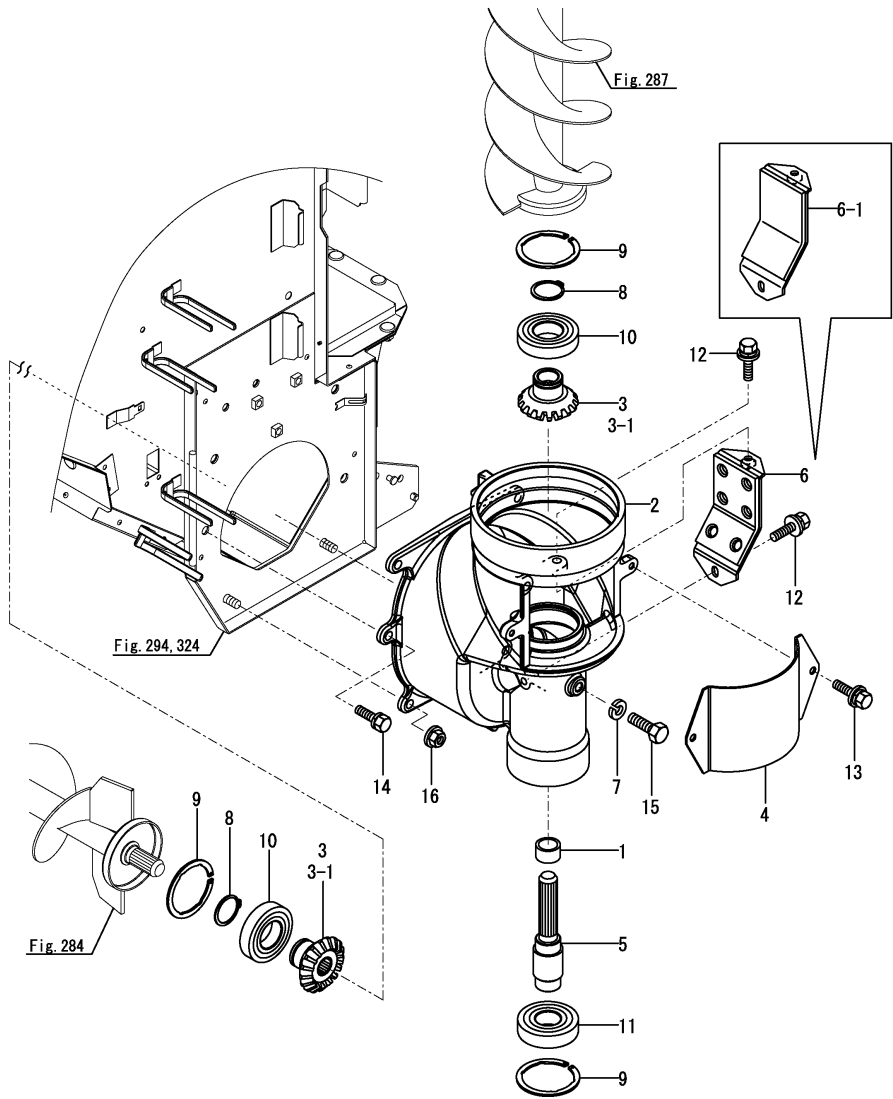
Fig.285. 하부컨베이어연결
