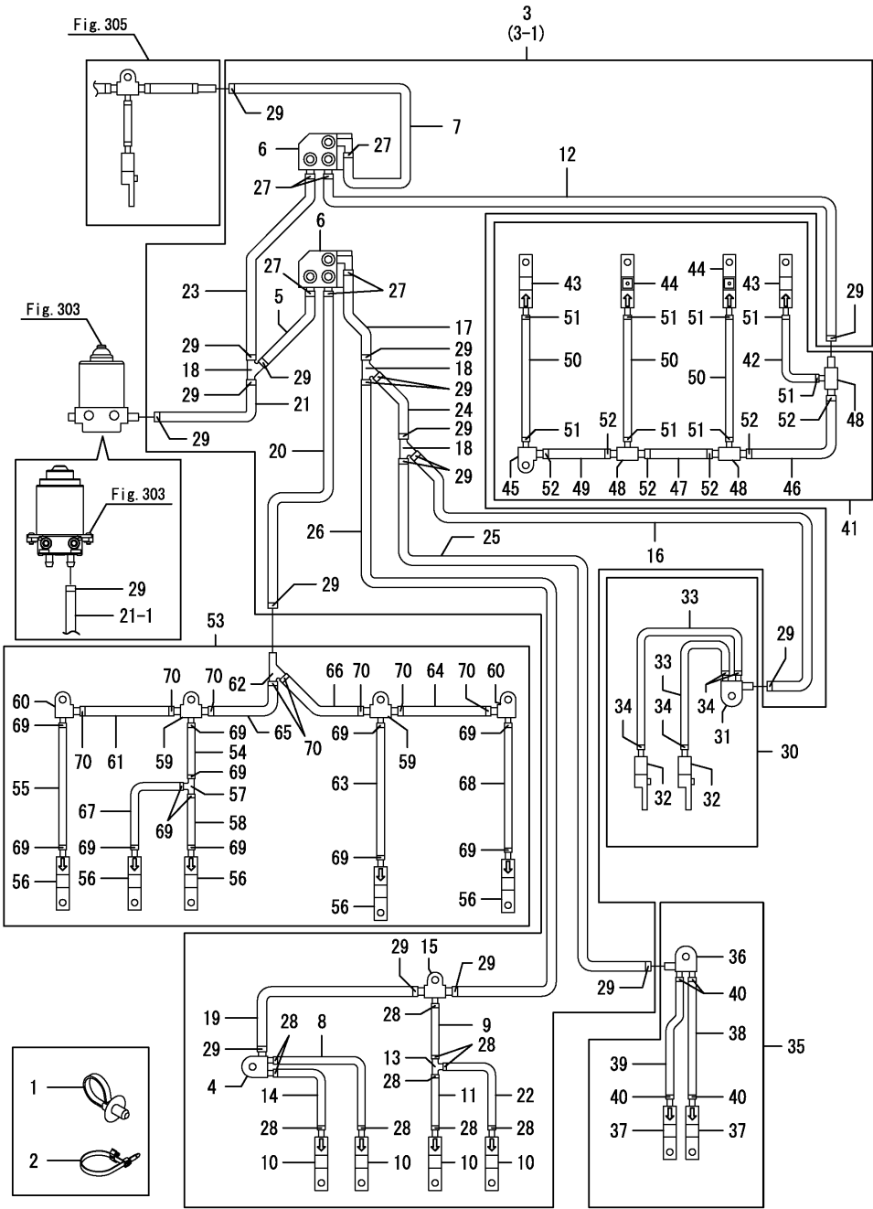
Fig.304. 주유장치(2)
