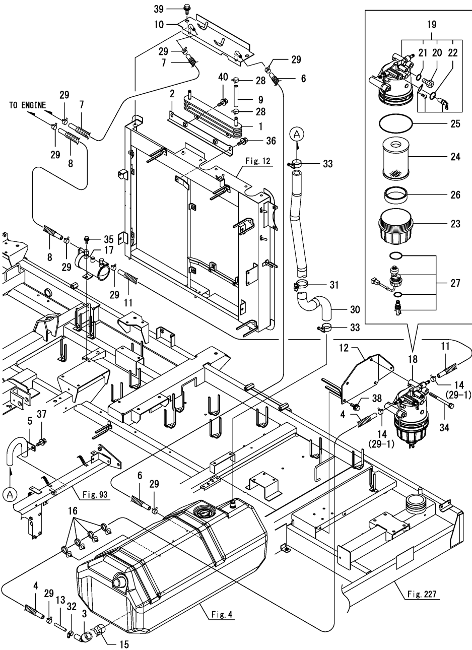
Fig.5. 연료탱크(2)
