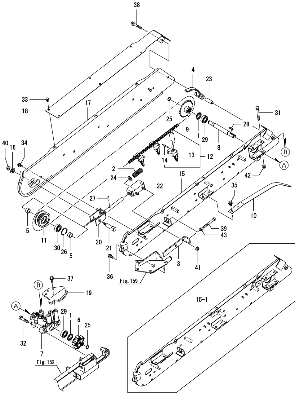
Fig.153. 쟁배출반송(이삭끝)
